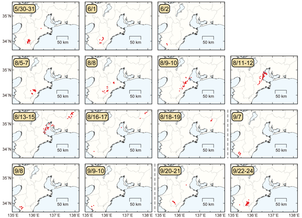
第 4 図 2024 年 5 月から 2024 年 10 月までの期間に東海・紀伊半島地域で発生した、主な深部低周波微動及び深部超低周波地震の活動における震央分布スナップショット。赤丸が当該期間の微動、青菱形が超低周波地震を表す。
