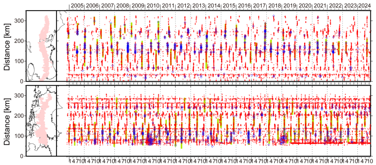
第 3 図 西南日本で発生した深部低周波微動（赤丸）及び深部超低周波地震（青菱形）の 2004 年 11 月から約 20 年間の時空間分布. 黄緑色太線は、傾斜変動から検出された短期的スロースリップイベントを示す.
