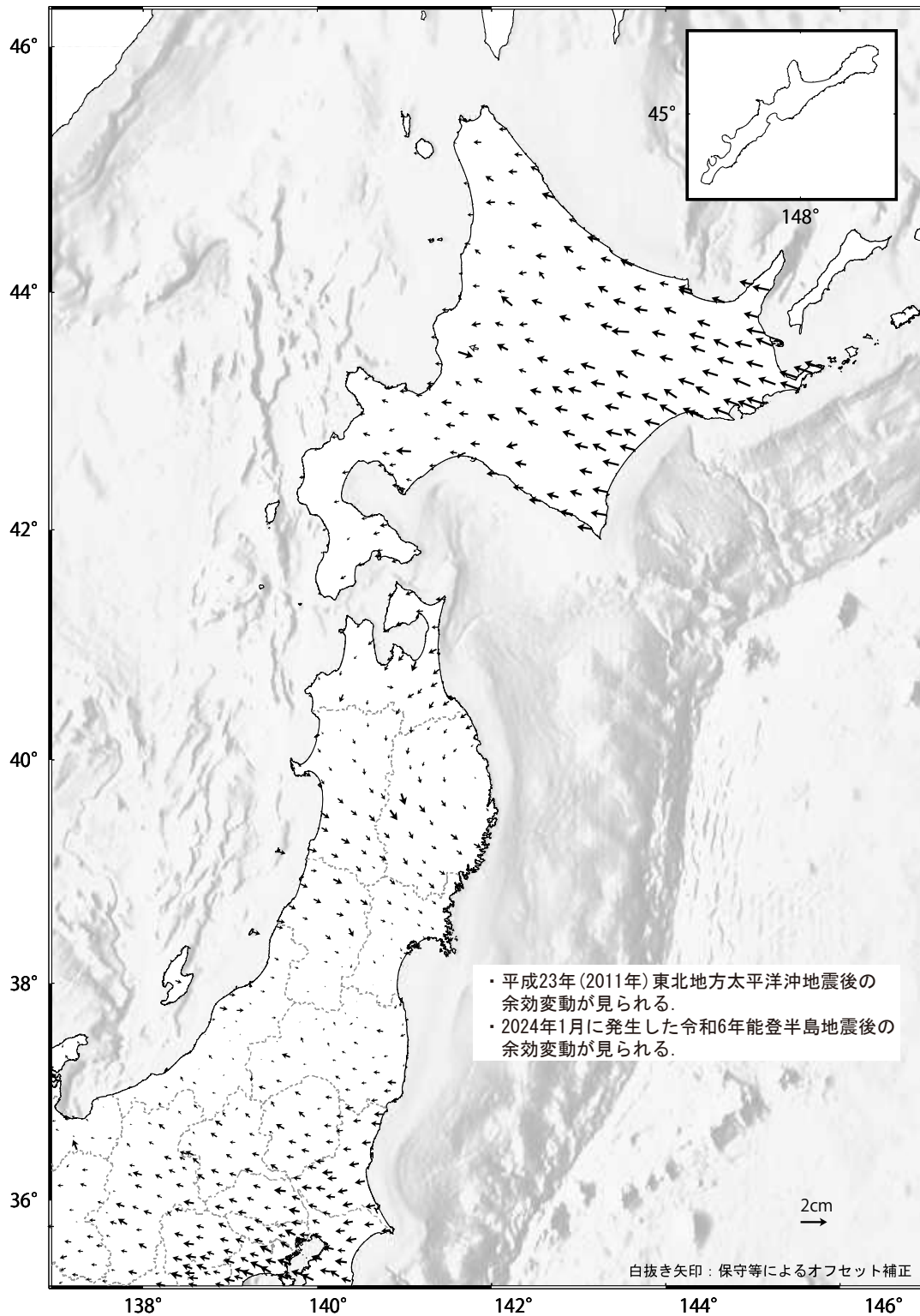
第 1 図 GNSS 連続観測データから求めた 2025 年 1 月～2025 年 4 月の水平変動
