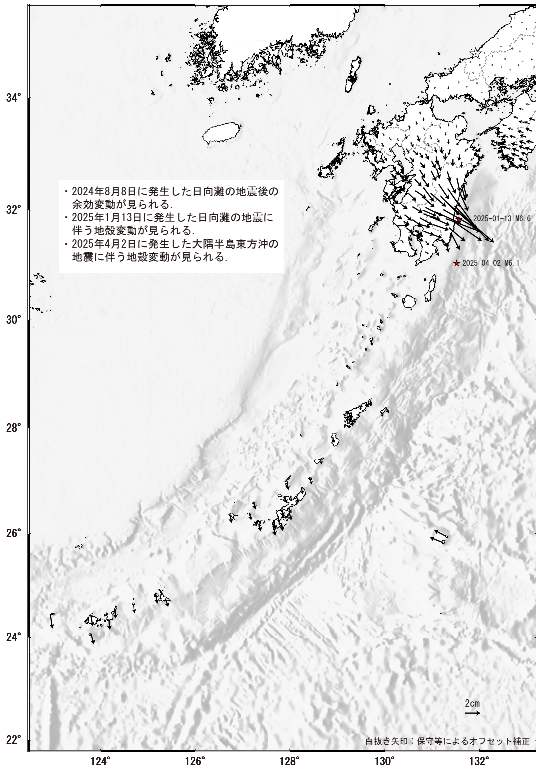
第 3 図 GNSS 連続観測データから求めた 2025 年 1 月～2025 年 4 月の水平変動（つづき）
