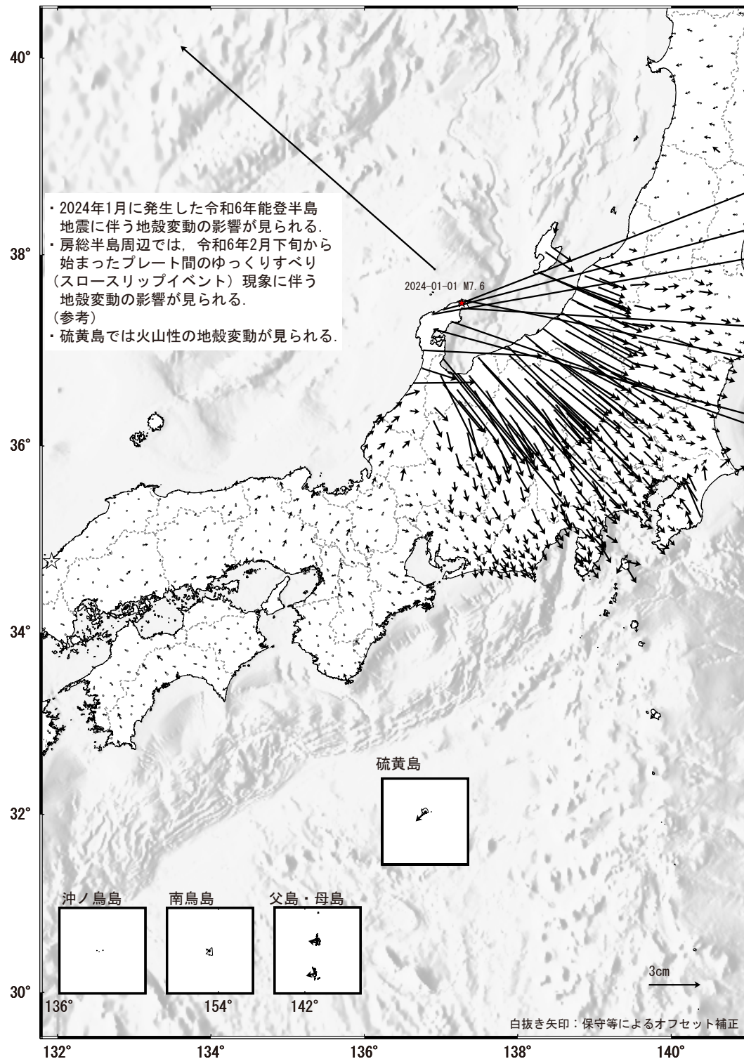
第 5 図 GNSS 連続観測データから求めた 2 期間の水平変動の差 (つづき)
