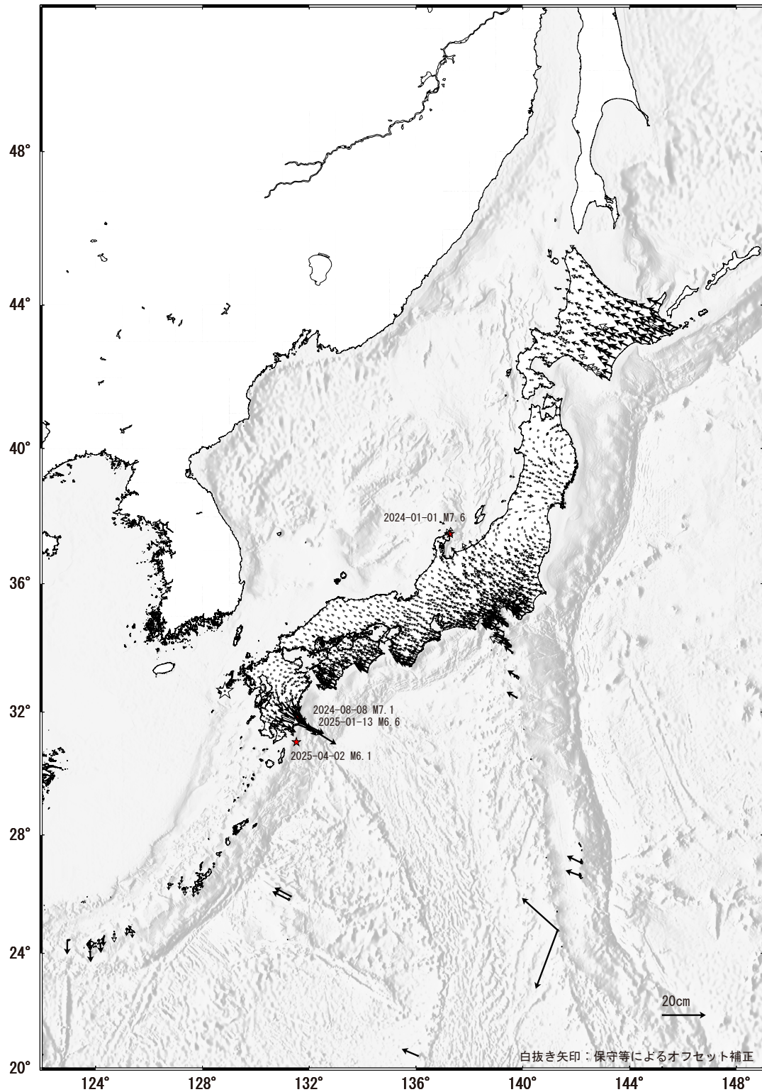
第 7 図 GNSS 連続観測データから求めた 2024 年 4 月～2025 年 4 月の水平変動
