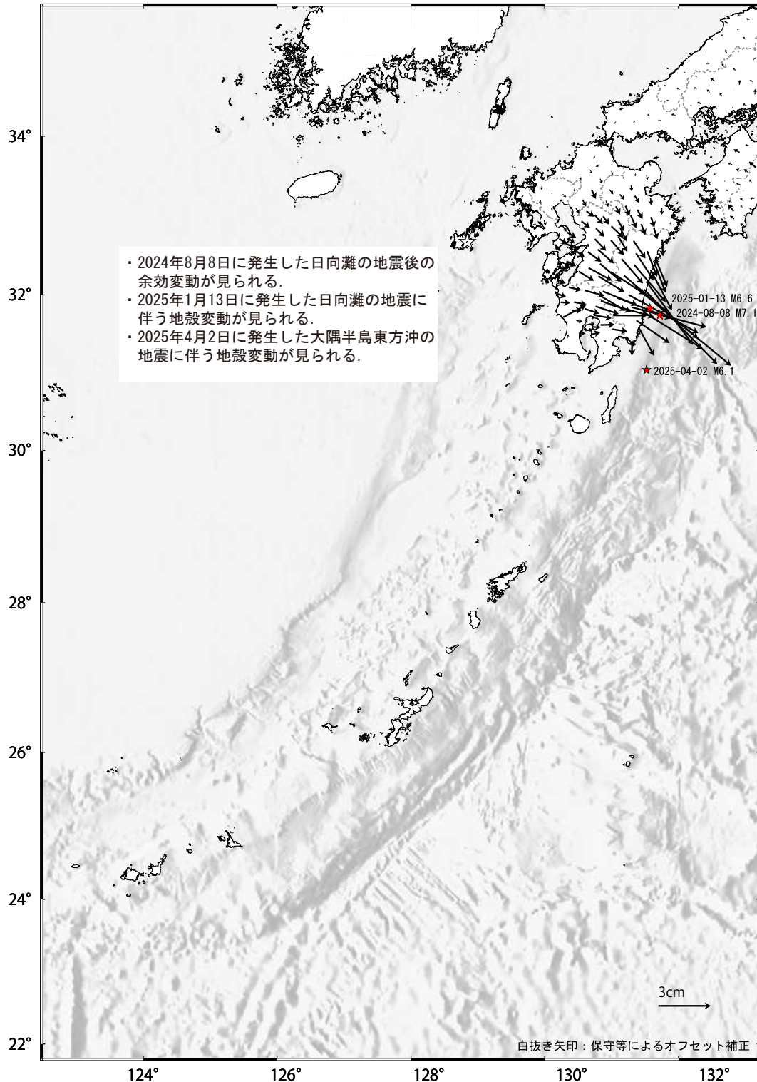
第 6 図 GNSS 連続観測データから求めた 2 期間の水平変動の差 (つづき)
