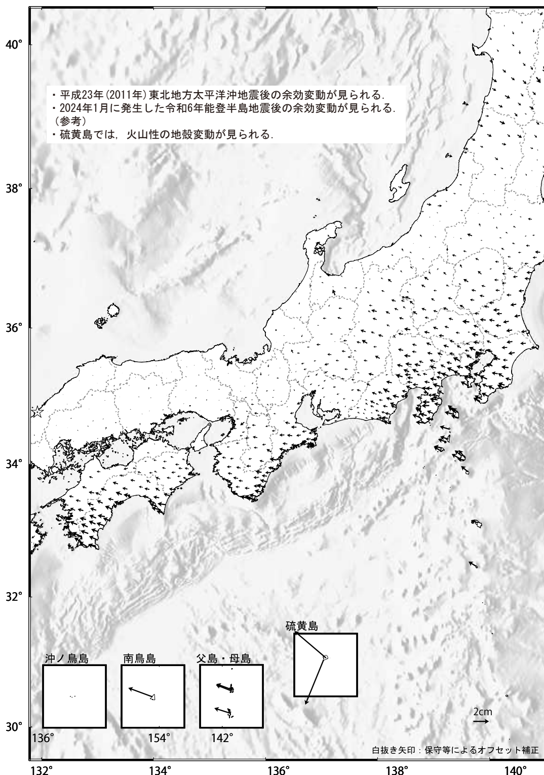
第 2 図 GNSS 連続観測データから求めた 2025 年 1 月～2025 年 4 月の水平変動（つづき）
