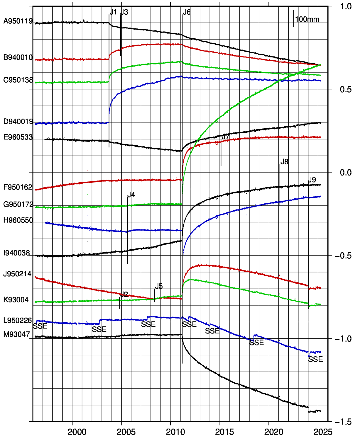
第 2a 図 プレート沈み込み方向の位置変化（東日本；1996 年から 2025 年 4 月） 沈み込みと逆方向が上向き。地点番号は、第 1 図の観測点記号に GEONET 観測点番号を付加したもの。 J1:2003 年十勝沖地震 (M8.0), J2:2004 年新潟県中越地震 (M6.8), J3:2004 年 11 月 29 日釧路沖の地震 (M7.1), J4:2005 年 8 月 16 日宮城県沖の地震 (M7.2), J5:2008 年 5 月 8 日茨城県沖の地震 (M7.0), J6:2011 年東北地方太平洋沖地震 (M9.0), J7:2015 年 2 月 17 日三陸沖の地震 (M6.9), J8:2021 年 2 月 13 日福島県沖の地震 (M7.3), J9: 2024 年能登半島地震 (M7.6)。
