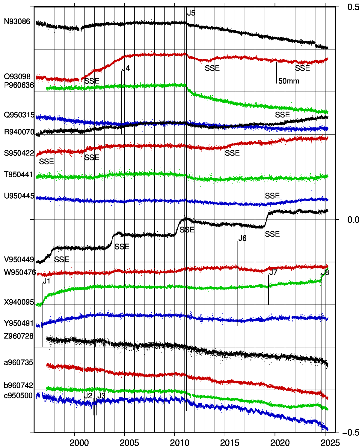
第 2b 図 プレート沈み込み方向の位置変化（西日本；1996 年から 2025 年 4 月） 沈み込みと逆方向が上向き。地点番号は、第 1 図の観測点記号に GEONET 観測点番号を付加したもの。 J1:1996 年 10 月 19 日日向灘の地震 (M6.9), J2:2001 年 12 月 18 日与那国島近海 (M7.3), J3:2002 年 3 月 31 日台湾付近の地震 (M7.2), J4:2004 年 9 月 5 日三重県南東沖の地震 (M7.4), J5:2011 年東北地方太平 洋沖地震 (M9.0), J6:2016 年熊本地震 (M7.3), J7:2019 年 5 月 10 日日向灘の地震 (M6.3), J8:2024 年 8 月 8 日日向灘の地震 (M7.1)。
