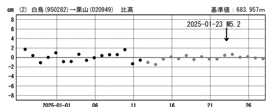
第 1 図 福島県会津の地震(2025 年 1 月 23 日, M5.2) 前後の観測データ(暫定): (上図) 基線図, (下図) 3 成分時系列グラフ
