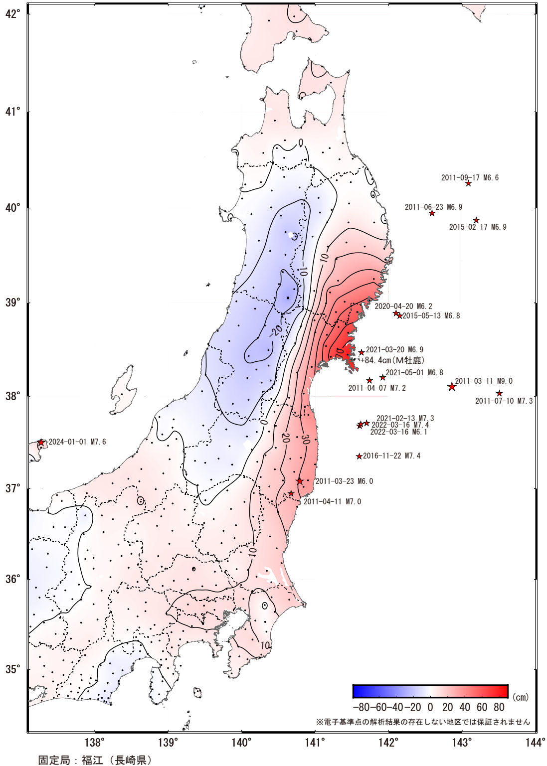
第 4 図 2011 年東北地方太平洋沖地震 (M9.0) 後の累積地殻変動 (上下、コンター)
