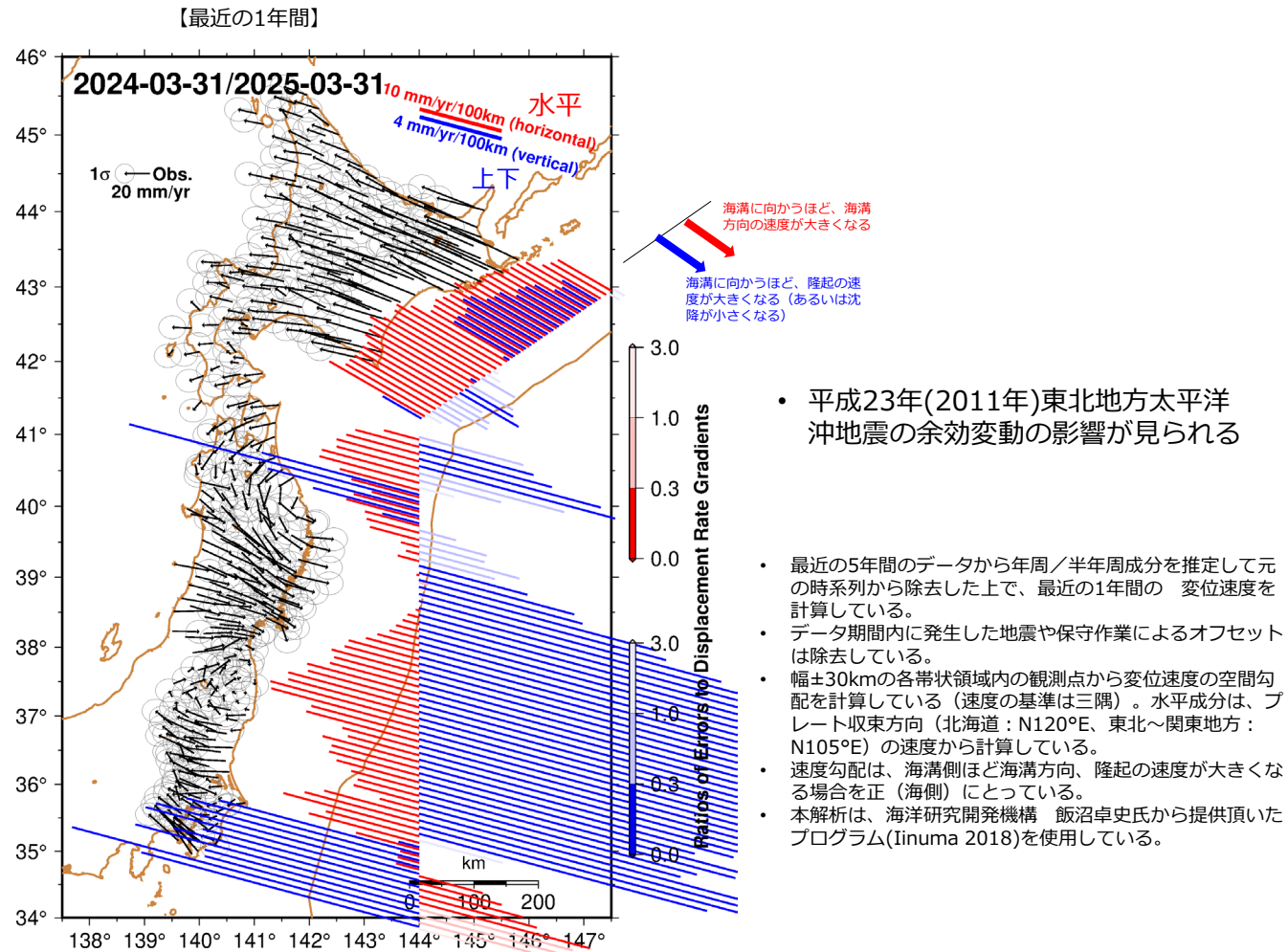
第 8 図 変位速度のプレート収束方向に関する水平勾配
