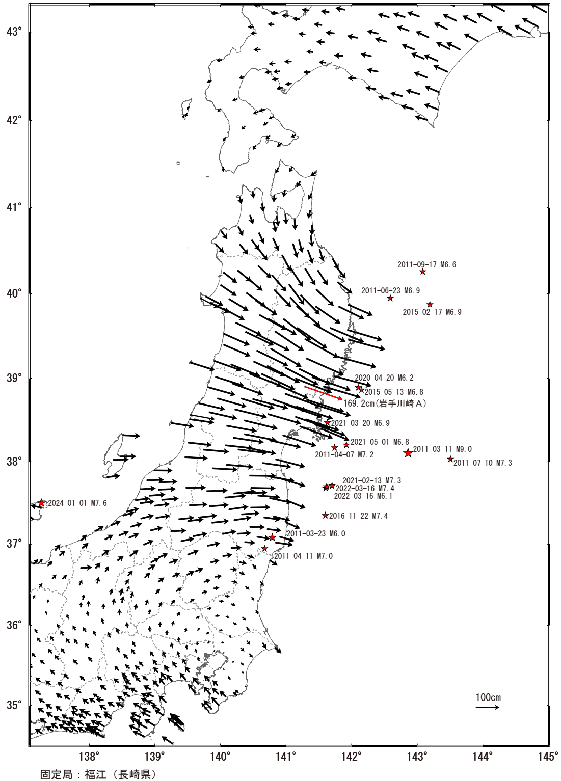
第 2 図 2011 年東北地方太平洋沖地震（M9.0）後の累積地殻変動（水平）
