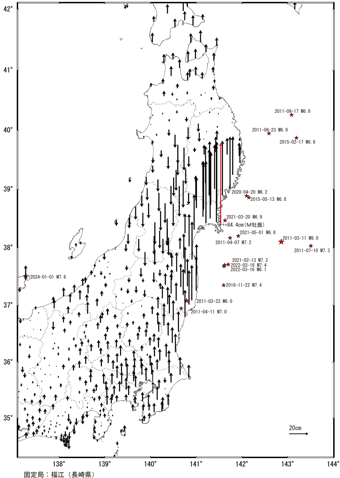
第 3 図 2011 年東北地方太平洋沖地震 (M9.0) 後の累積地殻変動 (上下)
