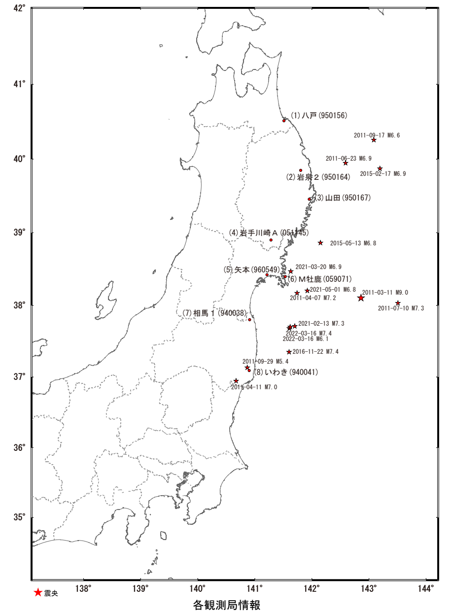
平成23年（2011年）東北地方太平洋沖地震後の地殻変動（時系列） 配点図
