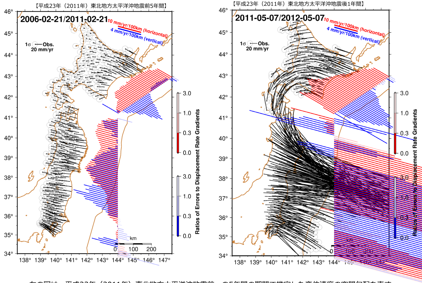
第 10 図 変位速度のプレート収束方向に関する水平勾配（比較用）
