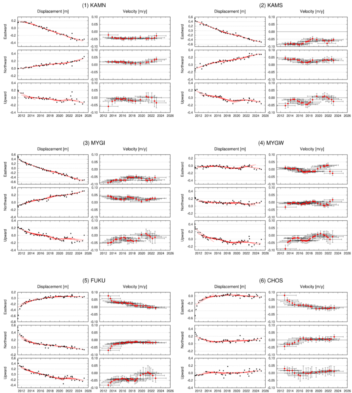
第 3 図 GNSS-A 観測時系列【北米プレート固定】
