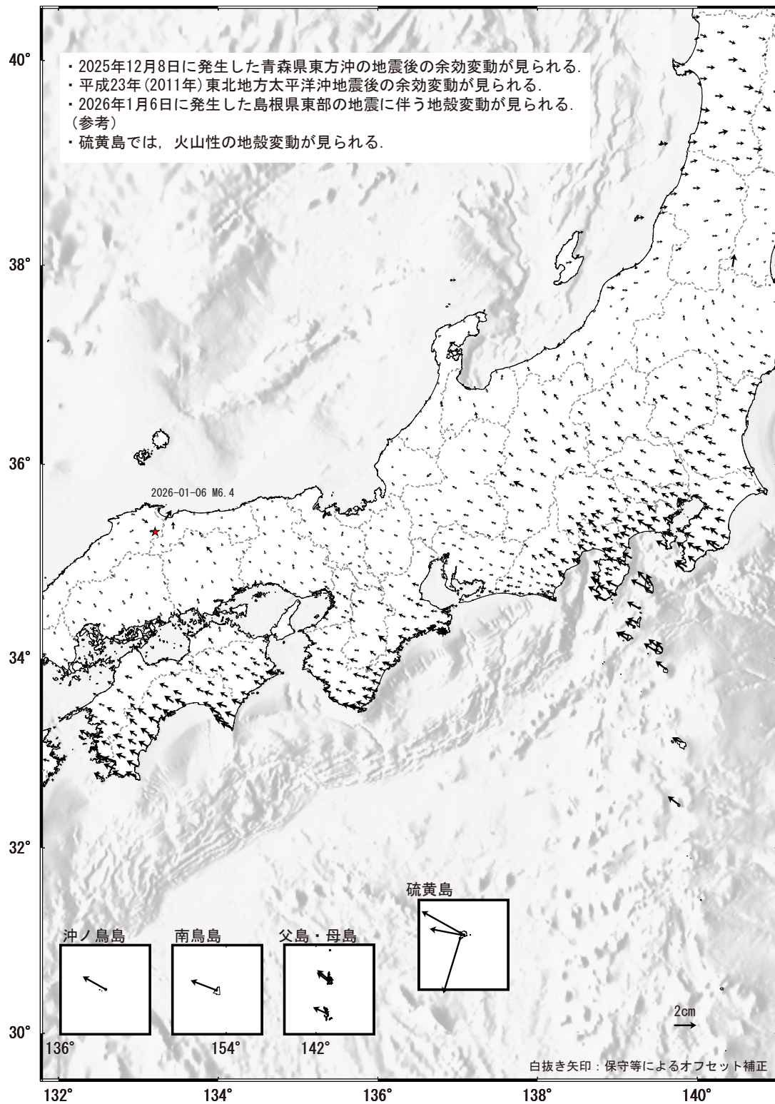
第 2 図 GNSS 連続観測データから求めた 2026 年 1 月～2026 年 4 月の水平変動（つづき）
