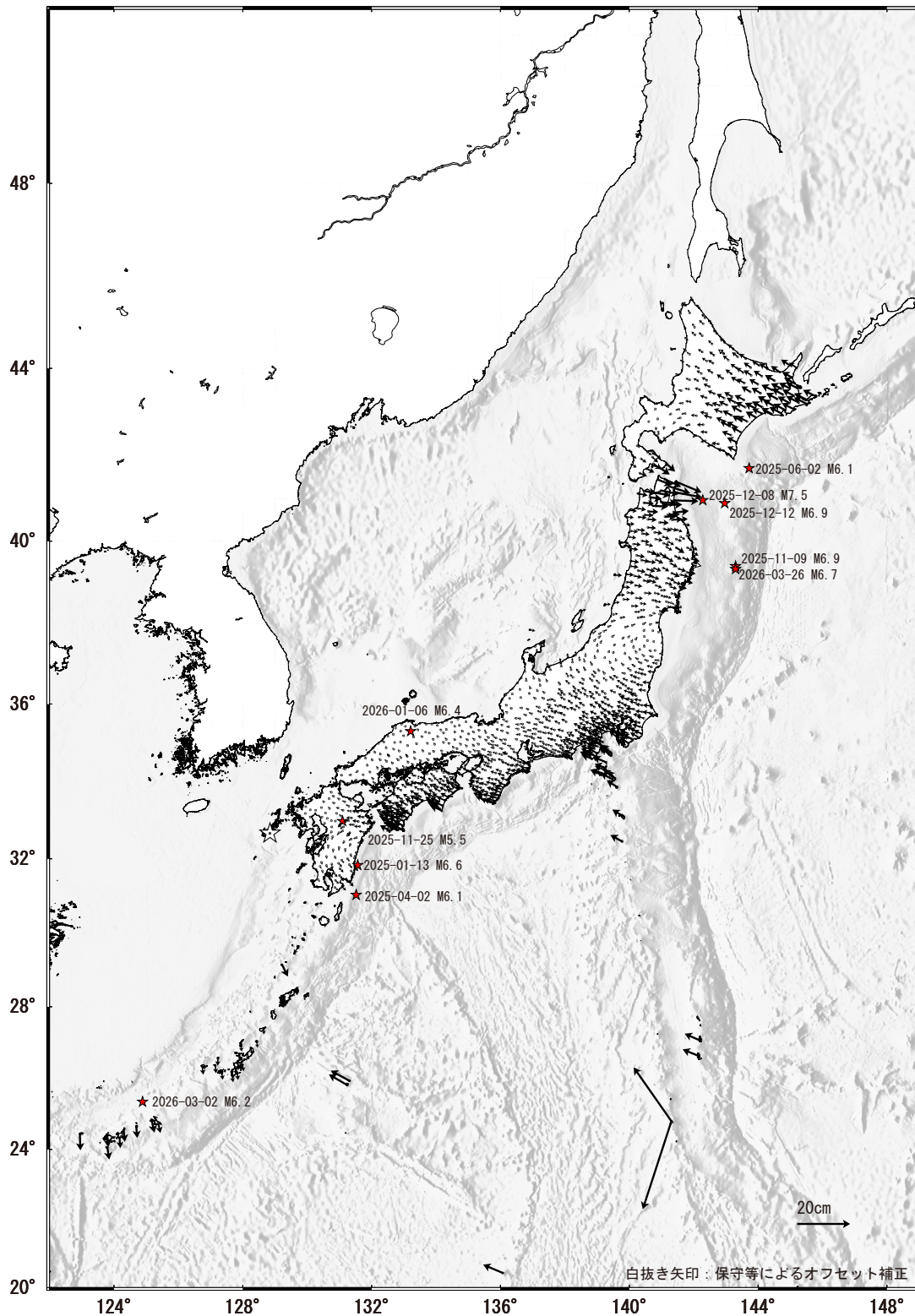
第 7 図 GNSS 連続観測データから求めた 2025 年 4 月～2026 年 4 月の水平変動
