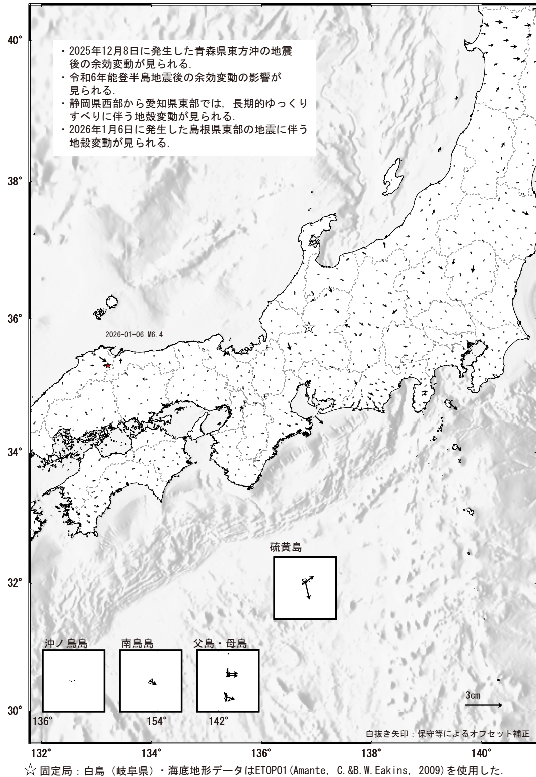
第 5 図 GNSS 連続観測データから求めた 2 期間の水平変動の差 (3 か月間) (つづき)
