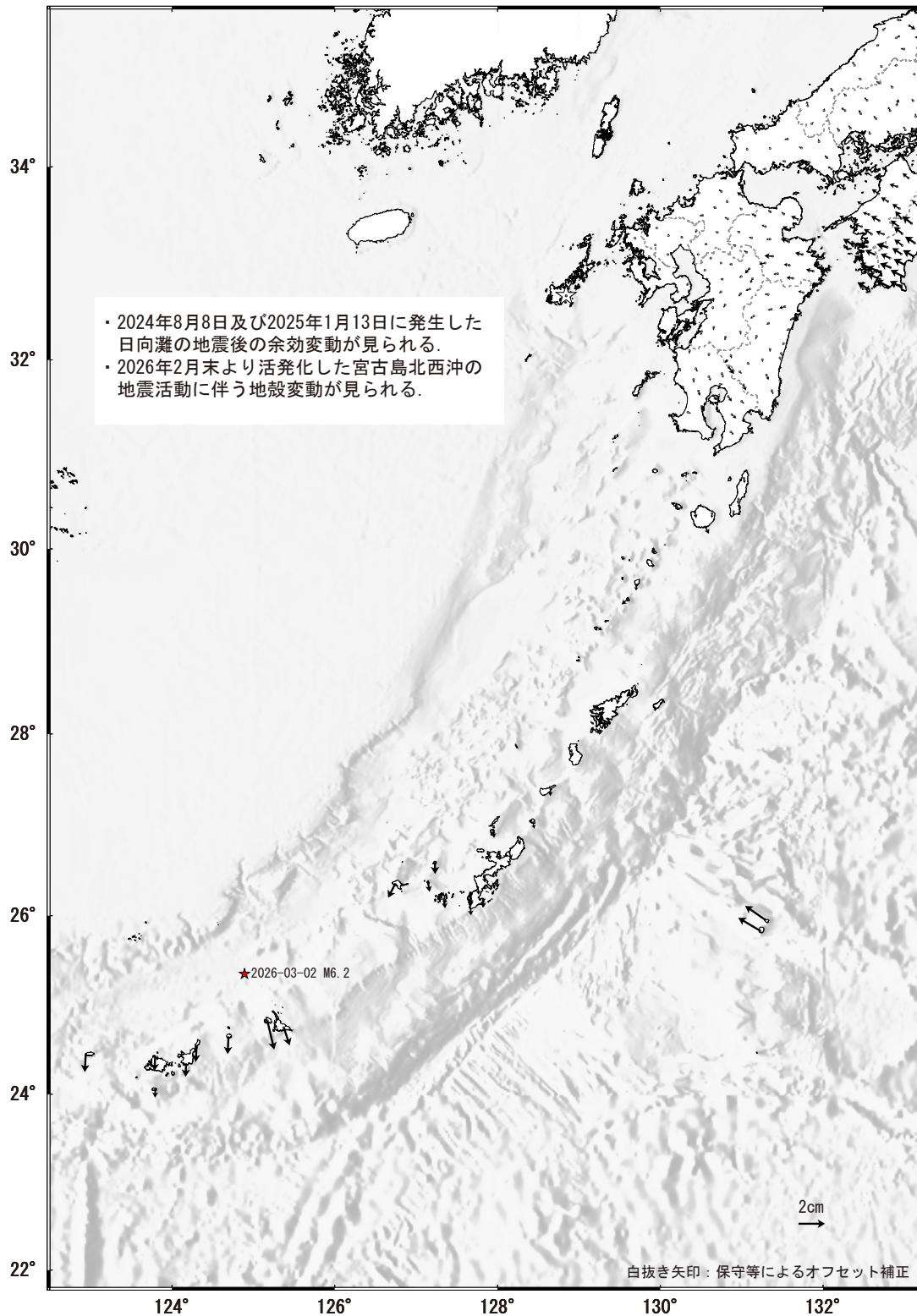
第 3 図 GNSS 連続観測データから求めた 2026 年 1 月～2026 年 4 月の水平変動（つづき）
