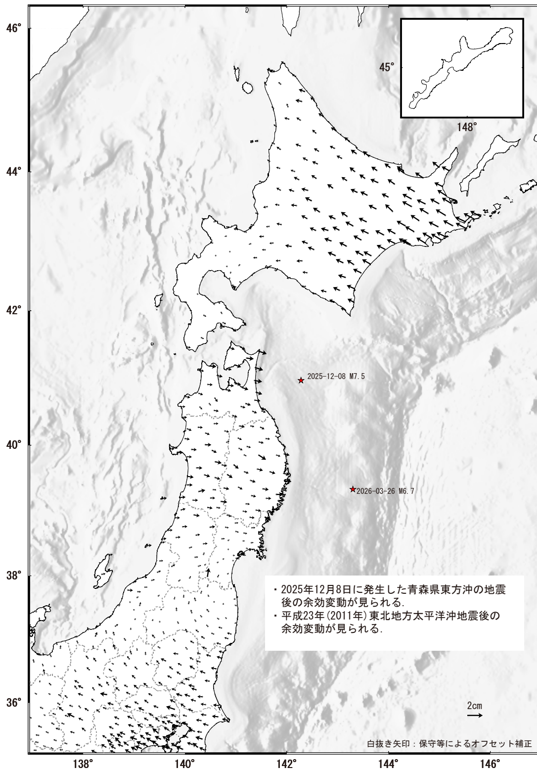
第 1 図 GNSS 連続観測データから求めた 2026 年 1 月～2026 年 4 月の水平変動
