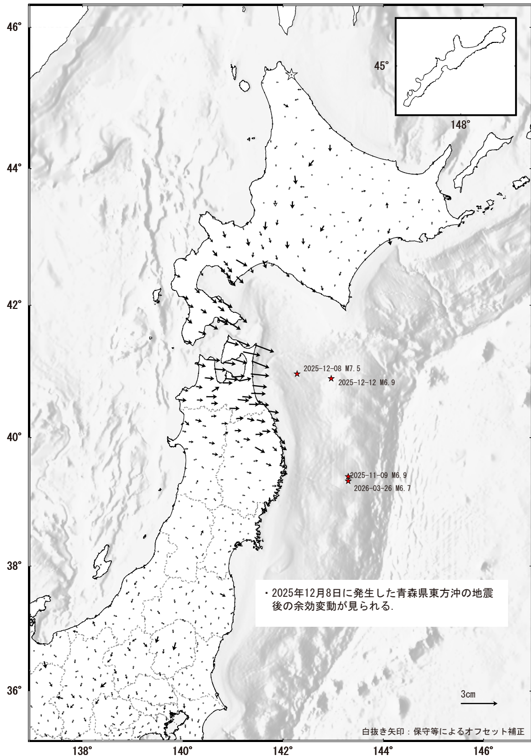
第 4 図 GNSS 連続観測データから求めた 2 期間の水平変動の差 (3 か月間)
