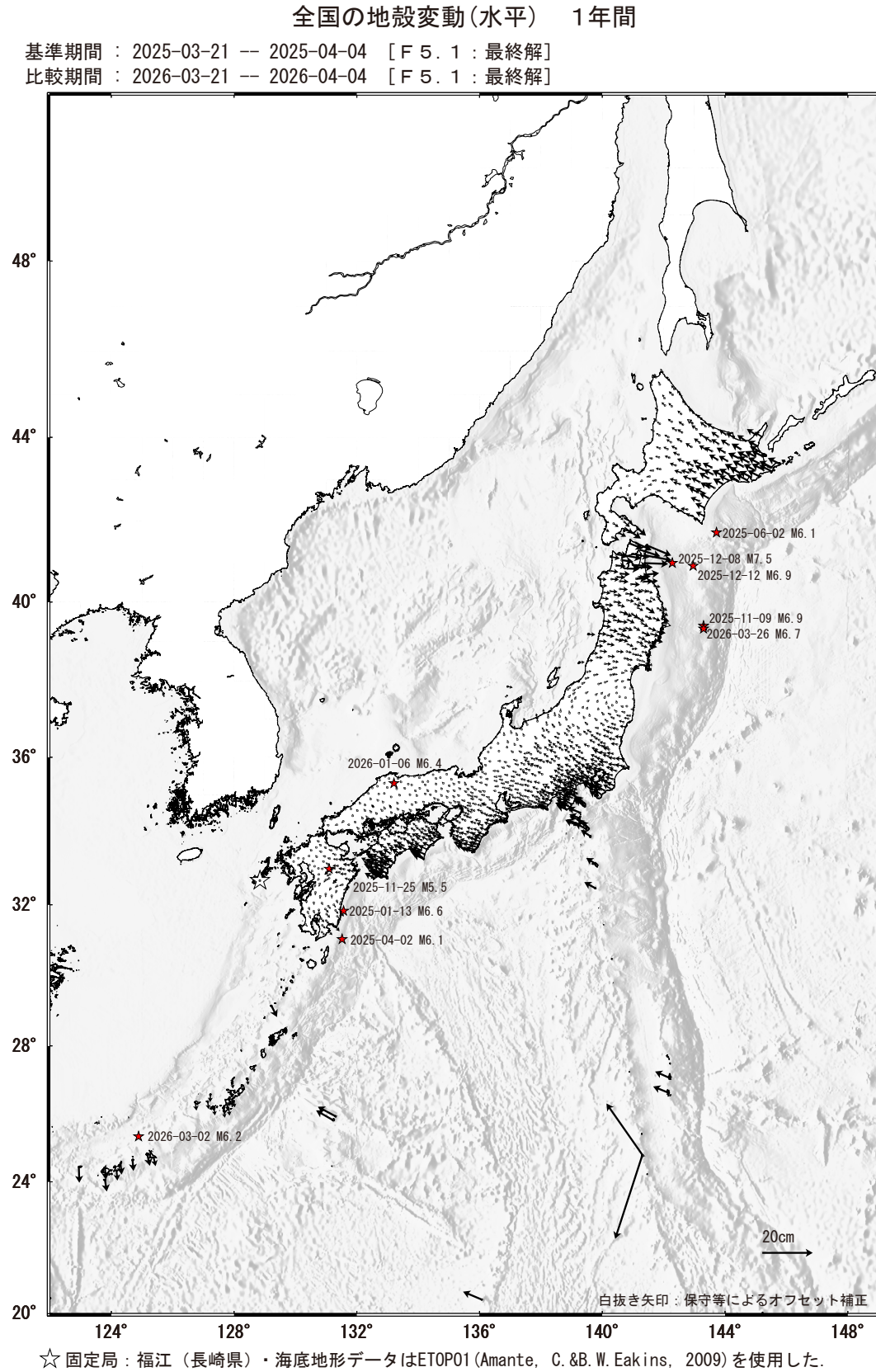
第 6 図 GNSS 連続観測データから求めた 2 期間の水平変動の差 (3 か月間) (つづき)
