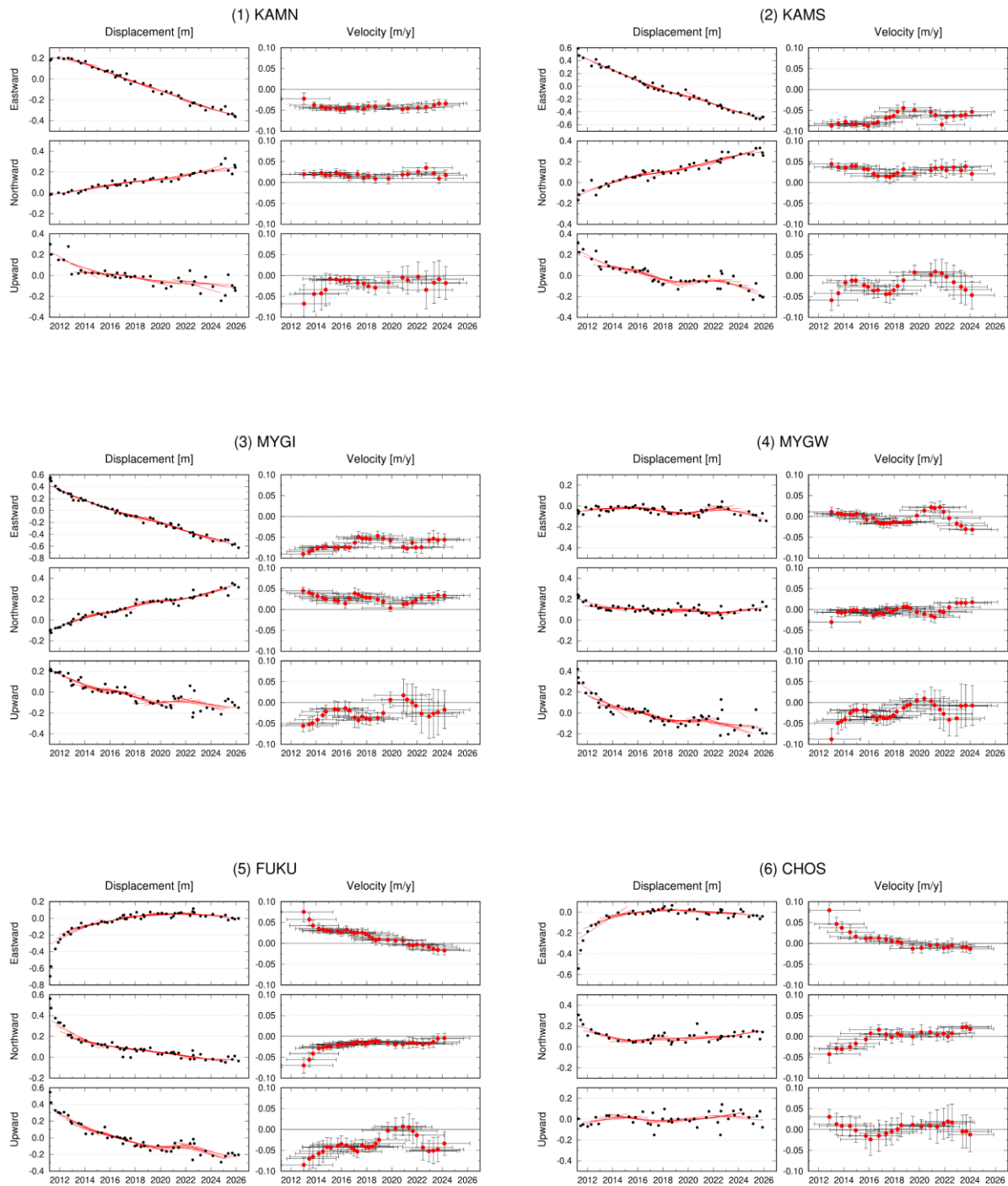
第 3 図 GNSS-A 観測時系列【北米プレート固定】
