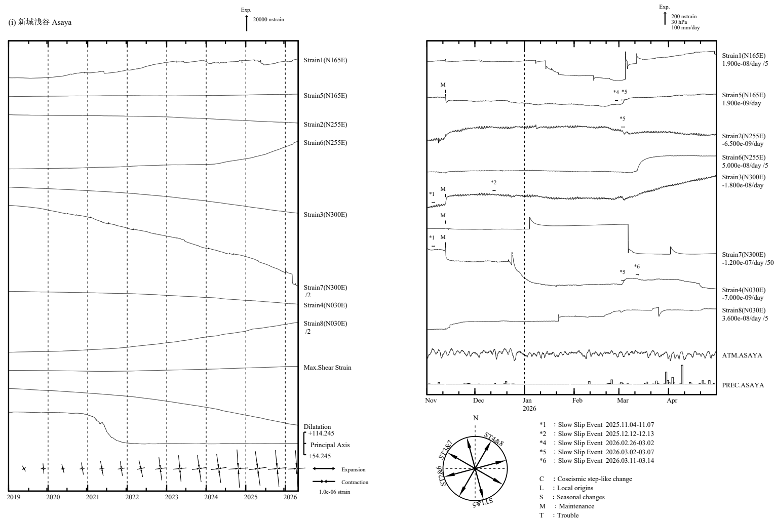
第4図(i) 左：2019年1月以後の多成分ひずみ計変化（日平均値）。主ひずみ・最大せん断ひずみ・面積ひずみは各方向成分から計算されている。 右：2025年11月～2026年4月の多成分ひずみ計変化（時間値：気圧・潮汐・地磁気・降水補正した値）。各図下部に気圧変化と降水量を示す。
