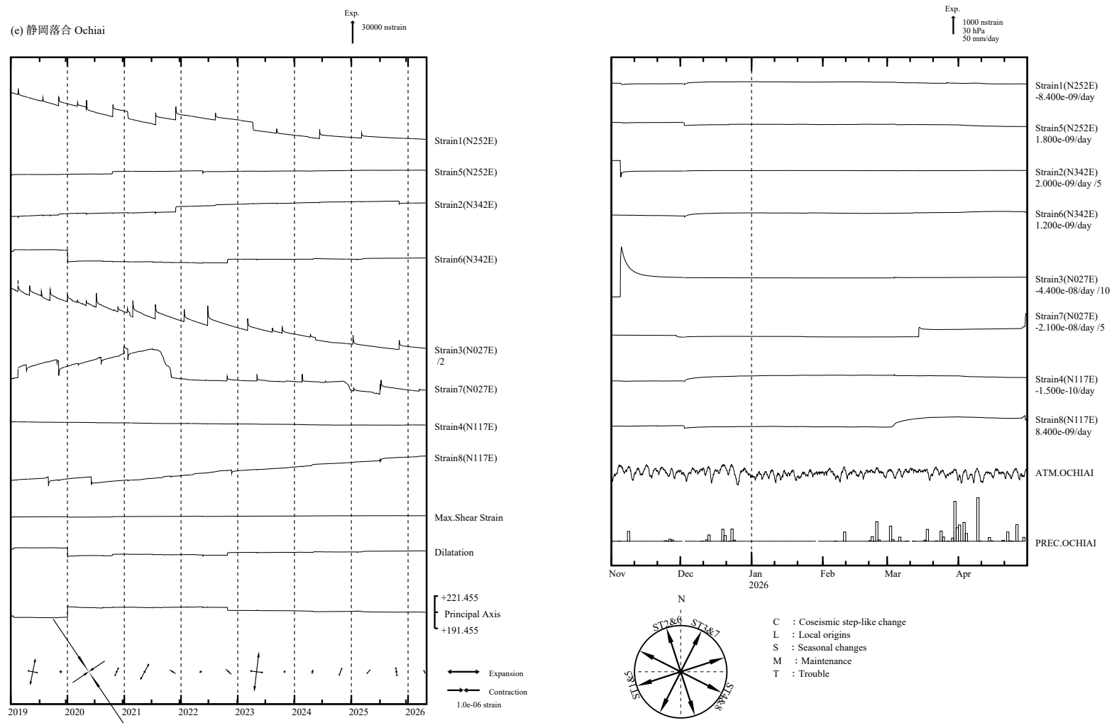
第 4 図 (e) 左：2019 年 1 月以後の多成分ひずみ計変化（日平均値）。主ひずみ・最大せん断ひずみ・面積ひずみは各方向成分から計算されている。 右：2025 年 11 月～2026 年 4 月の多成分ひずみ計変化（時間値：気圧・潮汐・地磁気・降水補正した値）。各図下部に気圧変化と降水量を示す。
