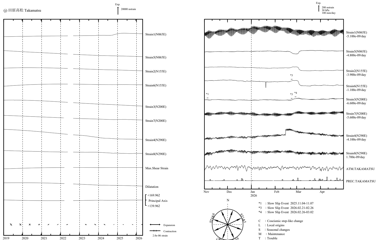
第 4 図 (j) 左：2019 年 1 月以後の多成分ひずみ計変化（日平均値）。主ひずみ・最大せん断ひずみ・面積ひずみは各方向成分から計算されている。 右：2025 年 11 月～2026 年 4 月の多成分ひずみ計変化（時間値：気圧・潮汐・地磁気・降水補正した値）。各図下部に気圧変化と降水量を示す。
