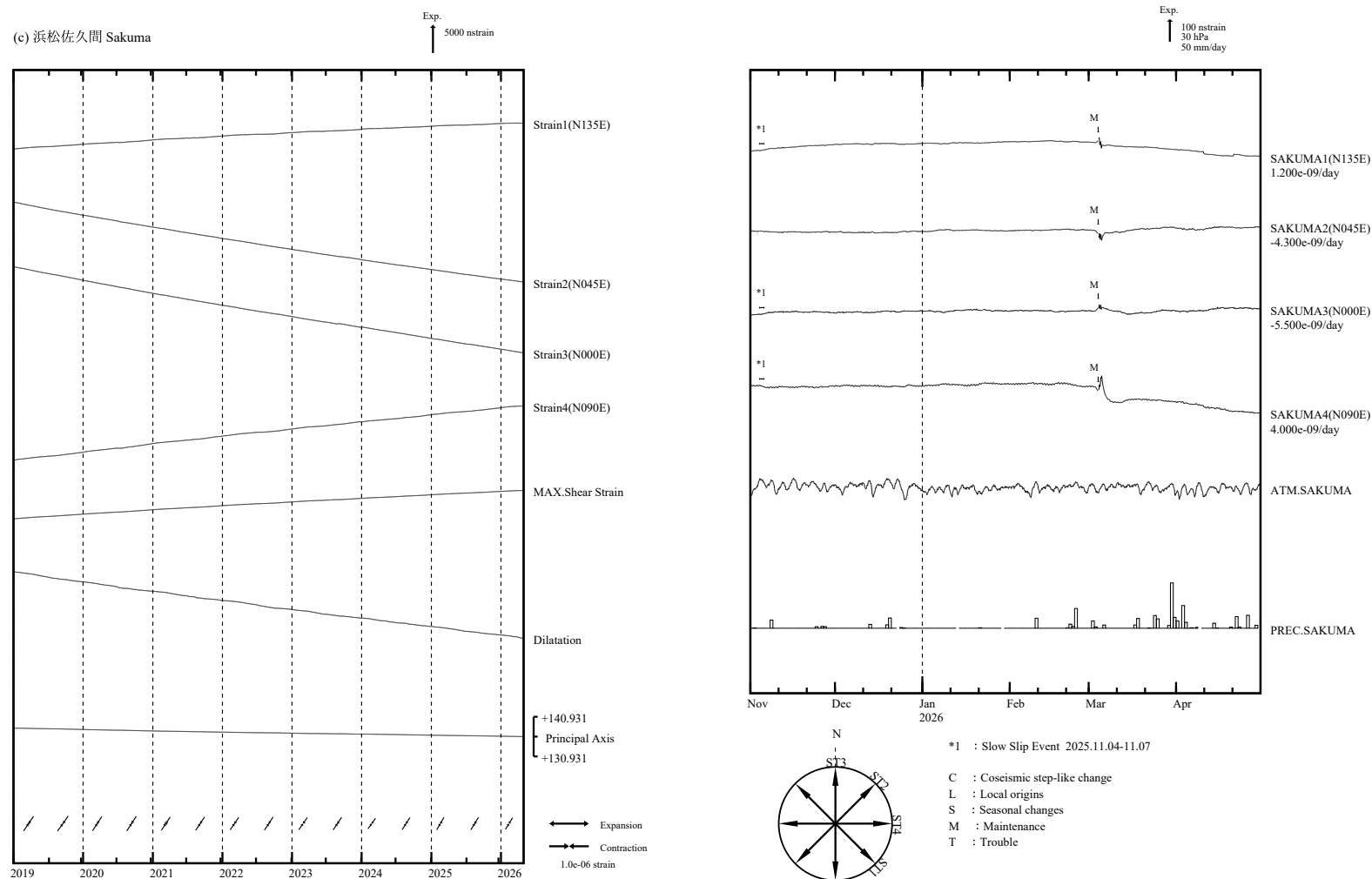
第 4 図 (c) 左 : 2019 年 1 月以後の多成分ひずみ計変化 (日平均値)。主ひずみ・最大せん断ひずみ・面積ひずみは各方向成分から計算されている。 右 : 2025 年 11 月～2026 年 4 月の多成分ひずみ計変化 (時間値 : 気圧・潮汐・地磁気・降水補正した値)。各図下部に気圧変化と降水量を示す。
