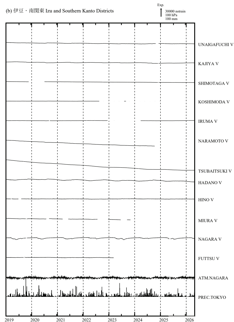
第 2 図 (a),(b) 2019 年 1 月以後の東海・伊豆・南関東地域における区域別体積ひずみ (V) 及び面積ひずみ (S) の変化 (日平均値)。各図下部に区域を代表する気圧変化と降水量を示す。
