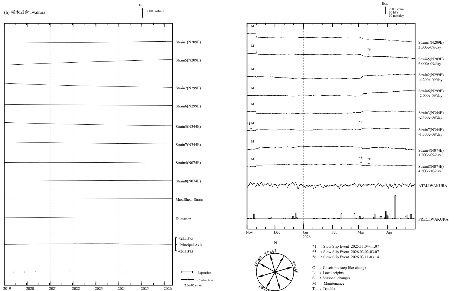
第 4 図 (h) 左 : 2019 年 1 月以後の多成分ひずみ計変化 (日平均値)。主ひずみ・最大せん断ひずみ・面積ひずみは各方向成分から計算されている。 右 : 2025 年 11 月～2026 年 4 月の多成分ひずみ計変化 (時間値 : 気圧・潮汐・地磁気・降水補正した値)。各図下部に気圧変化と降水量を示す。
