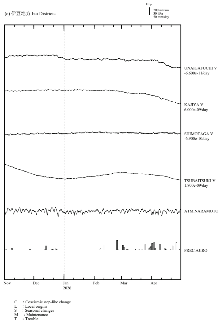
第 3 図 (c),(d) 2025 年 11 月～2026 年 4 月の東海・伊豆・南関東地域における区域別体積ひずみ (V) 及び面積ひずみ (S) の変化 (時間値: 気圧・潮汐・降水補正した値)。各図下部に区域を代表する気圧変化と降水量を示す。地点名の下の D strain/day 及び /M はそれぞれ 1 日あたりのトレンド変化量を D として補正していること及び縮尺を 1/M 倍にして表示していることを示している。
