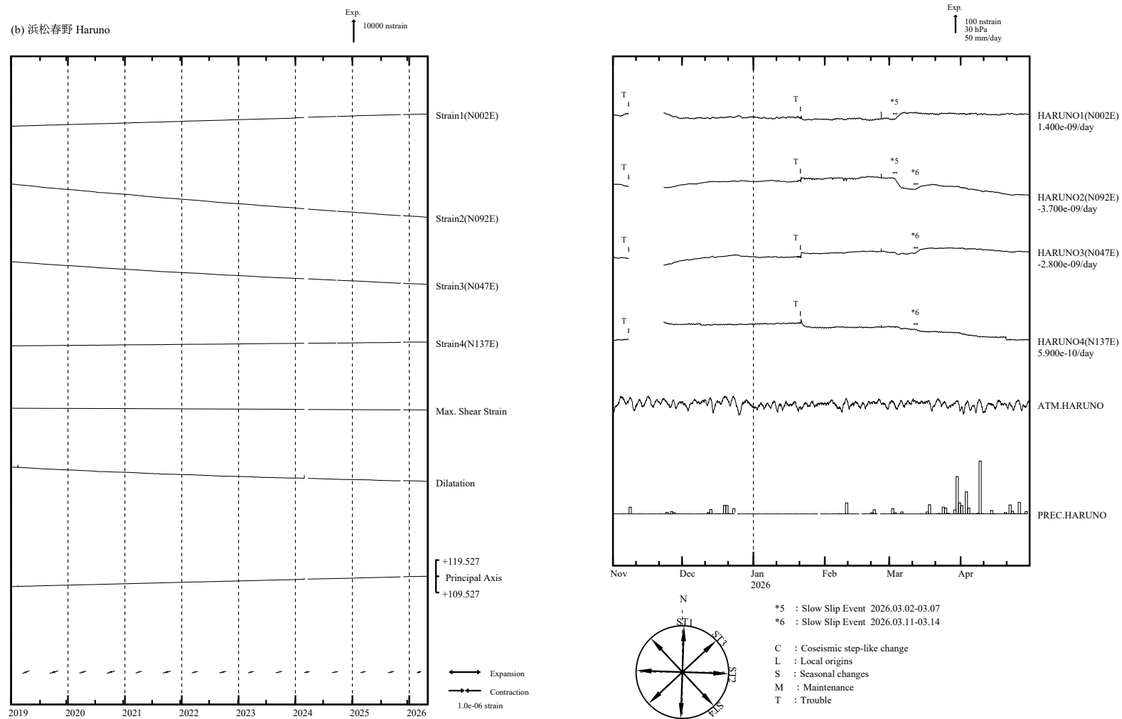
第 4 図 (b) 左：2019 年 1 月以後の多成分ひずみ計変化（日平均値）。主ひずみ・最大せん断ひずみ・面積ひずみは各方向成分から計算されている。 右：2025 年 11 月～2026 年 4 月の多成分ひずみ計変化（時間値：気圧・潮汐・地磁気・降水補正した値）。各図下部に気圧変化と降水量を示す。
