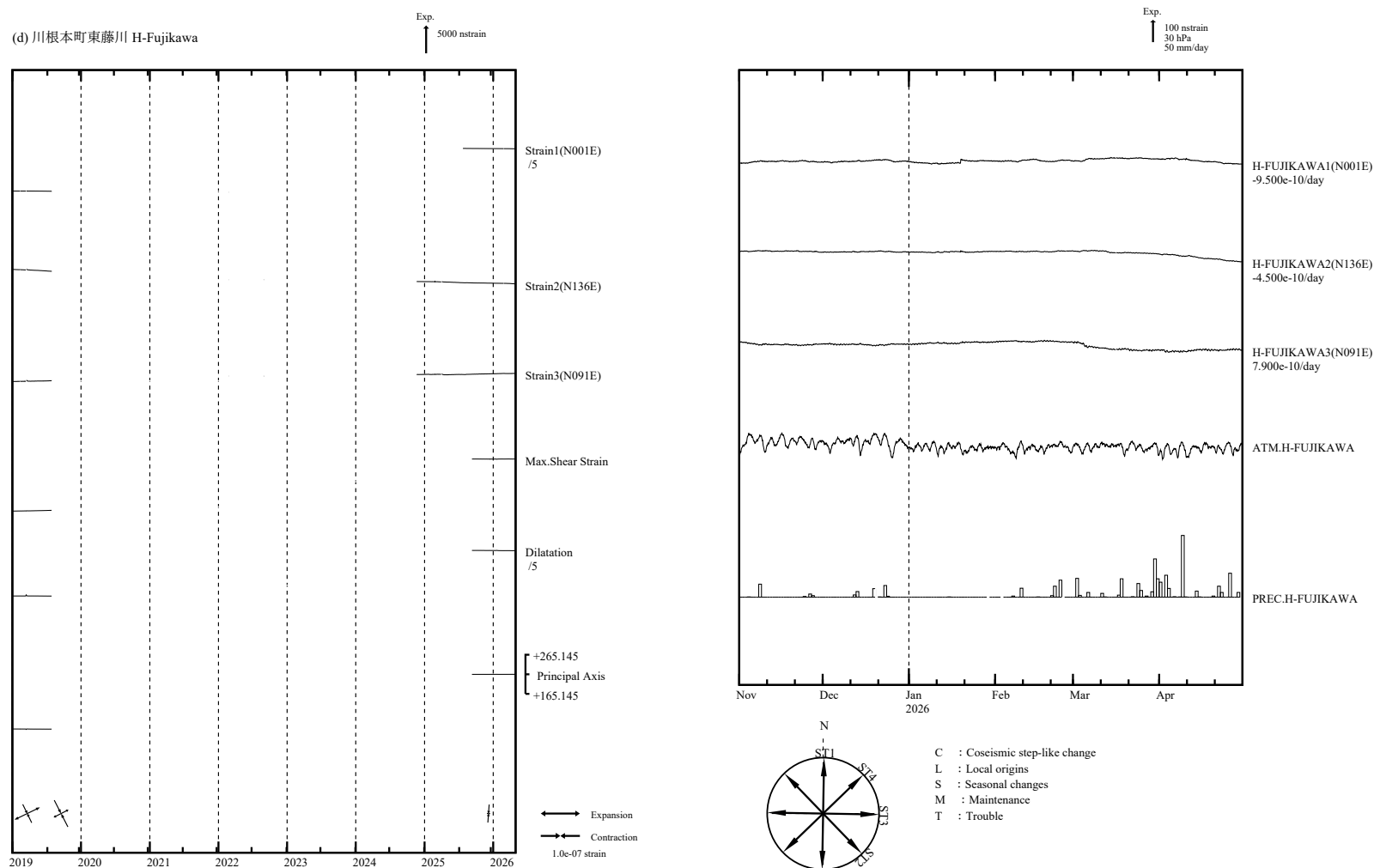
第 4 図 (d) 左：2019 年 1 月以後の多成分ひずみ計変化（日平均値）。主ひずみ・最大せん断ひずみ・面積ひずみは各方向成分から計算されている。 右：2025 年 11 月～2026 年 4 月の多成分ひずみ計変化（時間値：気圧・潮汐・地磁気・降水補正した値）。各図下部に気圧変化と降水量を示す。
