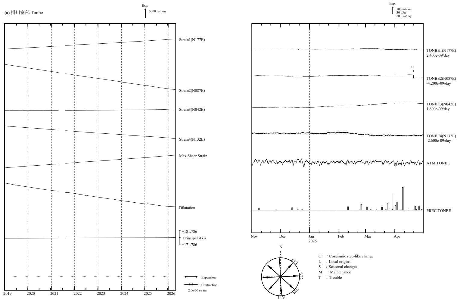
第 4 図 (a) 左 : 2019 年 1 月以後の多成分ひずみ計変化 (日平均値). 主ひずみ・最大せん断ひずみ・面積ひずみは各方向成分から計算されている. 右 : 2025 年 11 月～2026 年 4 月の多成分ひずみ計変化 (時間値 : 気圧・潮汐・地磁気・降水補正した値). 各図下部に気圧変化と降水量を示す.
