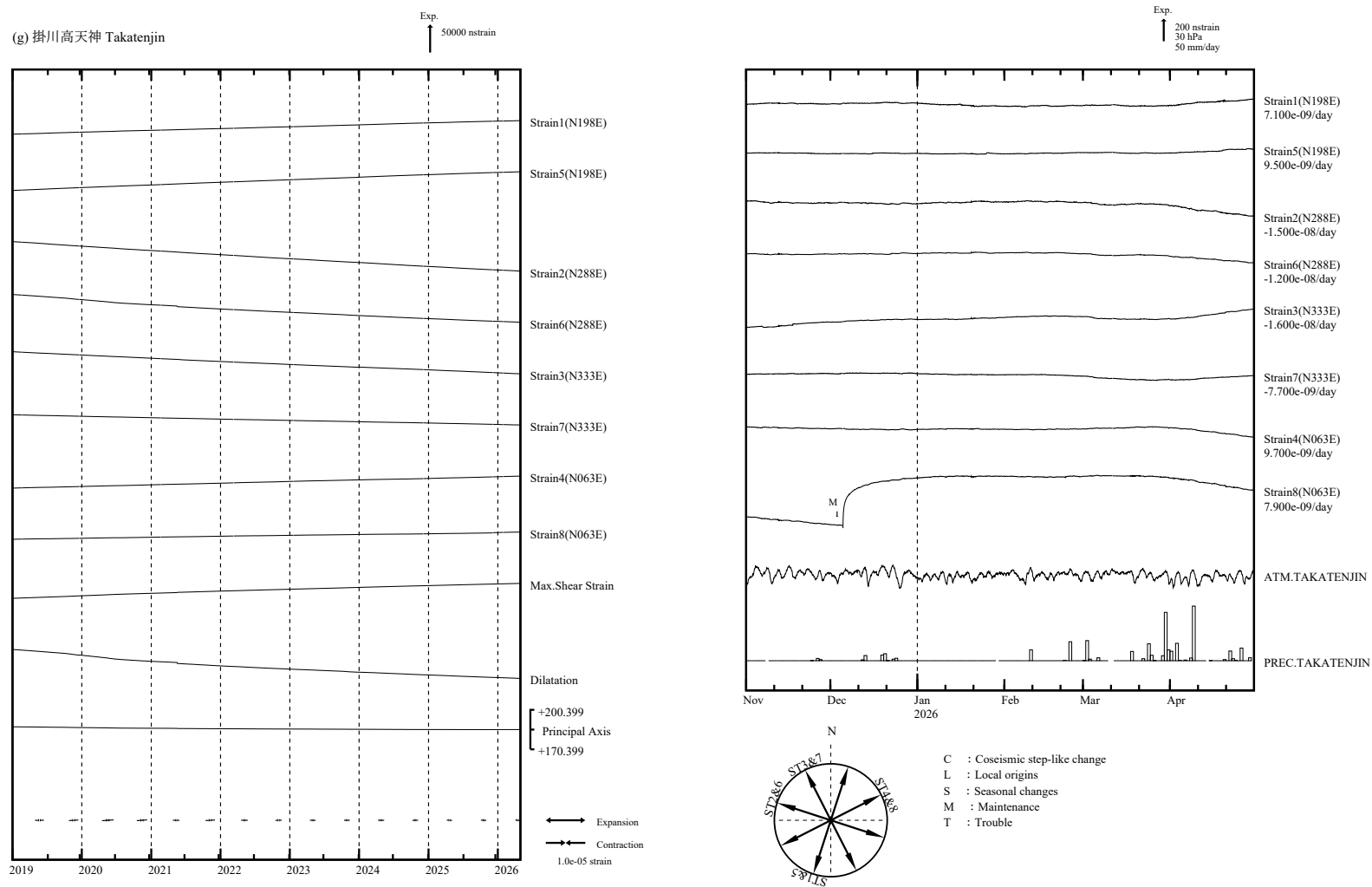
第 4 図 (g) 左：2019 年 1 月以後の多成分ひずみ計変化（日平均値）。主ひずみ・最大せん断ひずみ・面積ひずみは各方向成分から計算されている。 右：2025 年 11 月～2026 年 4 月の多成分ひずみ計変化（時間値：気圧・潮汐・地磁気・降水補正した値）。各図下部に気圧変化と降水量を示す。
