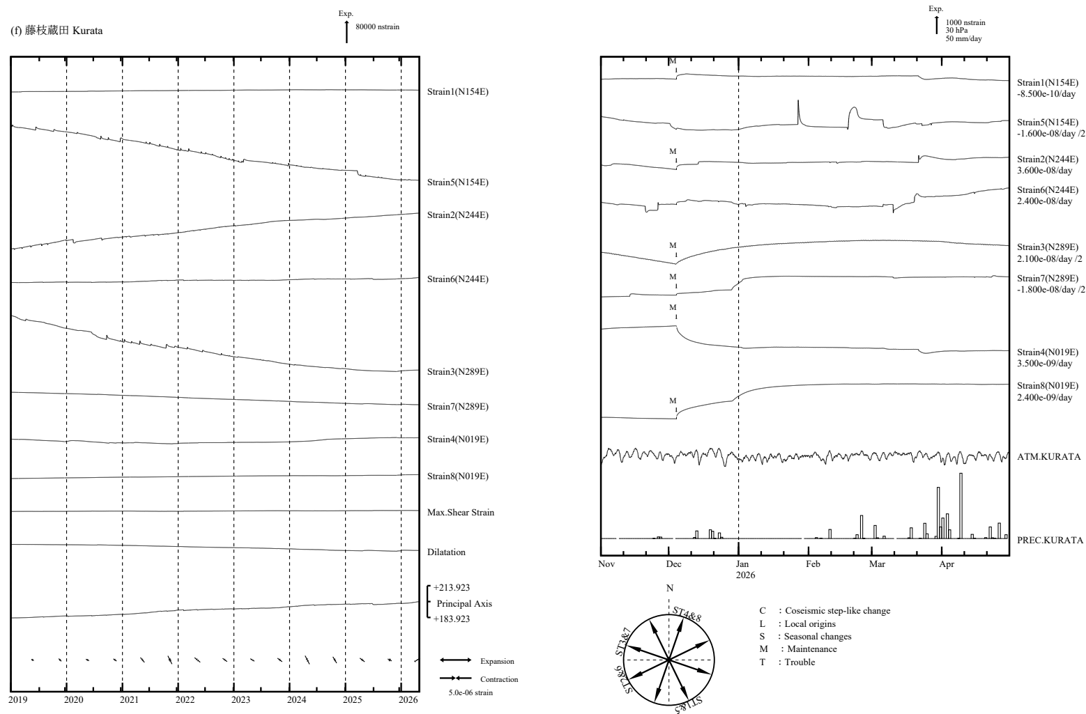
第 4 図 (f) 左 : 2019 年 1 月以後の多成分ひずみ計変化 (日平均値)。主ひずみ・最大せん断ひずみ・面積ひずみは各方向成分から計算されている。 右 : 2025 年 11 月～2026 年 4 月の多成分ひずみ計変化 (時間値 : 気圧・潮汐・地磁気・降水補正した値)。各図下部に気圧変化と降水量を示す。
