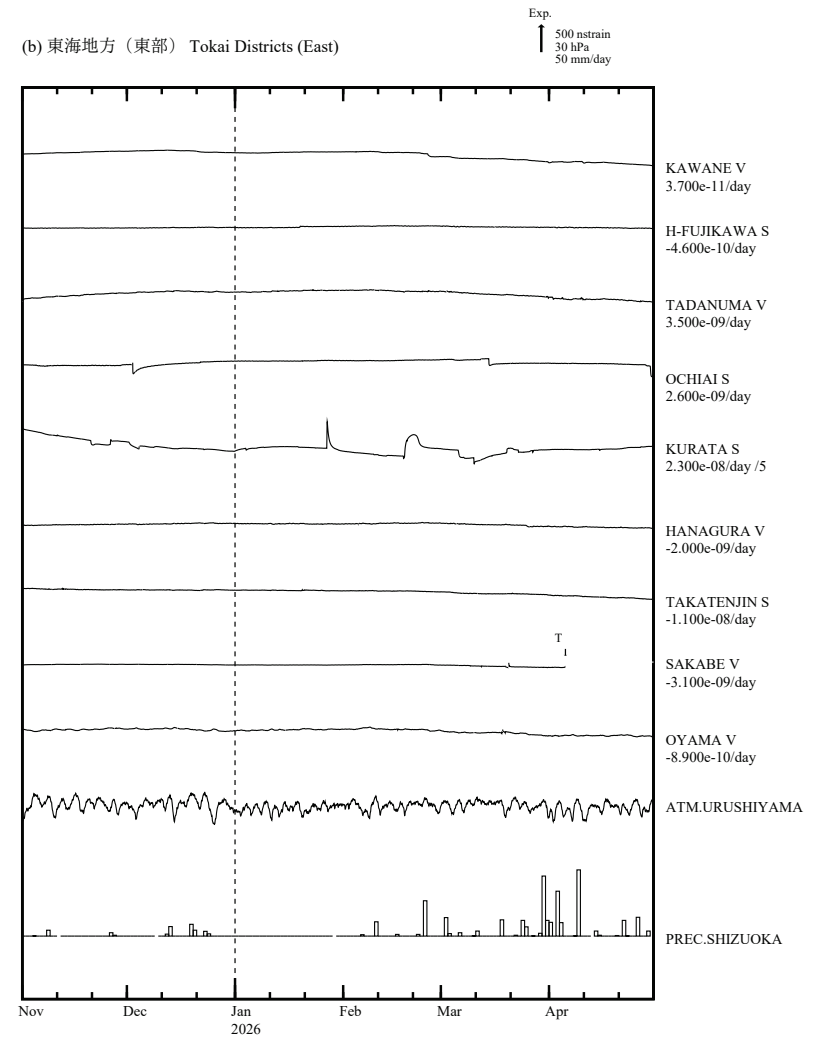
第 3 図 (a),(b) 2025 年 11 月～2026 年 4 月の東海・伊豆・南関東地域における区域別体積ひずみ (V) 及び面積ひずみ (S) の変化 (時間値: 気圧・潮汐・降水補正した値)。各図下部に区域を代表する気圧変化と降水量を示す。地点名の下の D strain/day 及び /M はそれぞれ 1 日あたりのトレンド変化量を D として補正していること及び縮尺を 1/M 倍にして表示していることを示している。
