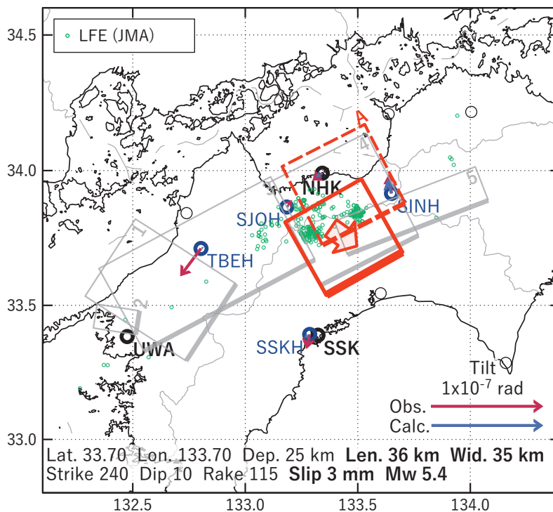
第 10 図 第 8 図 [B] を説明する断層モデル. 各図の説明は第 3 図を参照.
