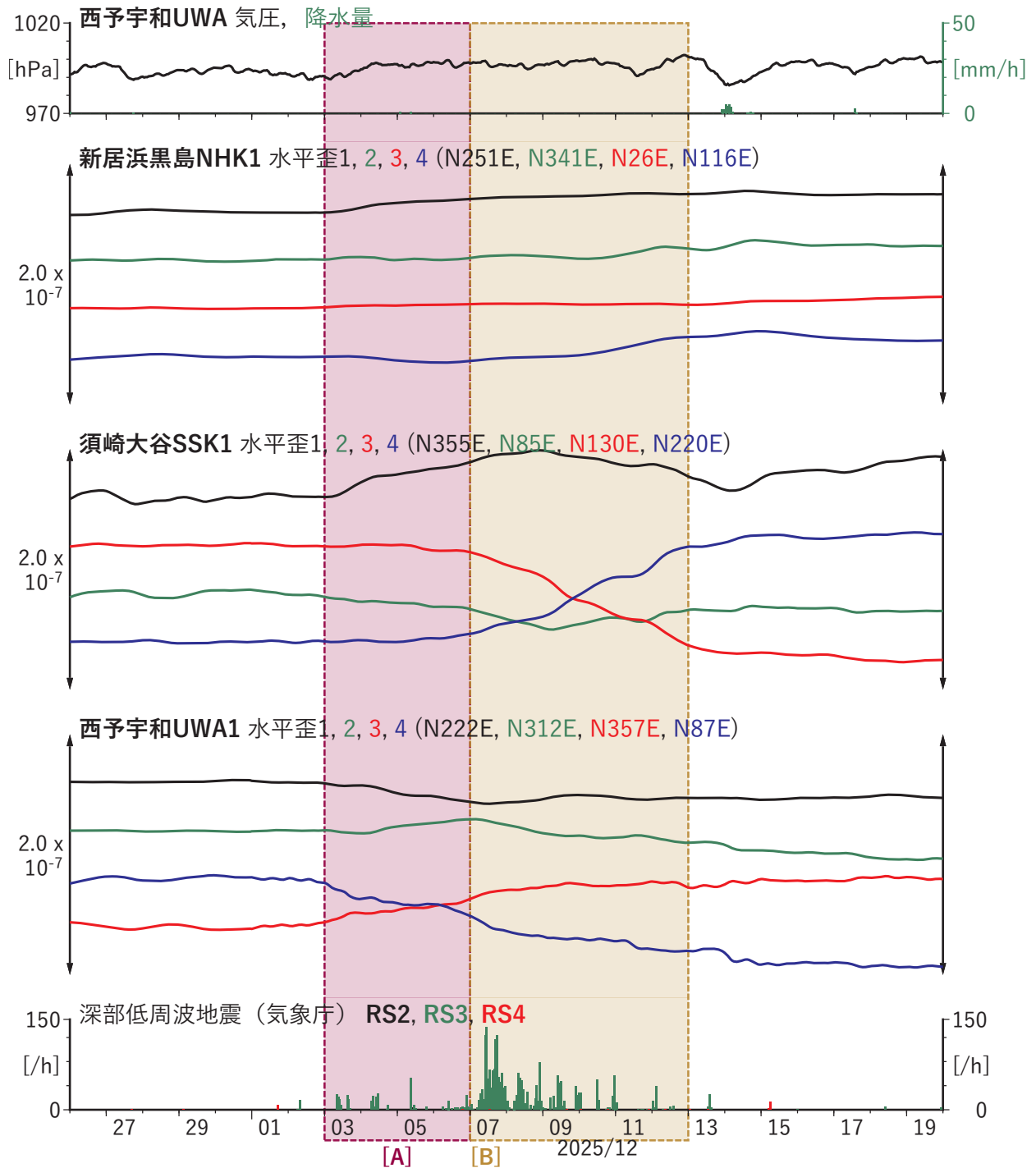
第 16 図 四国地域における歪・傾斜の観測結果と低周波地震の検出数 (2025/11/26–2025/12/19)。
