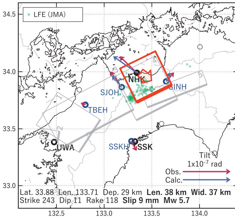
第 9 図 第 8 図 [A] を説明する断層モデル. 各図の説明は第 3 図を参照.
