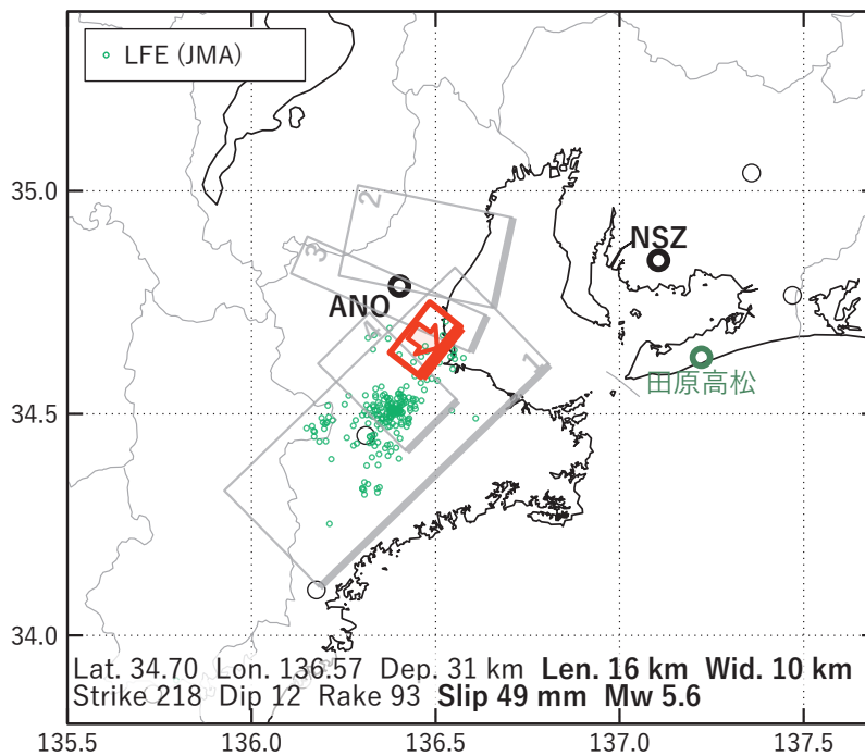
第 38 図 第 35 図 [C] を説明する断層モデル. 各図の説明は第 3 図を参照.
