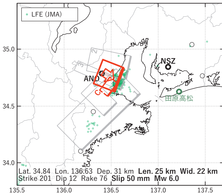
第 39 図 第 35 図 [D] を説明する断層モデル. 各図の説明は第 3 図を参照.
