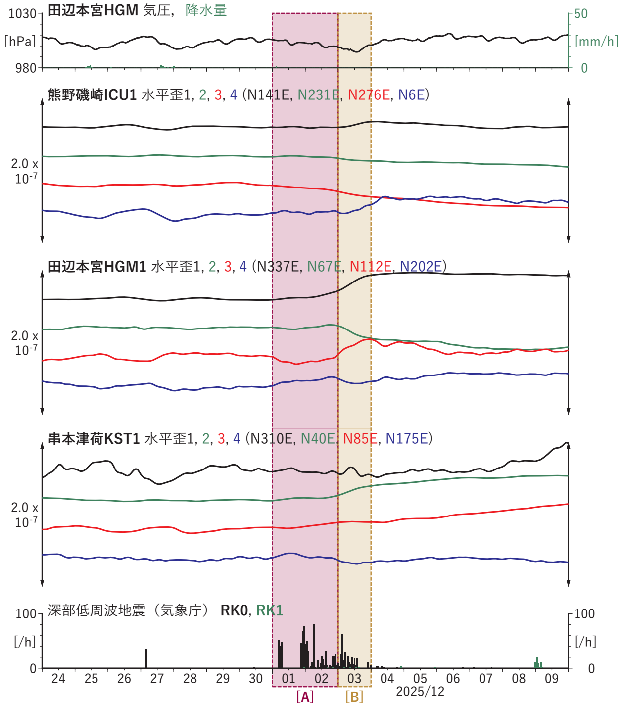
第 12 図 紀伊半島における歪の観測結果と低周波地震の検出数 (2025/11/24–2025/12/09)。
