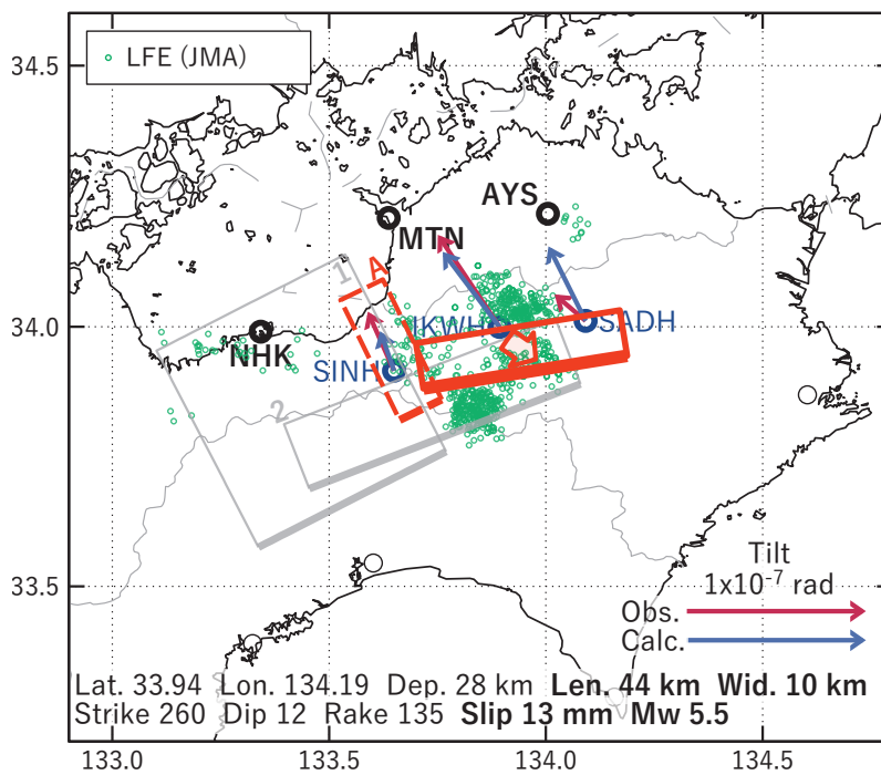
第 29 図 第 27 図 [B] を説明する断層モデル。各図の説明は第 3 図を参照。
