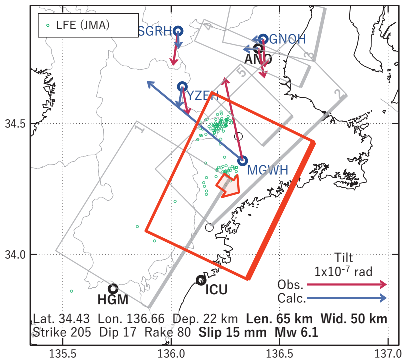
第 6 図 第 5 図 [A] を説明する断層モデル。各図の説明は第 3 図を参照。
