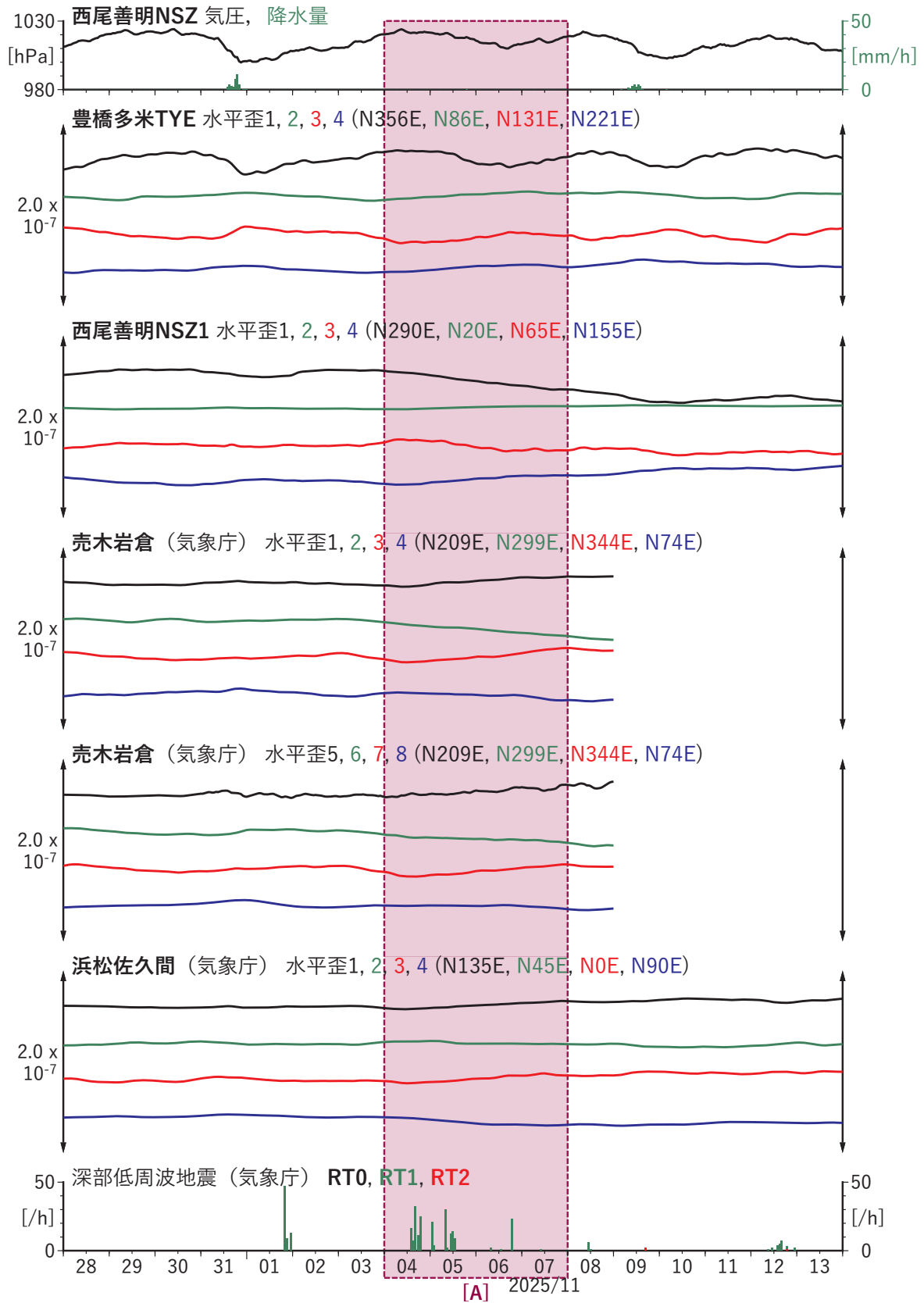
第 2 図 東海地域における歪・傾斜の観測結果と低周波地震の検出数 (2025/10/28–2025/11/14)。
