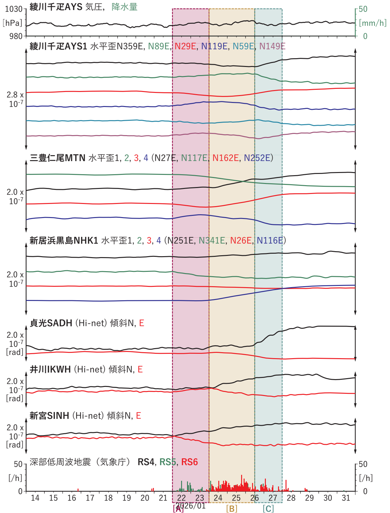
第 27 図 四国地域における歪・傾斜の観測結果と低周波地震の検出数 (2026/01/14–2026/02/01).
