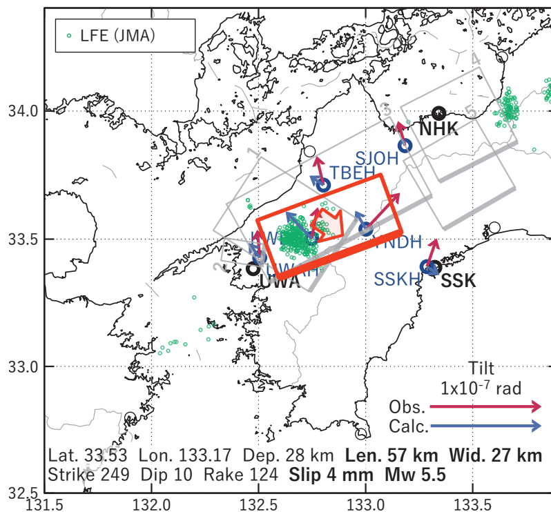
第 17 図 第 16 図 [A] を説明する断層モデル. 各図の説明は第 3 図を参照.
