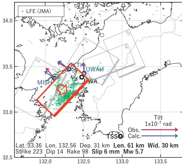
第 24 図 第 23 図 [A] を説明する断層モデル。各図の説明は第 3 図を参照。
