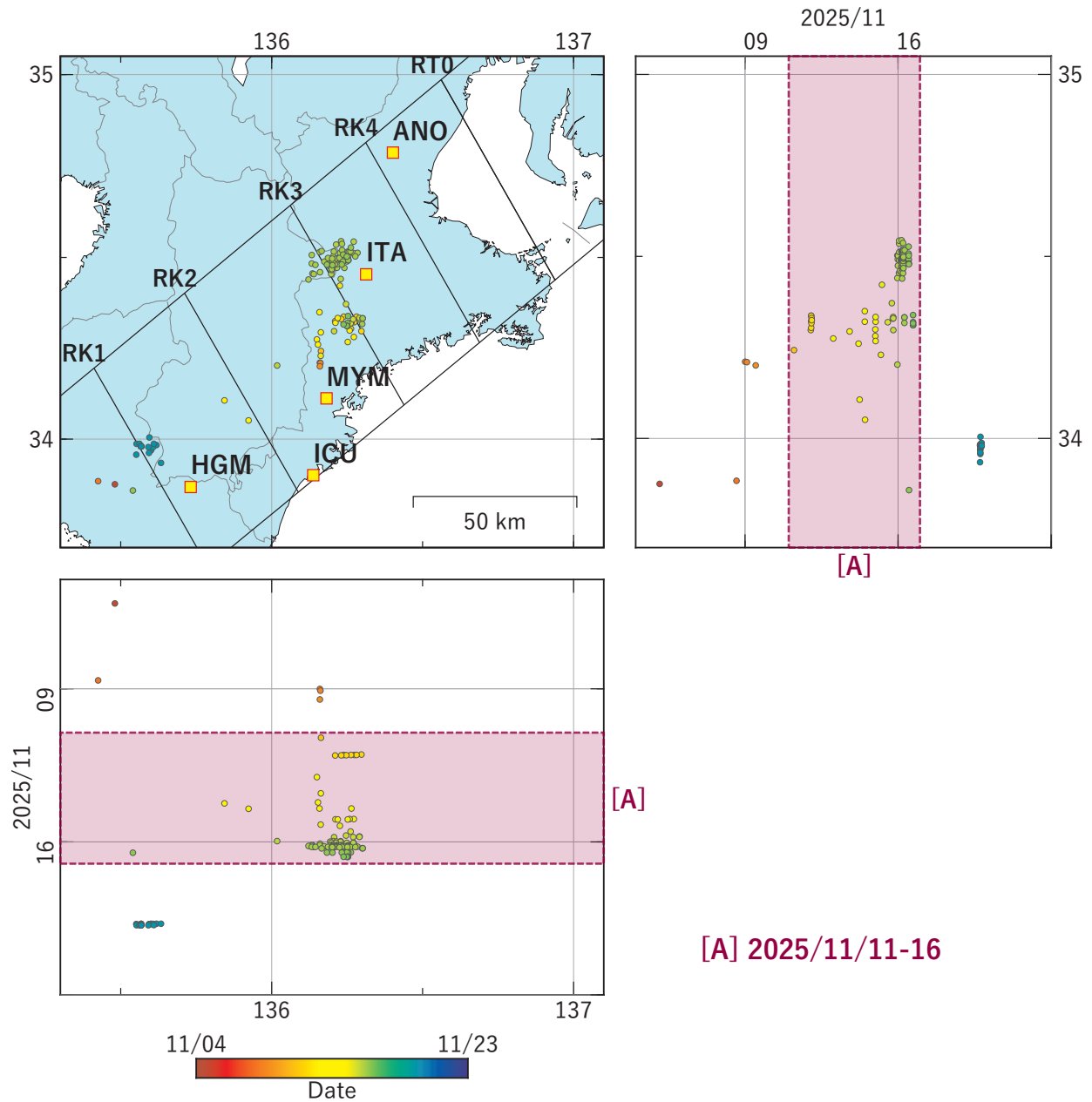
第 4 図 紀伊半島における低周波地震（気象庁一元化カタログによる）の時空間分布（2025/11/04–2025/11/22）.
