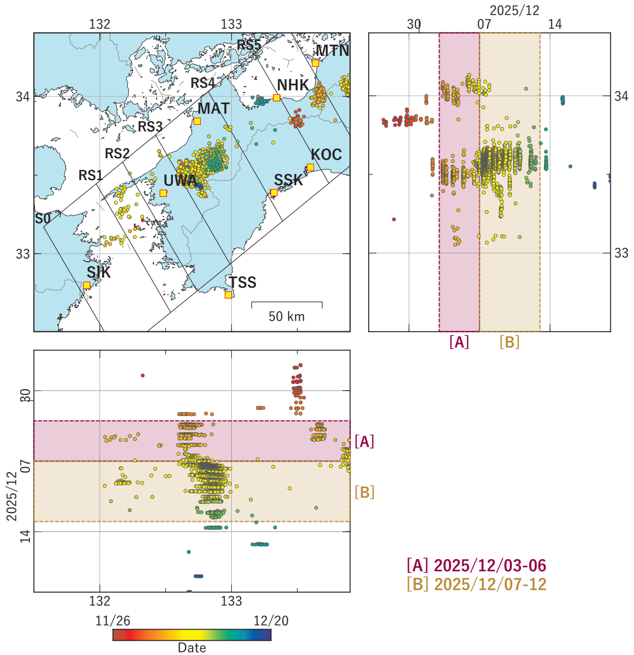
第 15 図 四国地域における低周波地震（気象庁一元化カタログによる）の時空間分布（2025/11/26–2025/12/19）.
