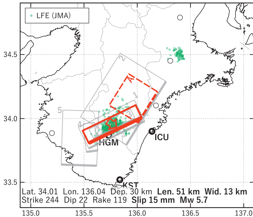
第 37 図 第 35 図 [B] を説明する断層モデル. 各図の説明は第 3 図を参照.
