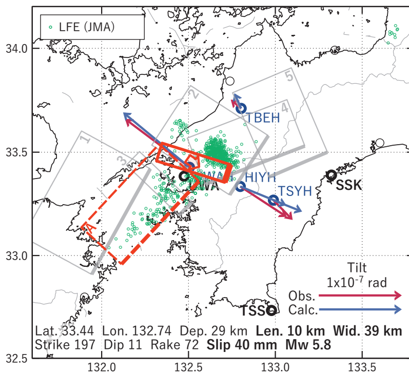
第 25 図 第 23 図 [B] を説明する断層モデル. 各図の説明は第 3 図を参照.
