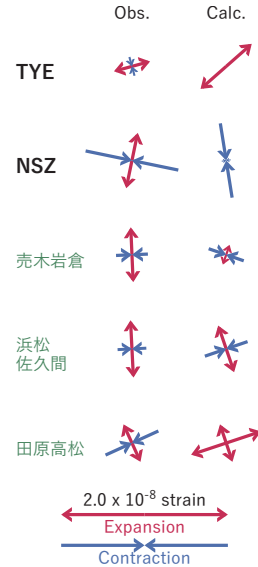
第 3 図 第 2 図 [A] を説明する断層モデル。以下の凡例の説明は以降の同様の図に共通。(図によっては気象庁・静岡県・防災科研 Hi-net の観測点や (b3) 体積歪の結果はない場合がある。) 黒・緑・青の丸印はそれぞれ産総研・気象庁および静岡県・防災科研 Hi-net の観測点、緑の小さな丸印は気象庁の推定した低周波地震。(a) 1 段階目の結果。灰色の濃淡は残差の総和で、赤色矩形が残差の総和が最小となる断層面の位置(大きさは 20x20 km で固定)。(b1) 2 段階目の結果。赤色矩形が残差の総和が最小となる断層面。矢印は傾斜の観測値と計算値の比較。灰色矩形は最近周辺で発生した短期的 SSE の推定断層面(番号との対応は本文参照)。(b2) 主歪の観測値と(b1)に示した断層モデルから求めた計算値との比較。(b3) 体積歪の観測値と(b1)に示した断層モデルから求めた計算値との比較。
