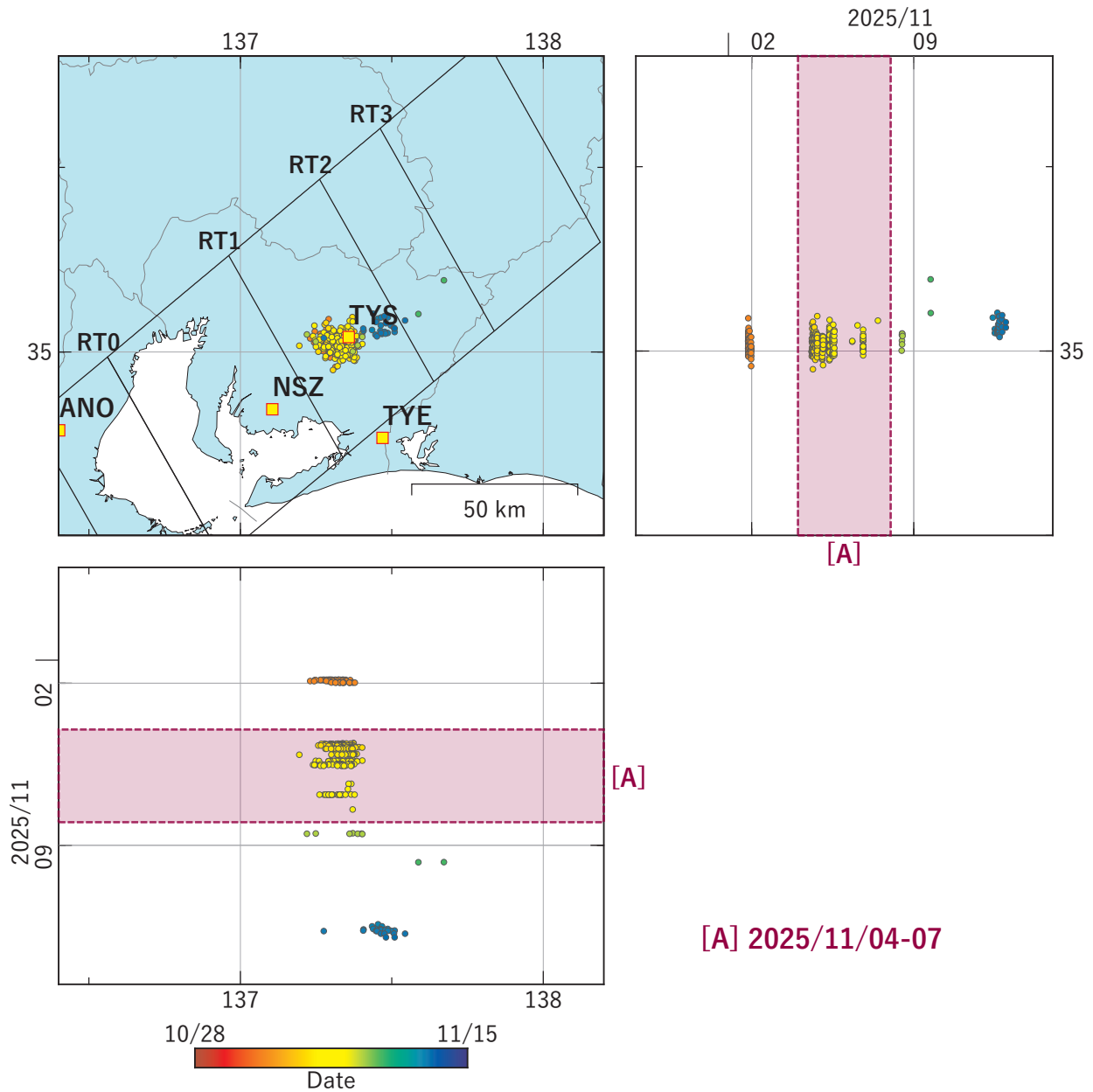
第 1 図 東海地域における低周波地震（気象庁一元化カタログによる）の時空間分布（2025/10/28–2025/11/14）.
