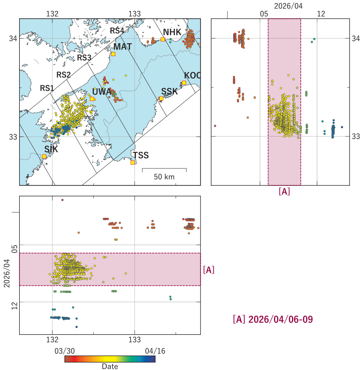
第 42 図 四国地域における低周波地震（気象庁一元化カタログによる）の時空間分布（2026/03/30–2026/04/15）.
