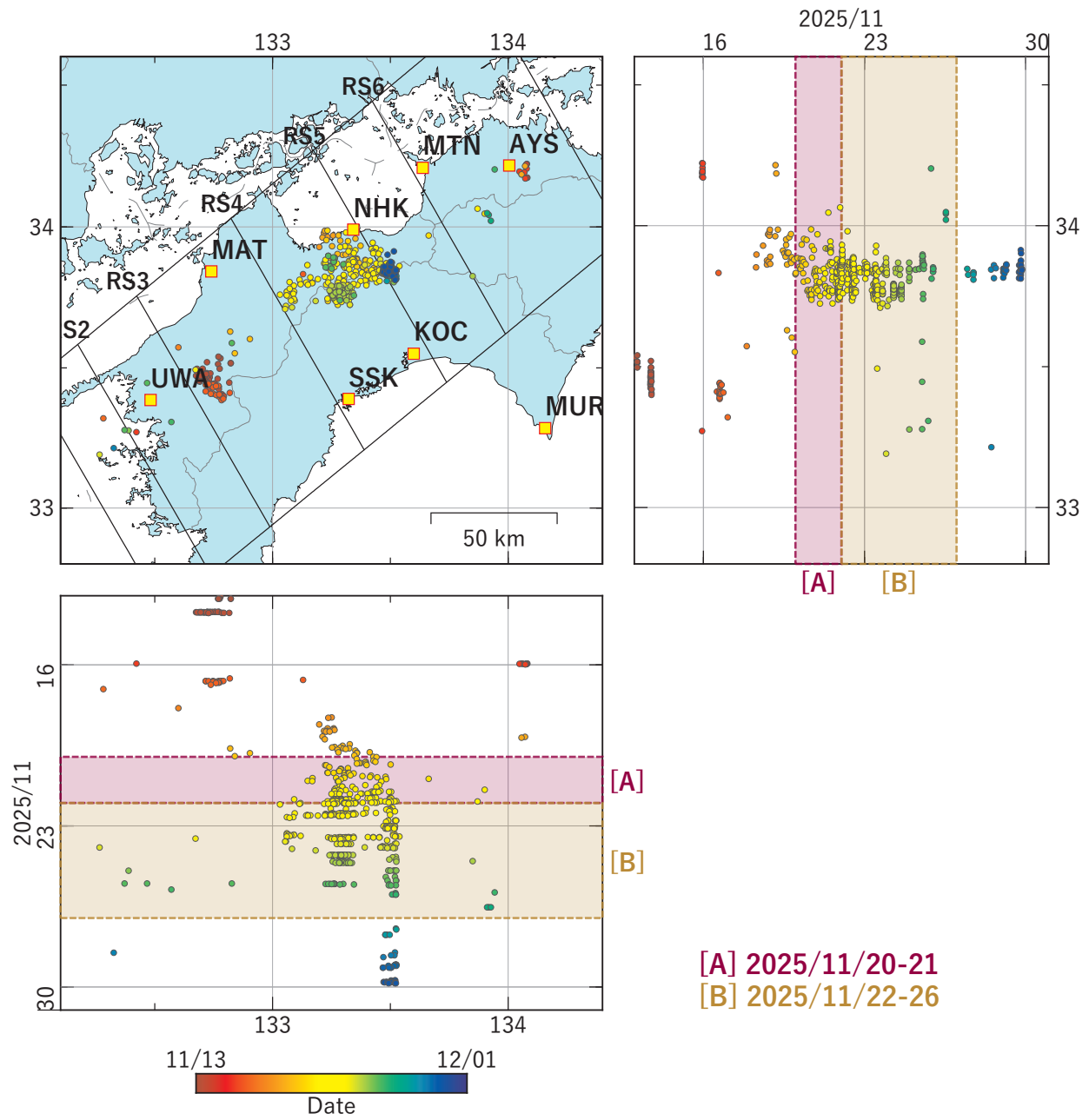
第 7 図 四国地域における低周波地震（気象庁一元化カタログによる）の時空間分布（2025/11/13–2025/11/30）.
