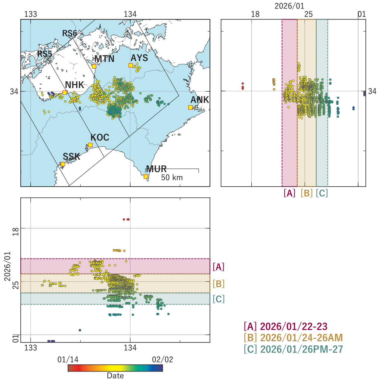
第 26 図 四国地域における低周波地震（気象庁一元化カタログによる）の時空間分布（2026/01/14-2026/02/01）.
