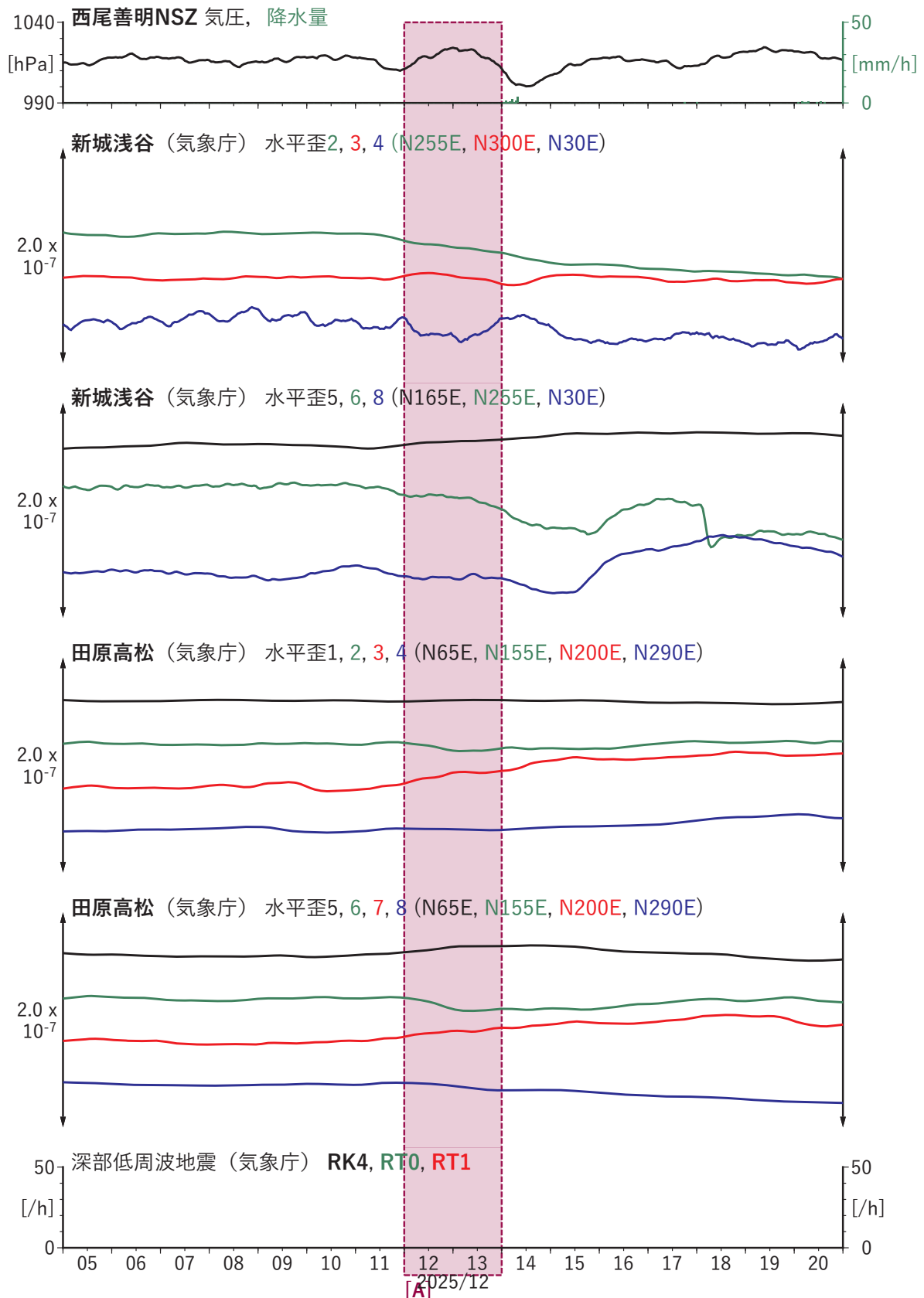
第 20 図 東海地域における歪の観測結果と低周波地震の検出数 (2025/12/05–2025/12/20)。
