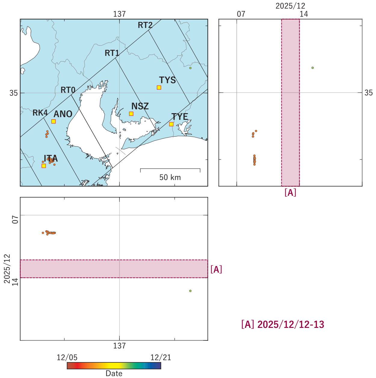
第 19 図 東海地域における低周波地震（気象庁一元化カタログによる）の時空間分布（2025/12/05–2025/12/20）.
