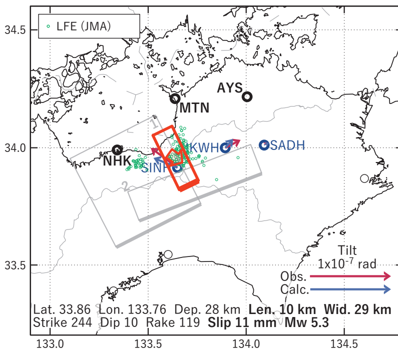
第 28 図 第 27 図 [A] を説明する断層モデル。各図の説明は第 3 図を参照。
