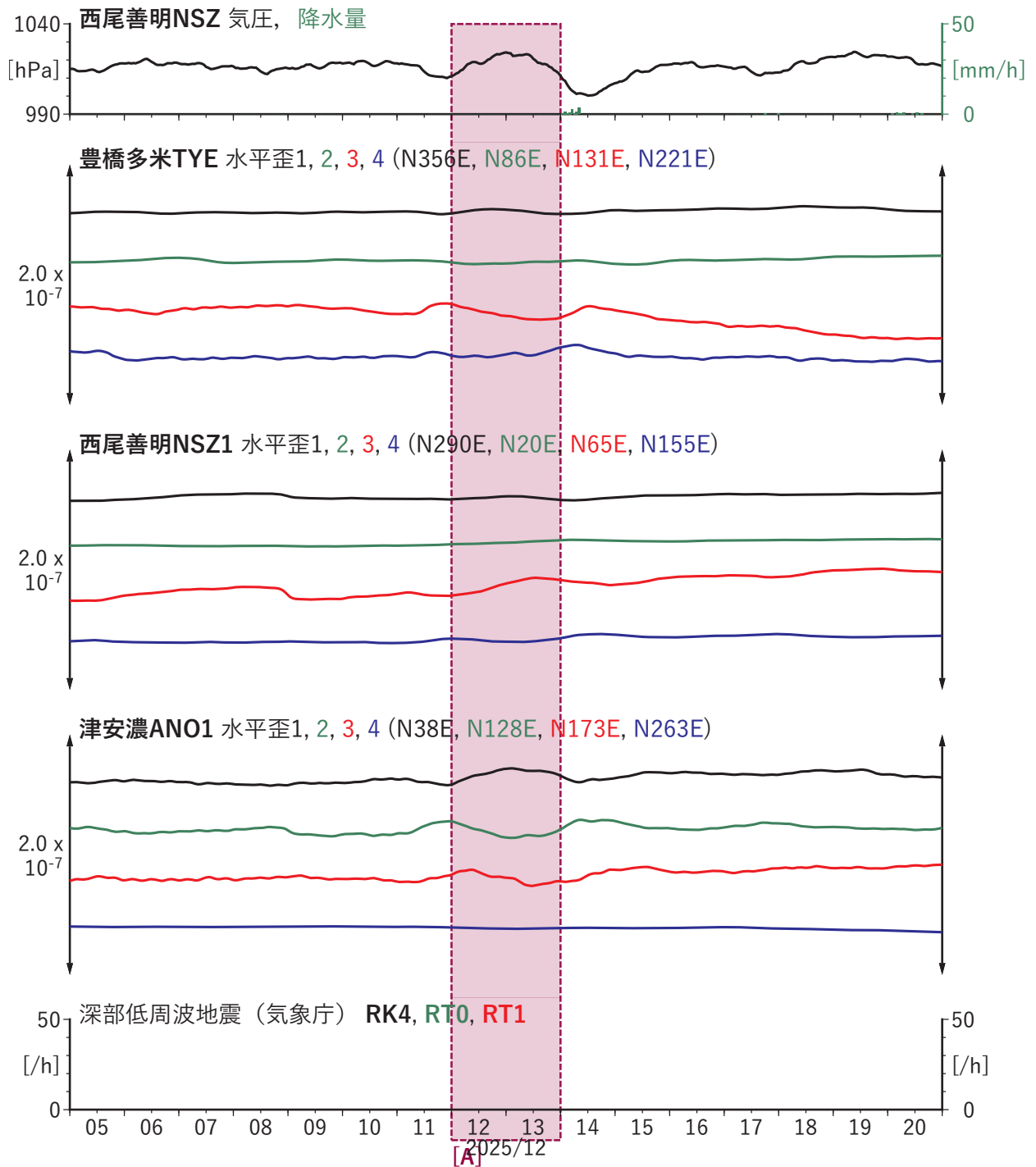
第 20 図 東海地域における歪の観測結果と低周波地震の検出数 (2025/12/05–2025/12/20)。
