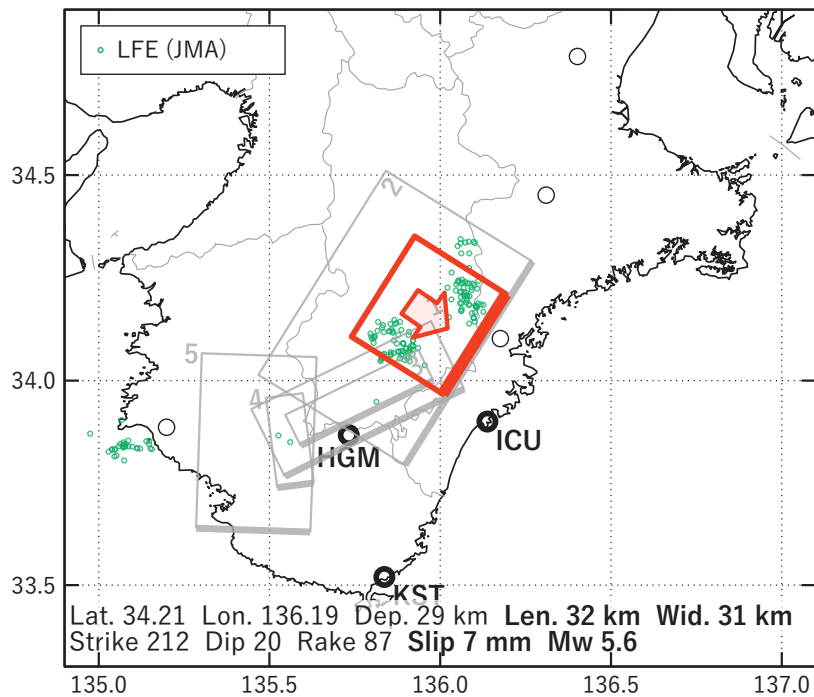
第 36 図 第 35 図 [A] を説明する断層モデル. 各図の説明は第 3 図を参照.
