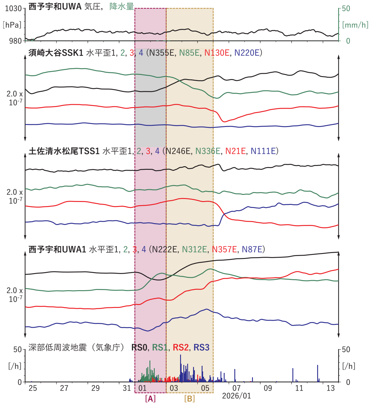
第 23 図 四国地域における歪・傾斜の観測結果と低周波地震の検出数 (2025/12/25–2026/01/13)。
