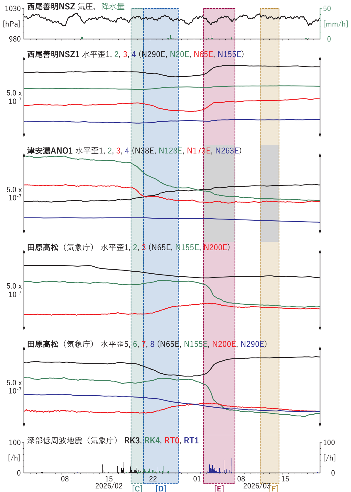
第 35 図 東海地域～紀伊半島における歪・傾斜の観測結果と低周波地震の検出数 (2026/02/02–2026/03/20)。
