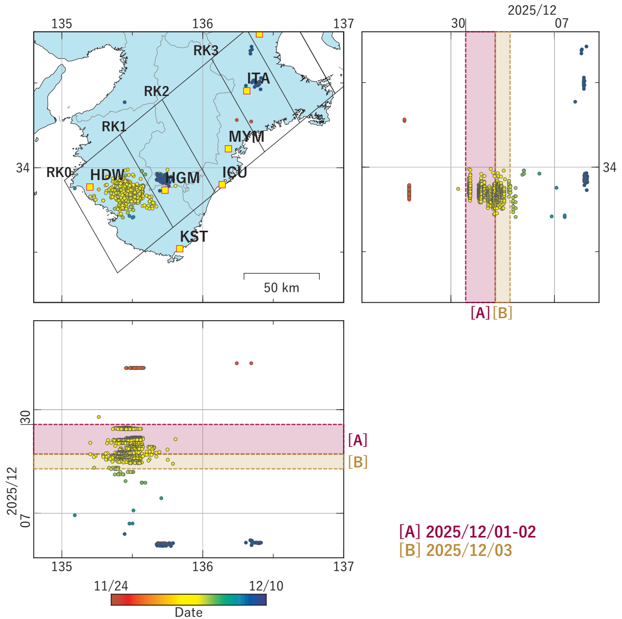
第 11 図 紀伊半島における低周波地震（気象庁一元化カタログによる）の時空間分布（2025/11/24–2025/12/09）.
