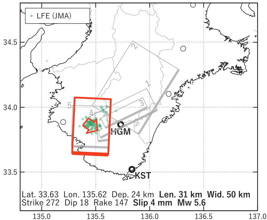
第 33 図 第 32 図 [A] を説明する断層モデル. 各図の説明は第 3 図を参照.
