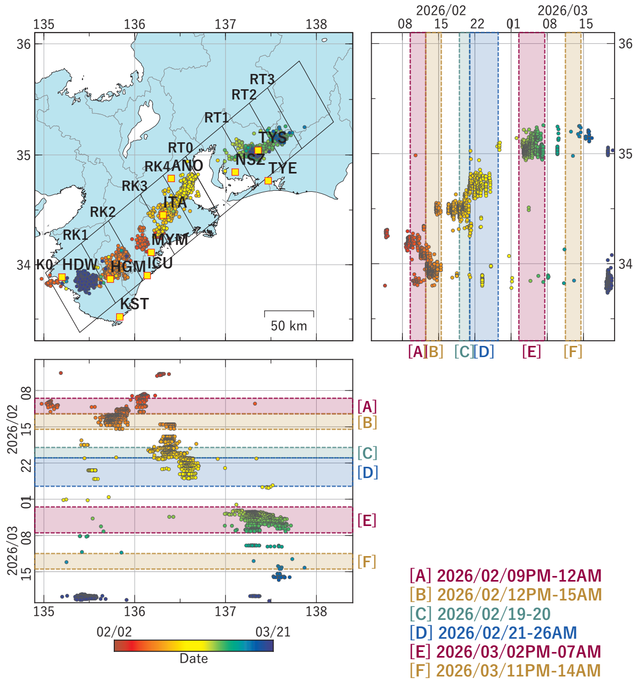
第 34 図 東海地域～紀伊半島における低周波地震（気象庁一元化カタログによる）の時空間分布（2026/02/02–2026/03/20）。
