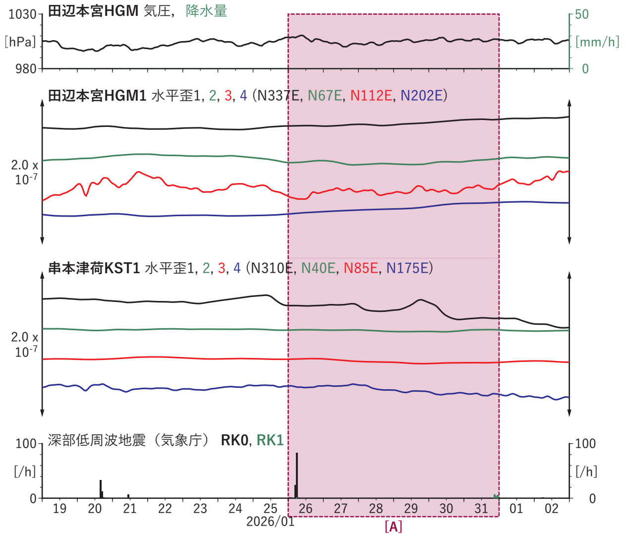
第 32 図 紀伊半島における歪の観測結果と低周波地震の検出数 (2026/01/19–2026/02/02)。
