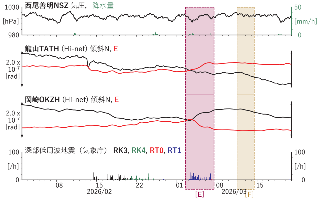
第 35 図 東海地域～紀伊半島における歪・傾斜の観測結果と低周波地震の検出数（2026/02/02–2026/03/20）.
