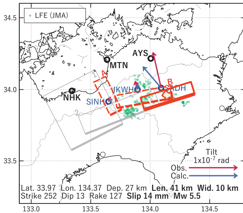
第 30 図 第 27 図 [C] を説明する断層モデル。各図の説明は第 3 図を参照。
