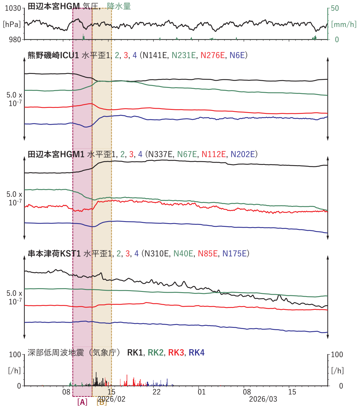
第 35 図 東海地域～紀伊半島における歪・傾斜の観測結果と低周波地震の検出数 (2026/02/02–2026/03/20)。
