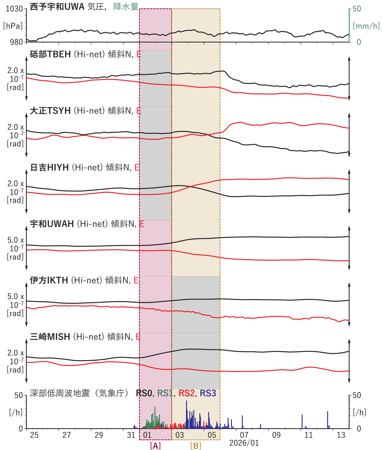
第 23 図 四国地域における歪・傾斜の観測結果と低周波地震の検出数 (2025/12/25–2026/01/13)。
