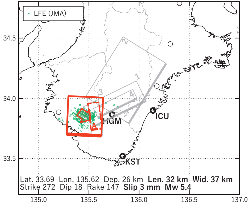
第 14 図 第 12 図 [B] を説明する断層モデル. 各図の説明は第 3 図を参照.
