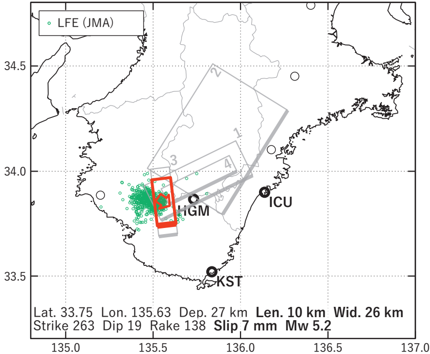
第 13 図 第 12 図 [A] を説明する断層モデル. 各図の説明は第 3 図を参照.
