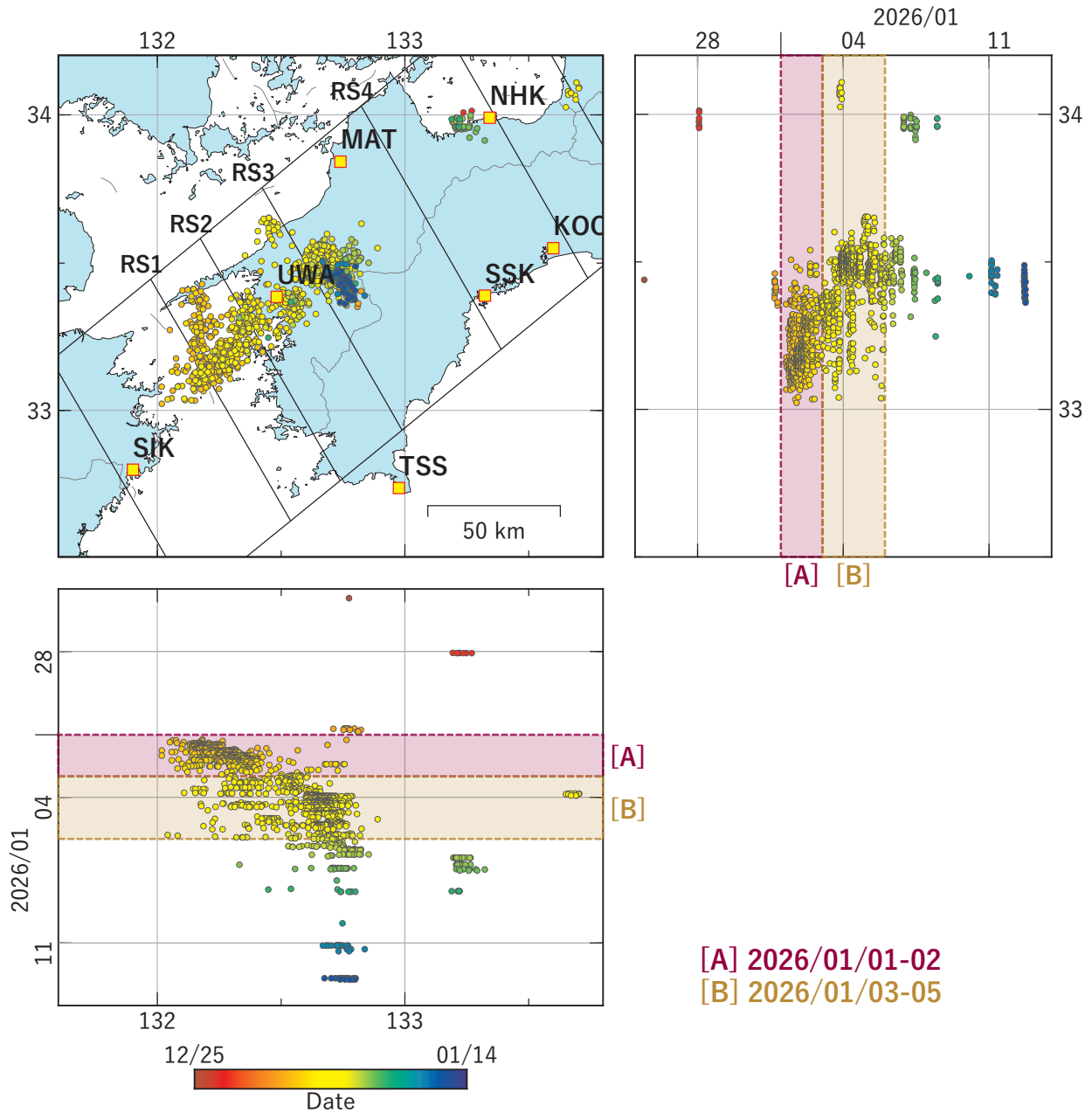
第 22 図 四国地域における低周波地震（気象庁一元化カタログによる）の時空間分布（2025/12/25–2026/01/13）。
