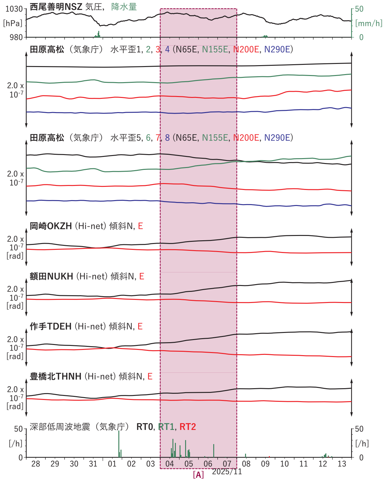
第 2 図 東海地域における歪・傾斜の観測結果と低周波地震の検出数 (2025/10/28–2025/11/14)。
