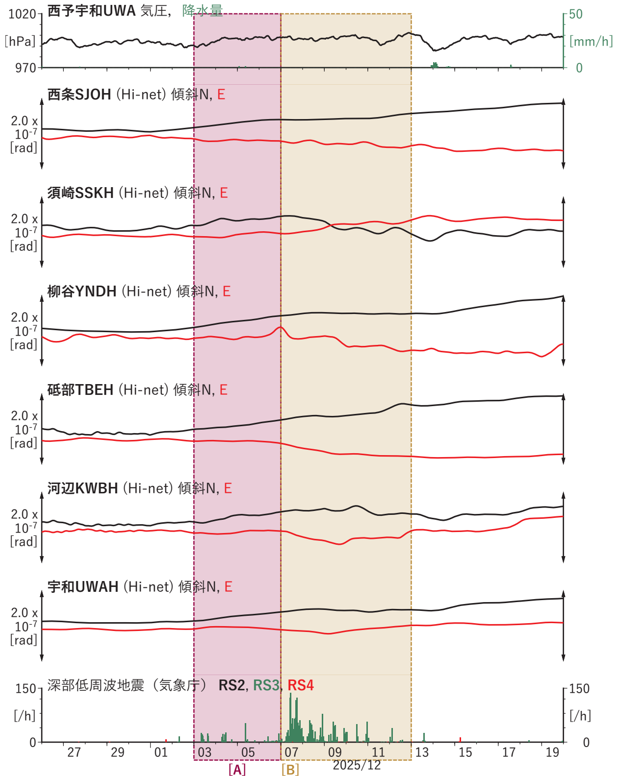
第 16 図 四国地域における歪・傾斜の観測結果と低周波地震の検出数 (2025/11/26–2025/12/19).
