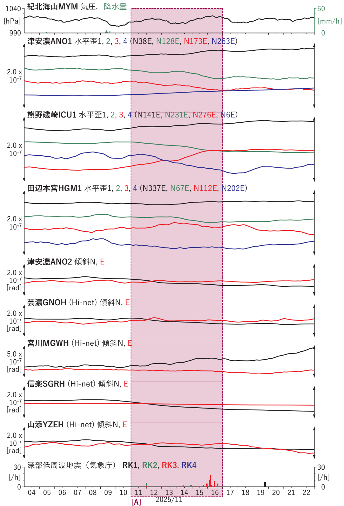
第 5 図 紀伊半島における歪・傾斜の観測結果と低周波地震の検出数 (2025/11/04–2025/11/22)。
