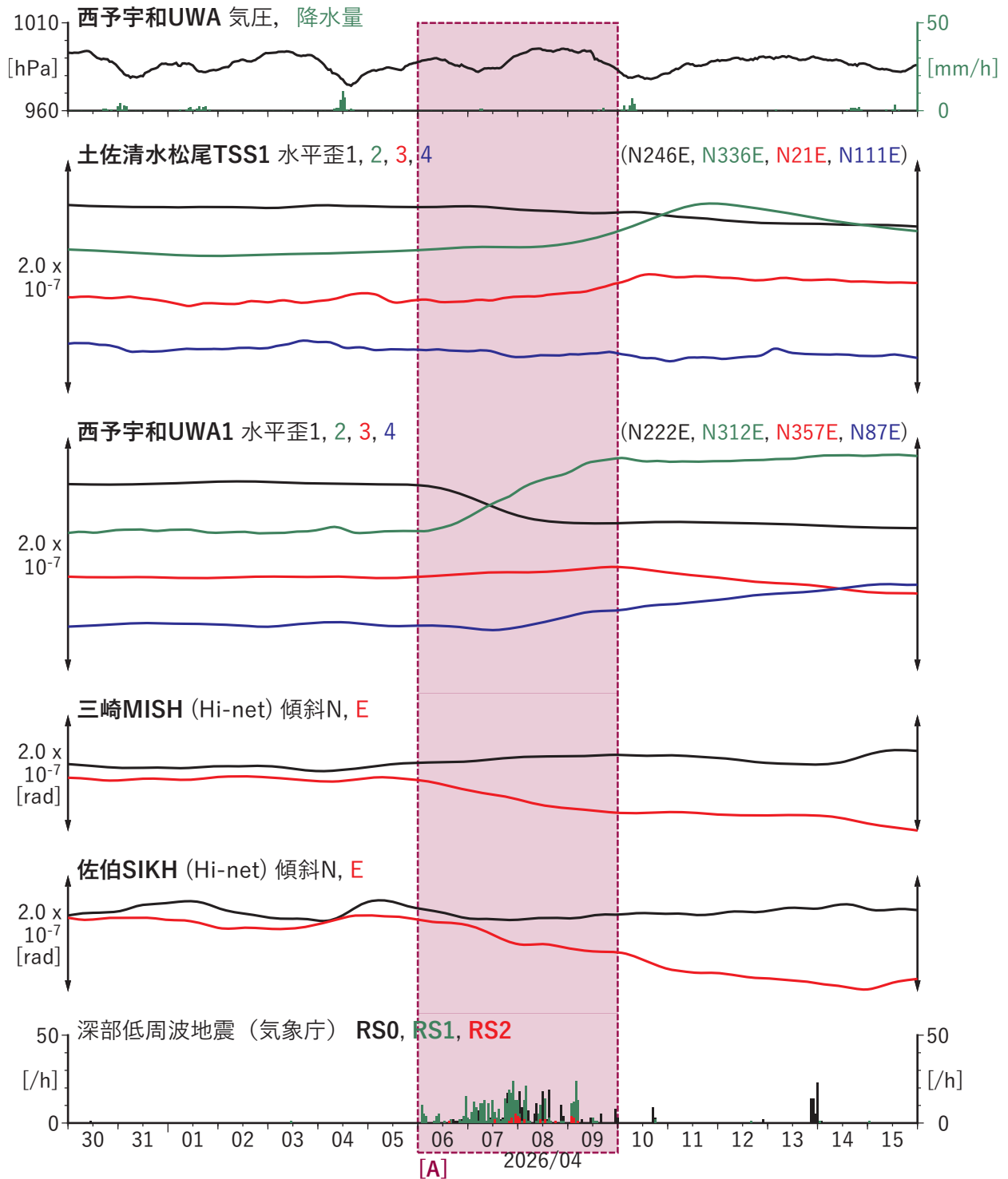
第 43 図 四国地域における歪・傾斜の観測結果と低周波地震の検出数 (2026/03/30–2026/04/15)。
