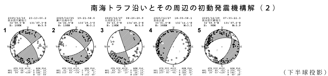
第 3 図 (b) つづき (2025 年 11 月～2026 年 1 月) Fig. 3(b) Continued (November 2025 – January 2026).
