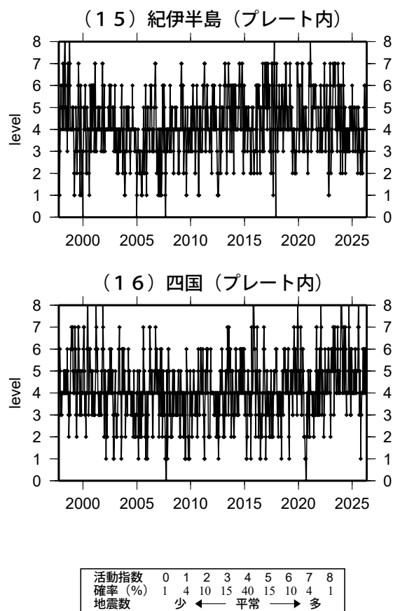
第 19 図 (d) つづき
