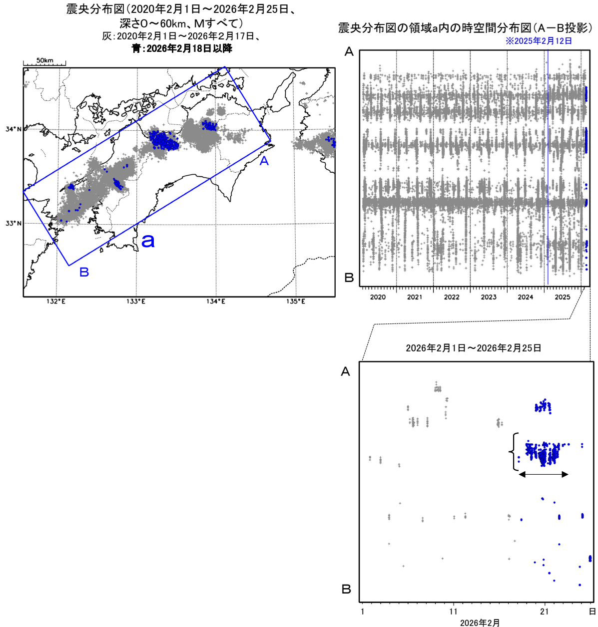
第 14 図 (a) 四国中部の深部低周波地震活動とひずみ変化, 及び推定されるゆっくりすべり領域
