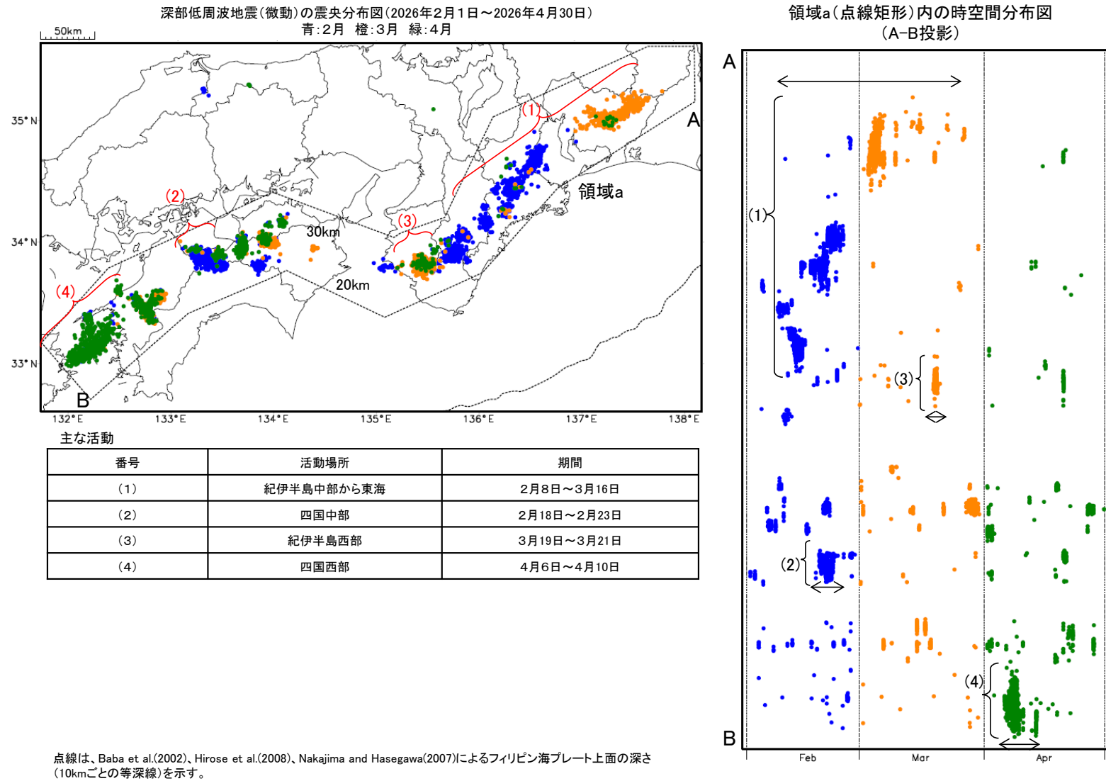
第2図(c) 東海地域から豊後水道にかけての深部低周波地震活動(2026年2月～4月)。
