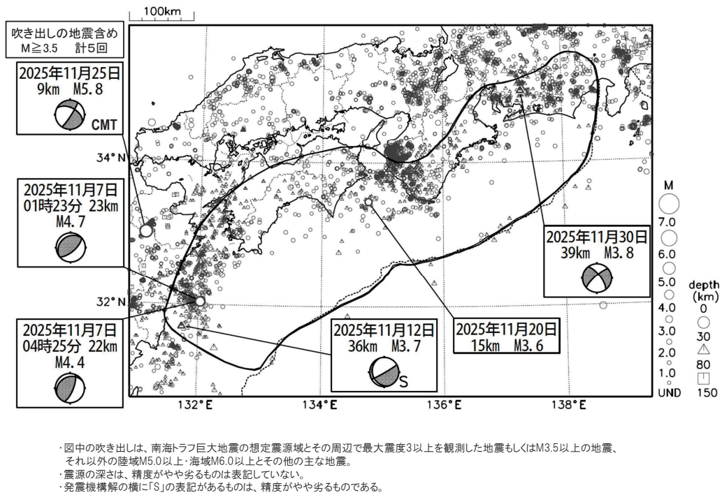
第 1 図 (a) 南海トラフ周辺の月別震央分布 (2025 年 11 月)
