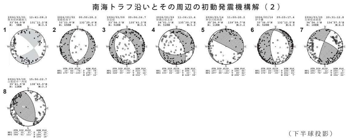
第 3 図 (e) つづき (2026 年 2 月～4 月)
