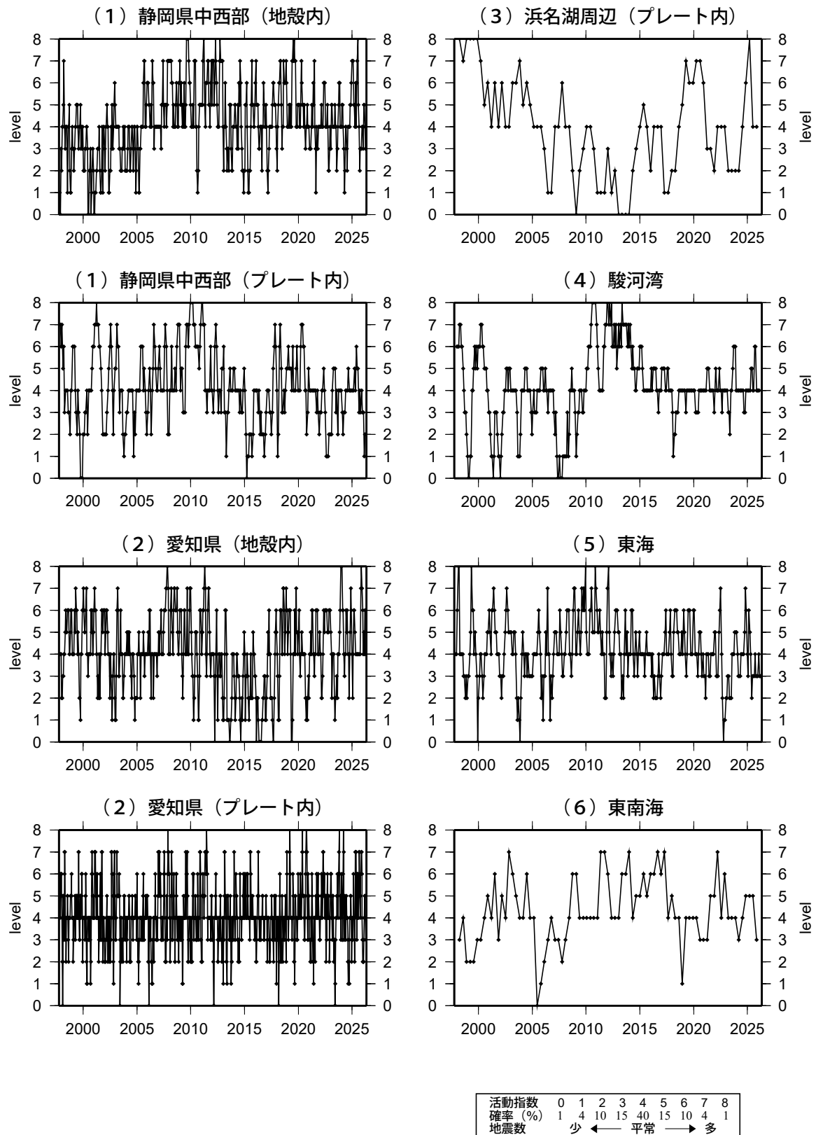
第 19 図 (b) 南海トラフ周辺の地震活動指数の推移
