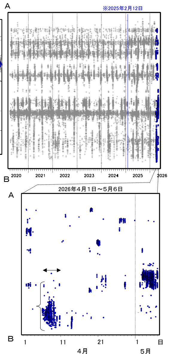
領域a内の時空間分布図(A-B投影)
