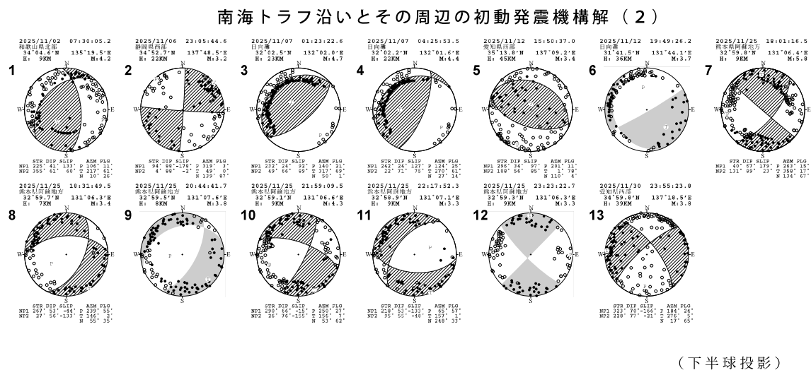
第 3 図 (a) 南海トラフ周辺で発生した主な地震の発震機構解 (2025 年 11 月～2026 年 1 月)
