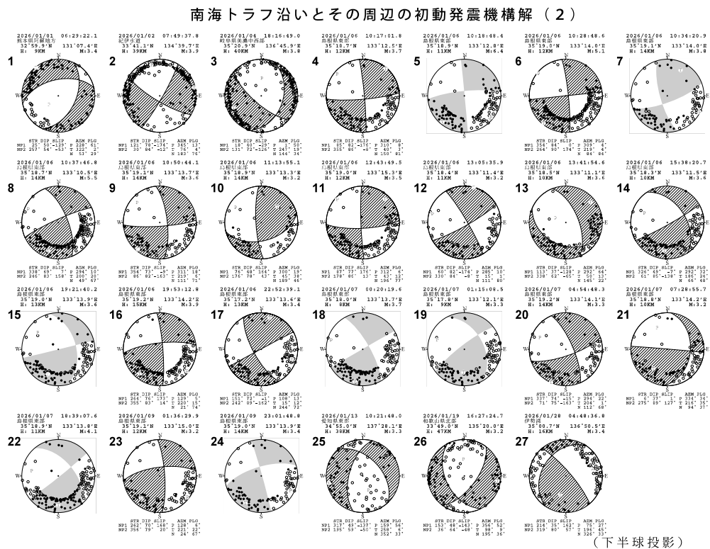
第 3 図 (c) つづき (2025 年 11 月～2026 年 1 月)
