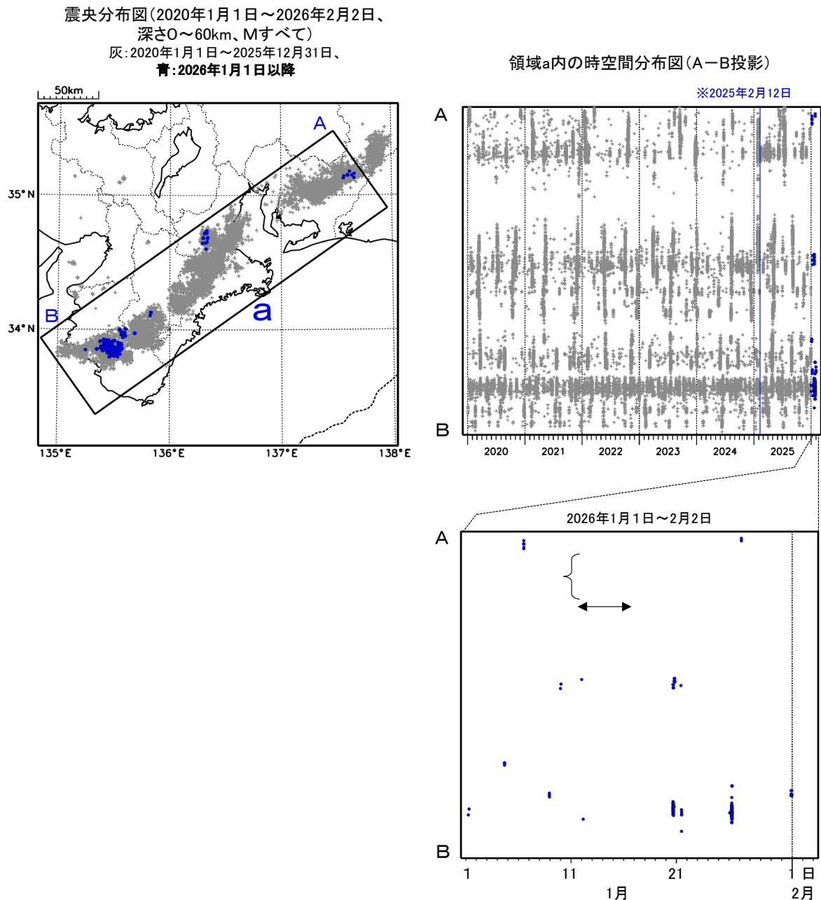
第 10 図 (a) 東海の深部低周波地震活動とひずみ変化、及び推定されるゆっくりすべり領域
