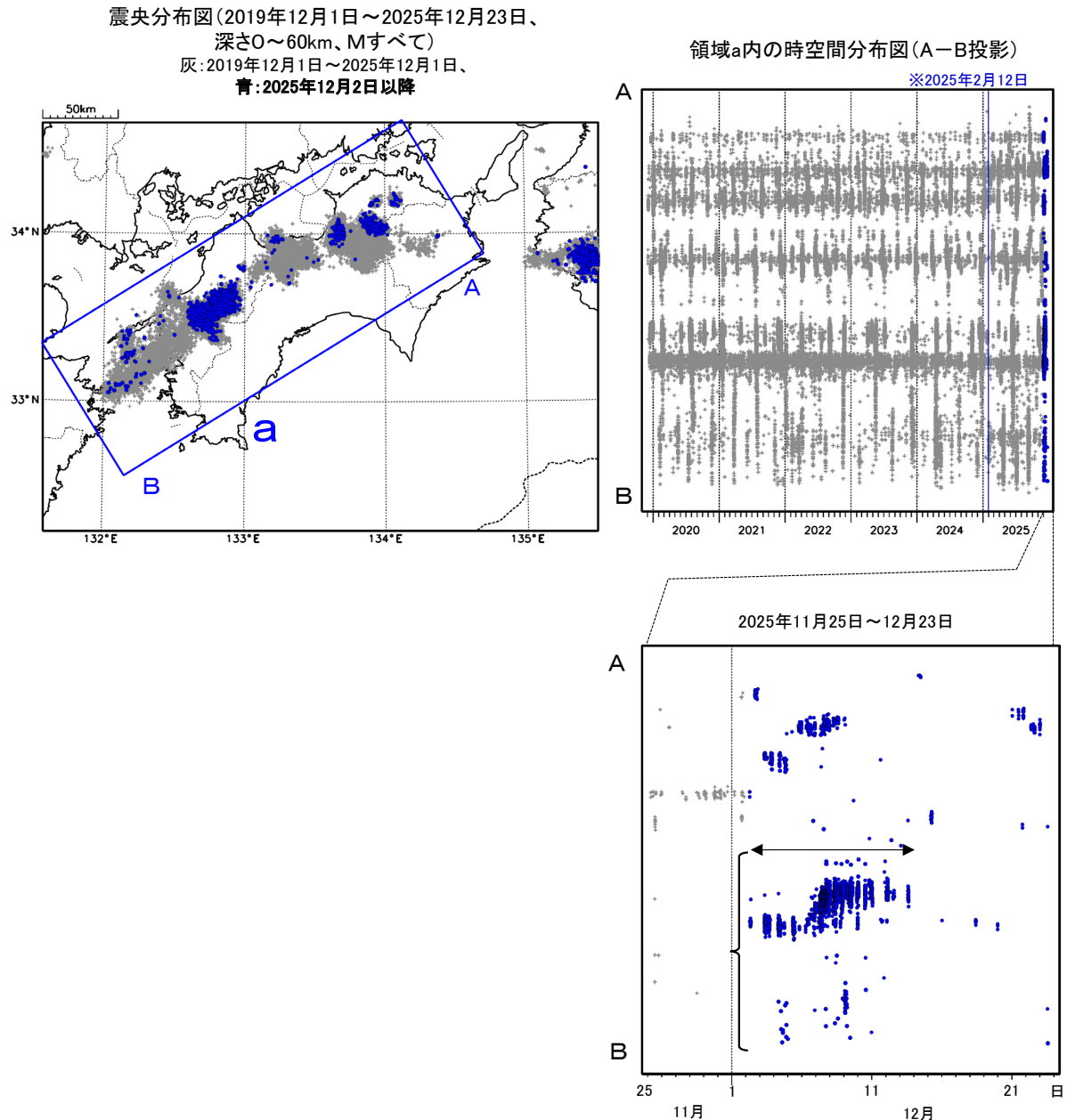
第 8 図 (a) 四国西部の深部低周波地震活動とひずみ変化, 及び推定されるゆっくりすべり領域
