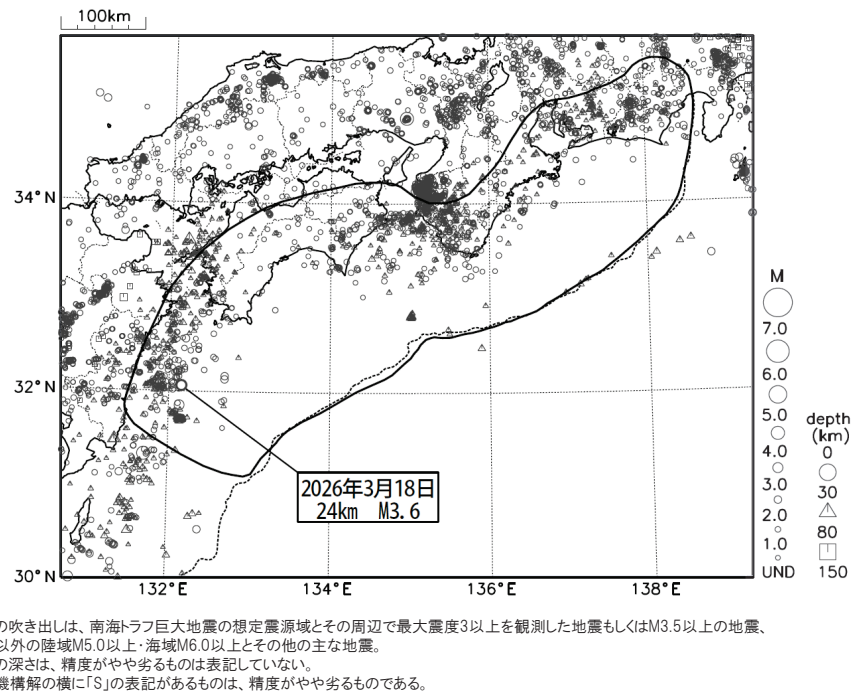
第 1 図 (e) つづき (2026 年 3 月)
