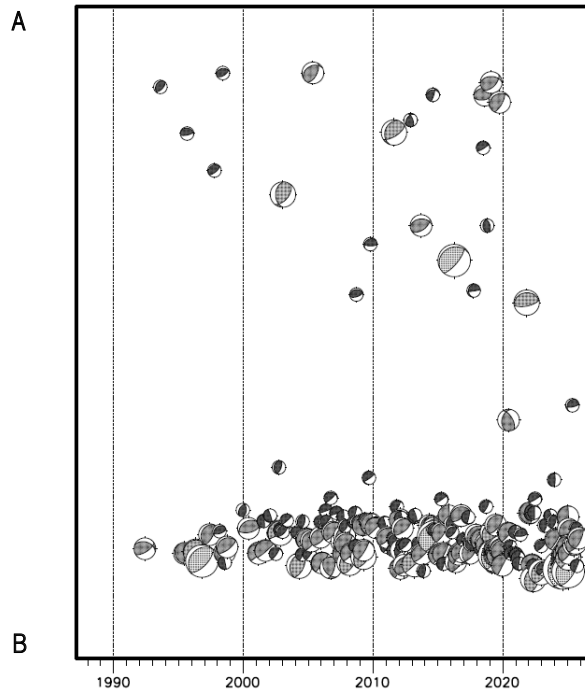
第 18 図 想定南海トラフ地震の発震機構解と類似の型の地震
