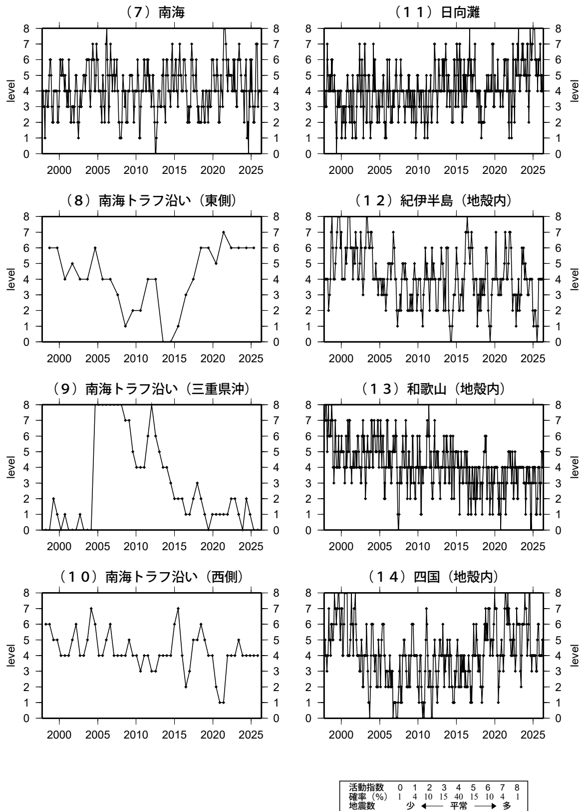
第 19 図 (c) つづき
