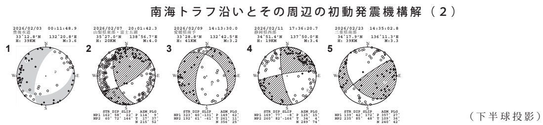
第 3 図 (d) つづき (2026 年 2 月～4 月)
