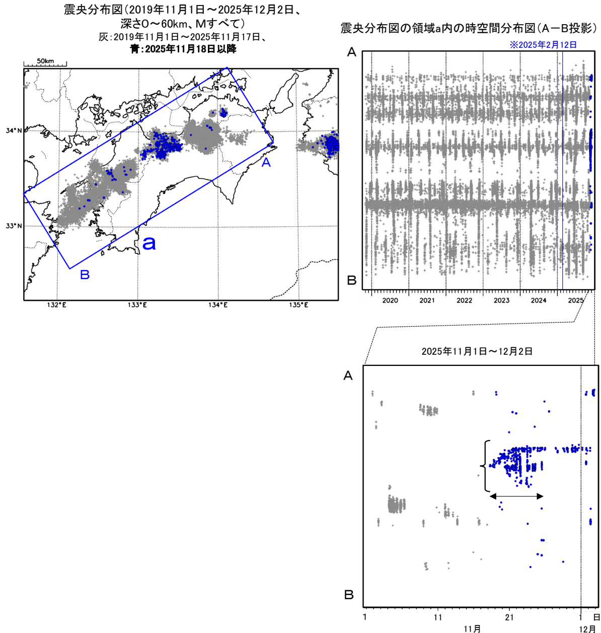
第 6 図 (a) 四国中部の深部低周波地震活動とひずみ変化，及び推定されるゆっくりすべり領域
