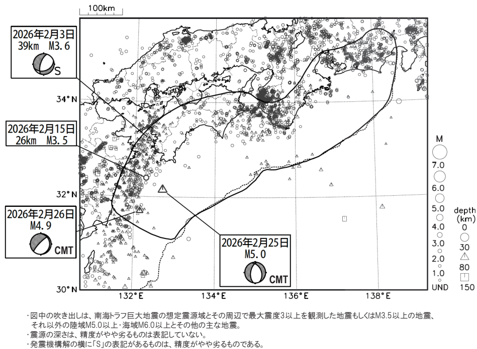
第 1 図 (d) つづき (2026 年 2 月)
