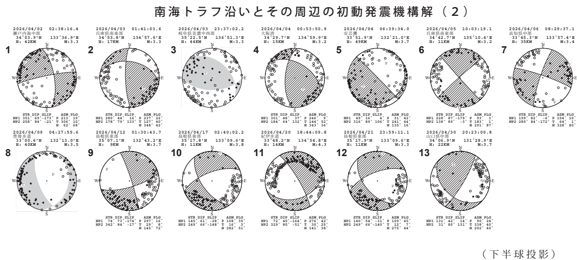
第 3 図 (f) つづき (2026 年 2 月～ 4 月)
