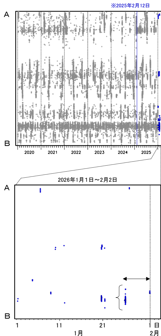
第 12 図 (a) 紀伊半島中部から紀伊半島西部の深部低周波地震活動とひずみ変化、及び推定されるゆっくりすべり領域
