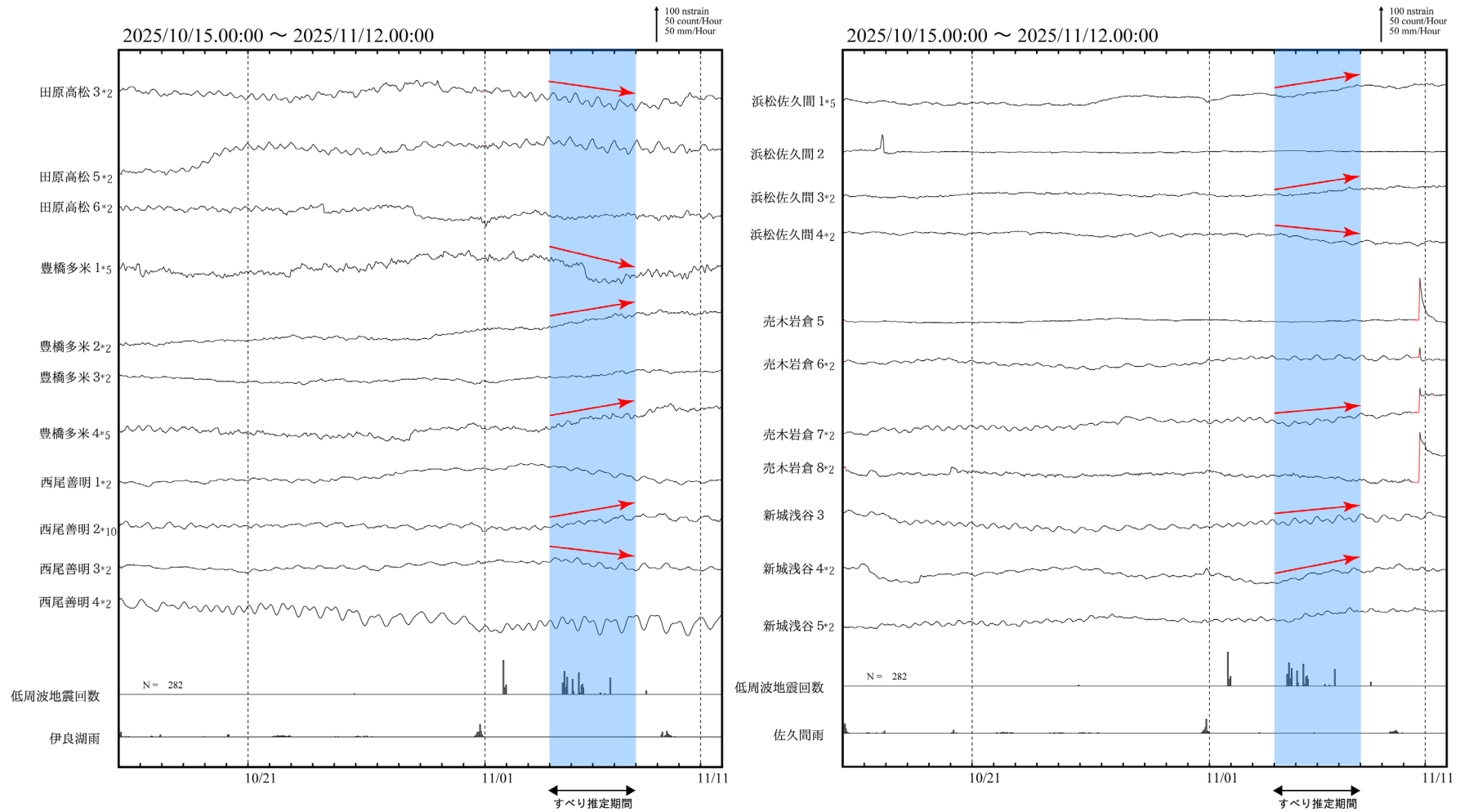
第 4 図 (b) つづき Fig. 4(b) Continued.
