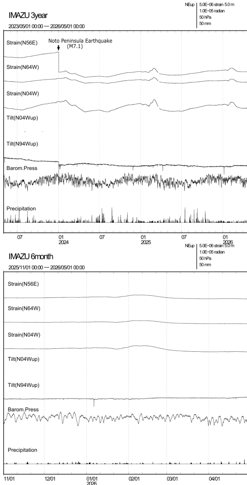
第 2 図 今津観測点における(上)2023 年 5 月～2026 年 4 月、(下)2025 年 11 月～2026 年 4 月のひずみ・傾斜変化(時間値)。毎年冬のひずみ・水位変化は、観測点付近の融雪のための地下水汲み上げに伴うもの。
