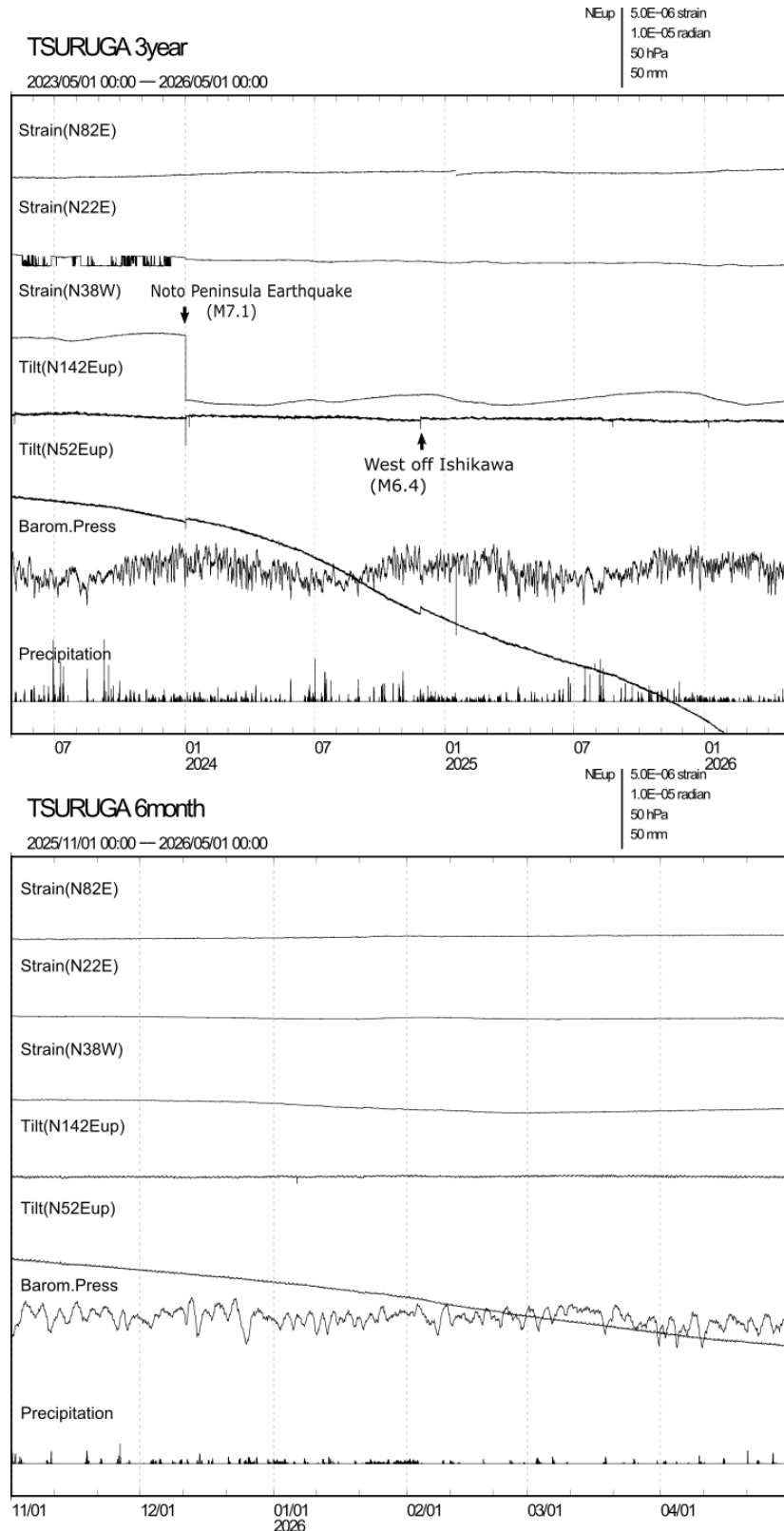
第 3 図 敦賀観測点における（上）2023 年 5 月～2026 年 4 月、（下）2025 年 11 月～2026 年 4 月のひずみ・傾斜変化（時間値）。
