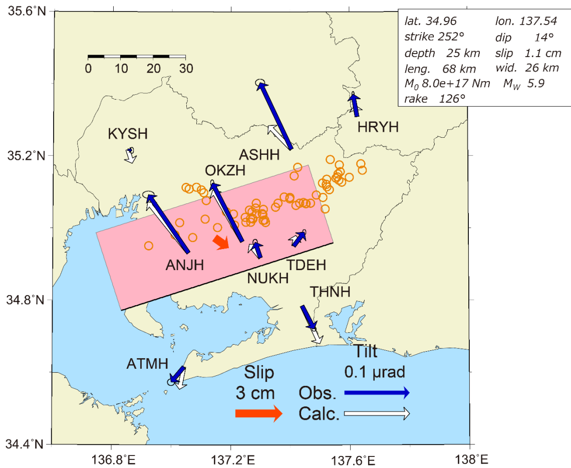
第 7 図 2026 年 3 月愛知県の短期的 SSE の断層モデル。図の見方は第 3 図と同じ。
