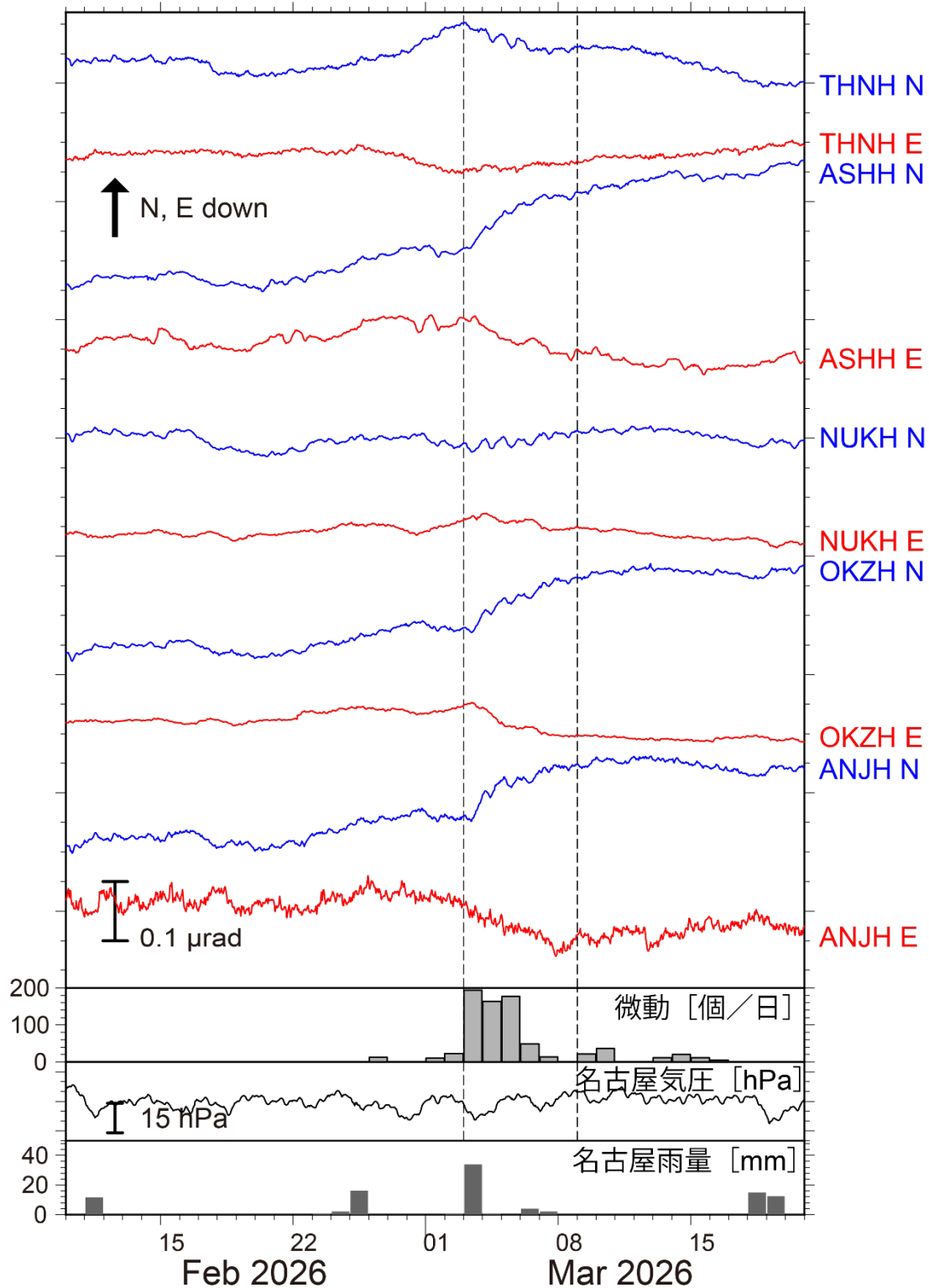
第 6 図 2026 年 2 月 10 日～3 月 20 日までの傾斜時系列。図の見方は第 2 図と同様。観測点位置は第 7 図に示した。3 月 3 日～8 日の傾斜変化量を SSE によるものと仮定した。愛知県周辺での微動活動度・気象庁名古屋観測点での気圧変化および雨量をあわせて表示した。
