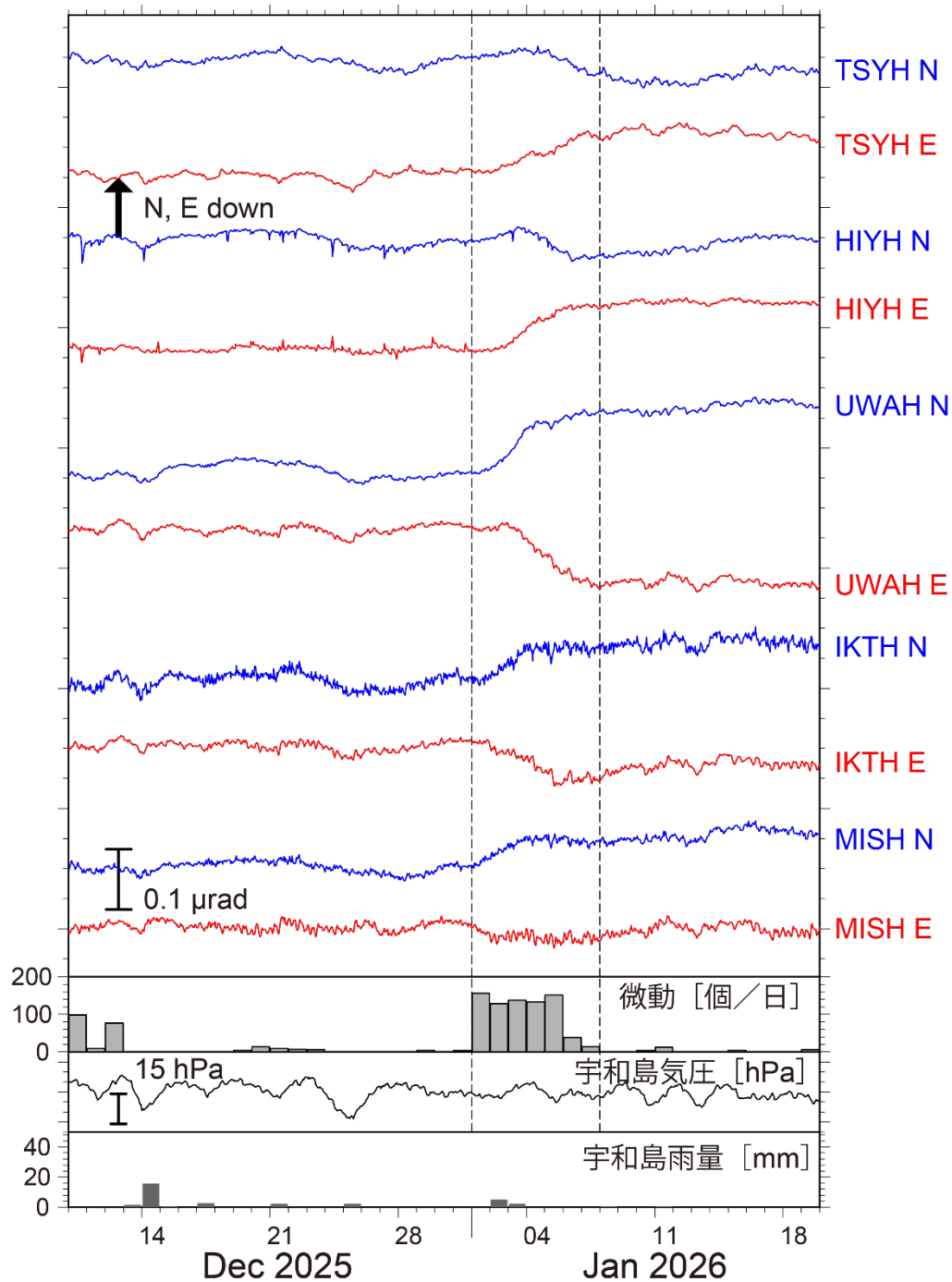
第 2 図 2025 年 12 月 10 日から 2026 年 1 月 19 日までの傾斜時系列。観測点位置は第 3 図に示した。記録は上方 向への変化が北・東下がり傾斜変動を表す。気圧応答・潮汐成分を BAYTAP-G 4) により除去し、直線ト レンドを補正した後の記録を示した。2026 年 1 月 1 日～7 日の傾斜変化量を SSE によるものと仮定した。 四国西部での微動活動度・気象庁宇和島観測点での気圧変化および雨量をあわせて表示した。
