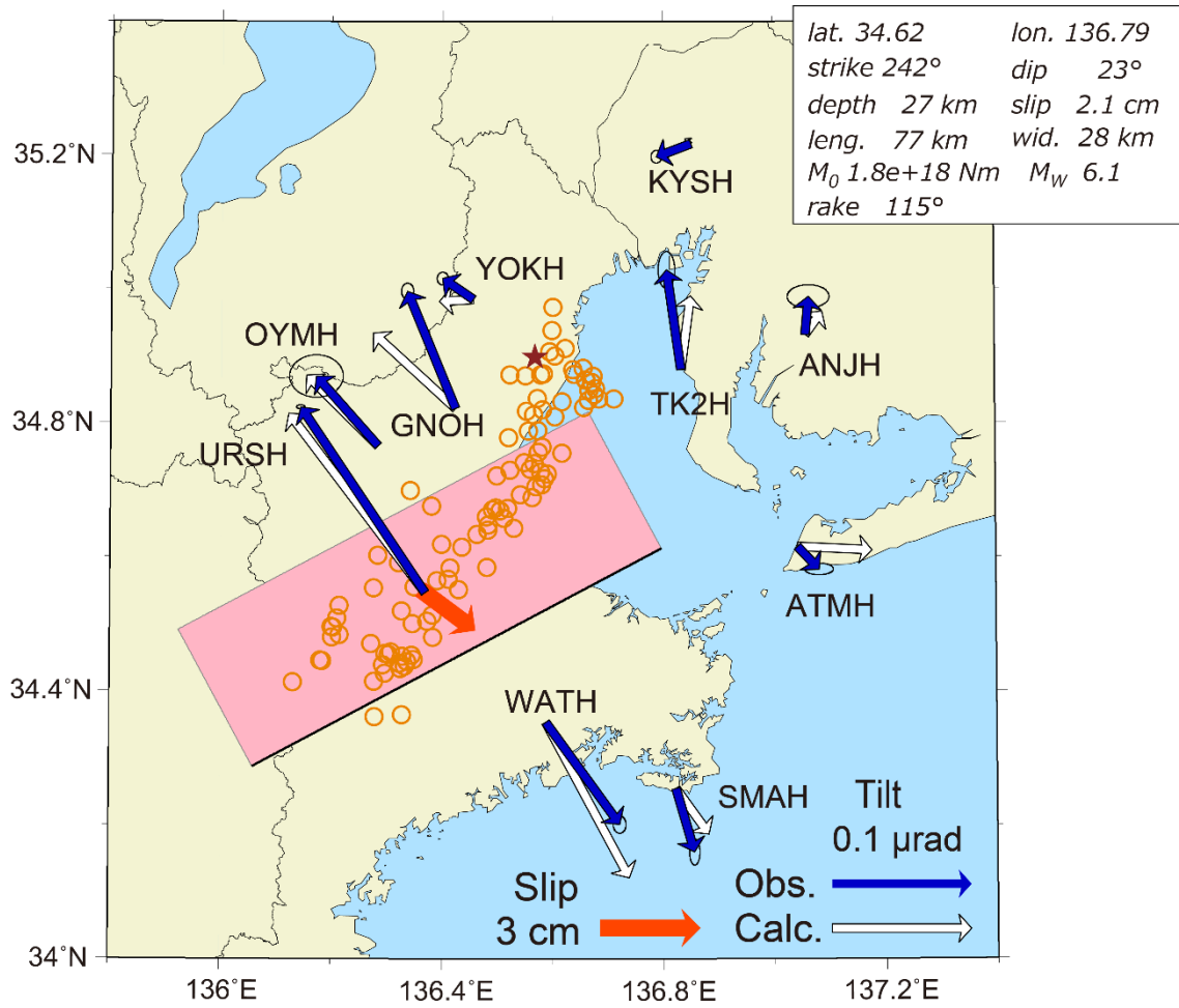
第 5 図 2026 年 2 月紀伊半島北部の短期的 SSE の断層モデル。図の見方は第 3 図と同じ。
