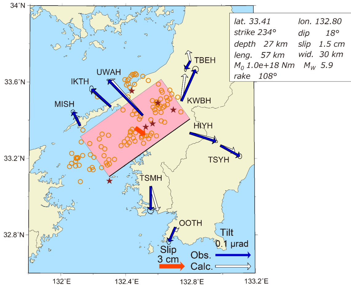
第 3 図 2026 年 1 月四国西部の短期的 SSE の断層モデル。第 2 図の破線で示された期間に観測された傾斜変化ベクトル（青矢印）・このデータから推定された SSE の断層モデル（赤矩形・矢印）・モデルから計算される傾斜変化ベクトル（白抜き矢印）を示す。同じ期間の微動と VLFE の震央を橙円と茶星印で示した。
