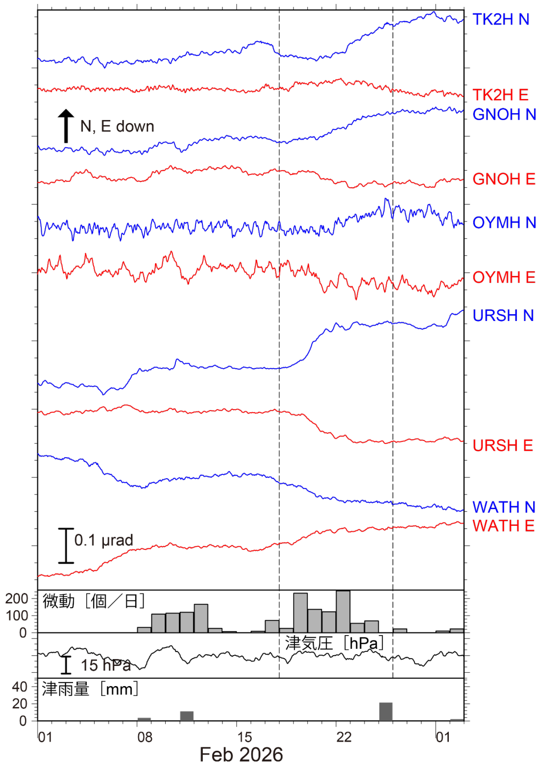
第 4 図 2026 年 2 月 1 日～3 月 2 日までの傾斜時系列。図の見方は第 2 図と同様。観測点位置は第 5 図に示した。2 月 18 日～25 日の傾斜変化量を SSE によるものと仮定した。紀伊半島北部～愛知県での微動活動度・気象庁津観測点での気圧変化および雨量をあわせて表示した。
