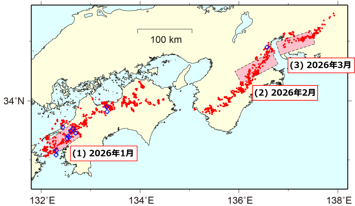
第 1 図 2025 年 11 月 1 日～2026 年 4 月 30 日の期間に検知された短期的 SSE (ピンク矩形). 同期間に発生した深部低周波微動 (赤点) 及び VLFE の震央 (青菱形) を重ねて表示した.
