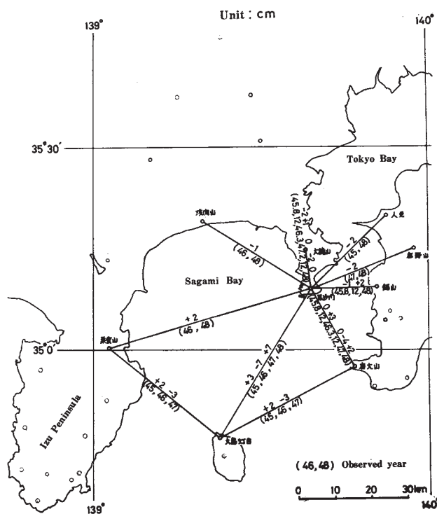
第1図 関東南部辺長測量結果
