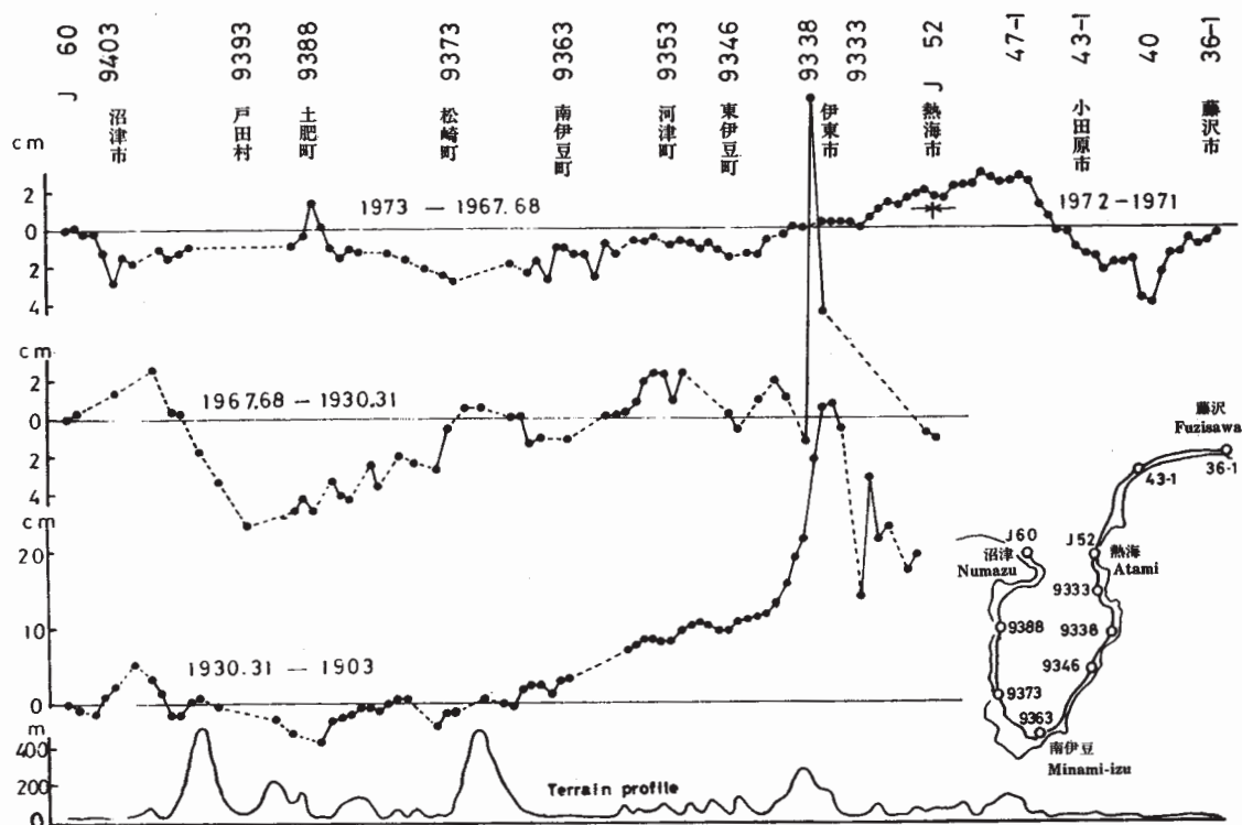
第1図 伊豆地方の上下変動
