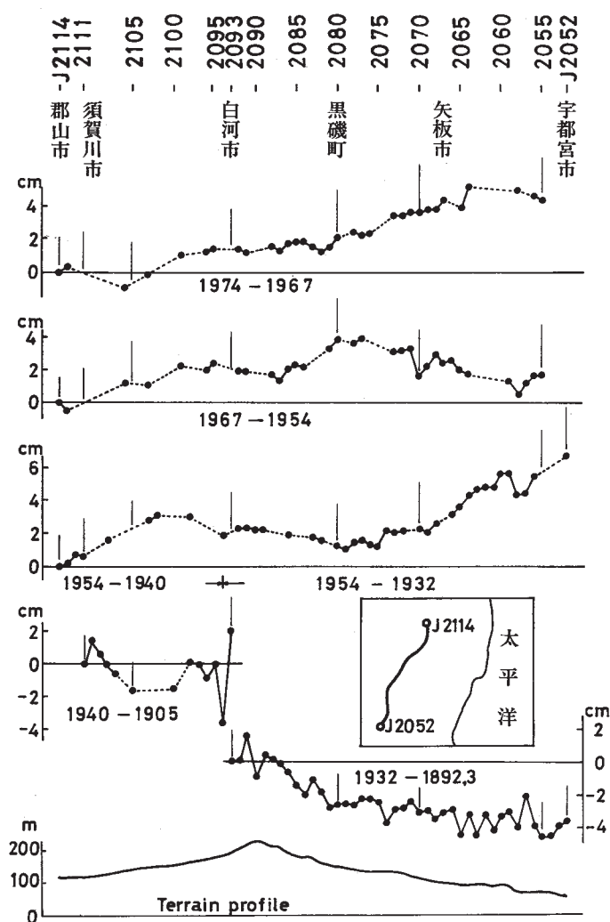
第1図 郡山市～宇都宮市間の上下変動
