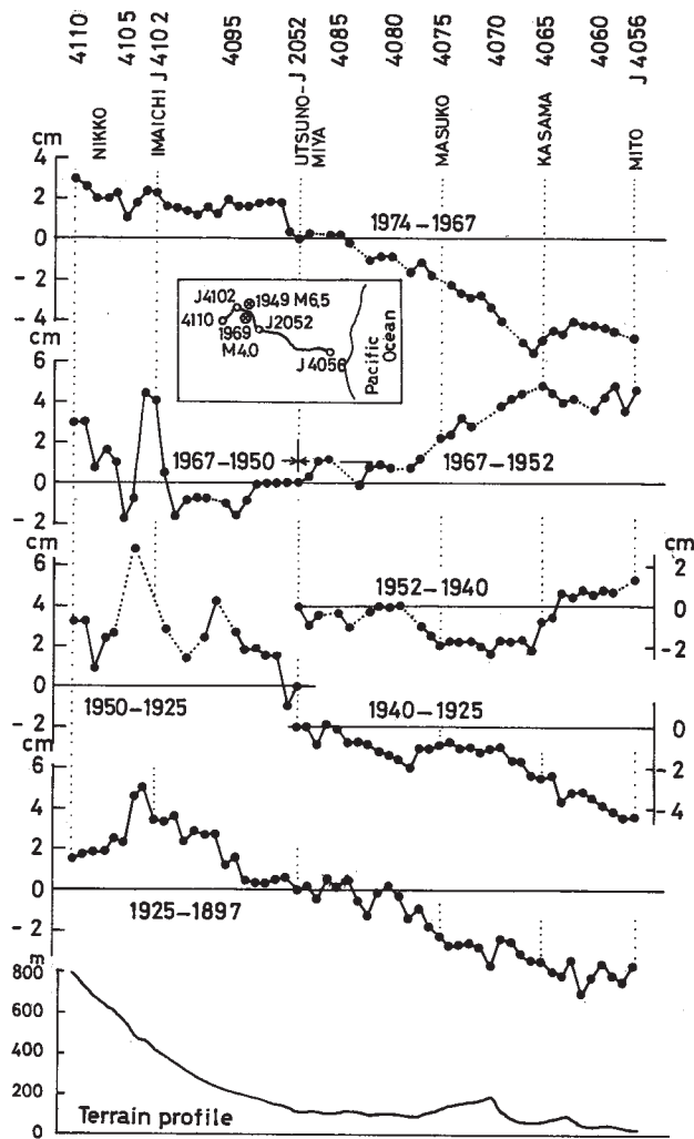
第 1 図 今市市～水戸市間の上下変動
