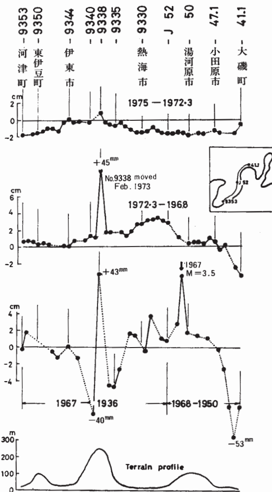
第1図 伊東市 - 大磯市間の上下変動
