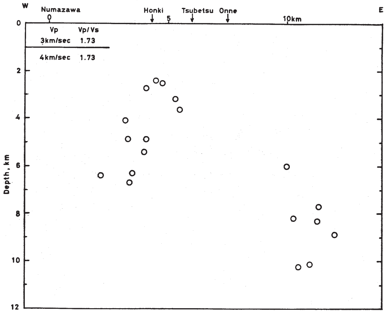
第2図 震源の東西断面図
