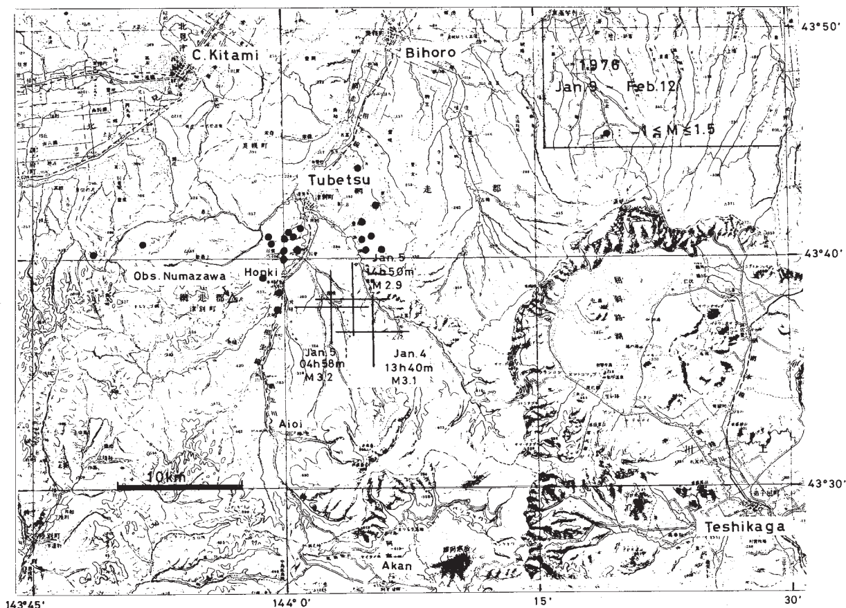
第1図 津別町で発生した地震の震央, + : 有感地震, ● : 極微小地震
