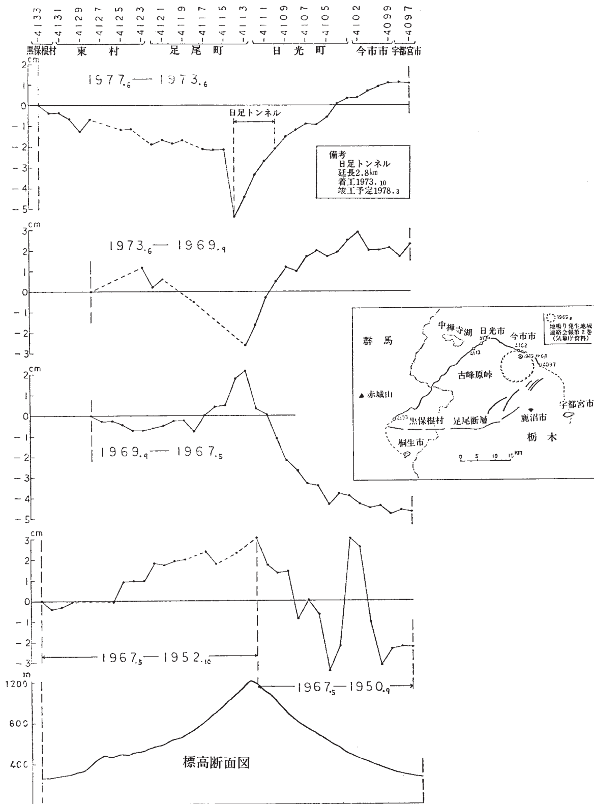
第1図 関東北部の上下変動
