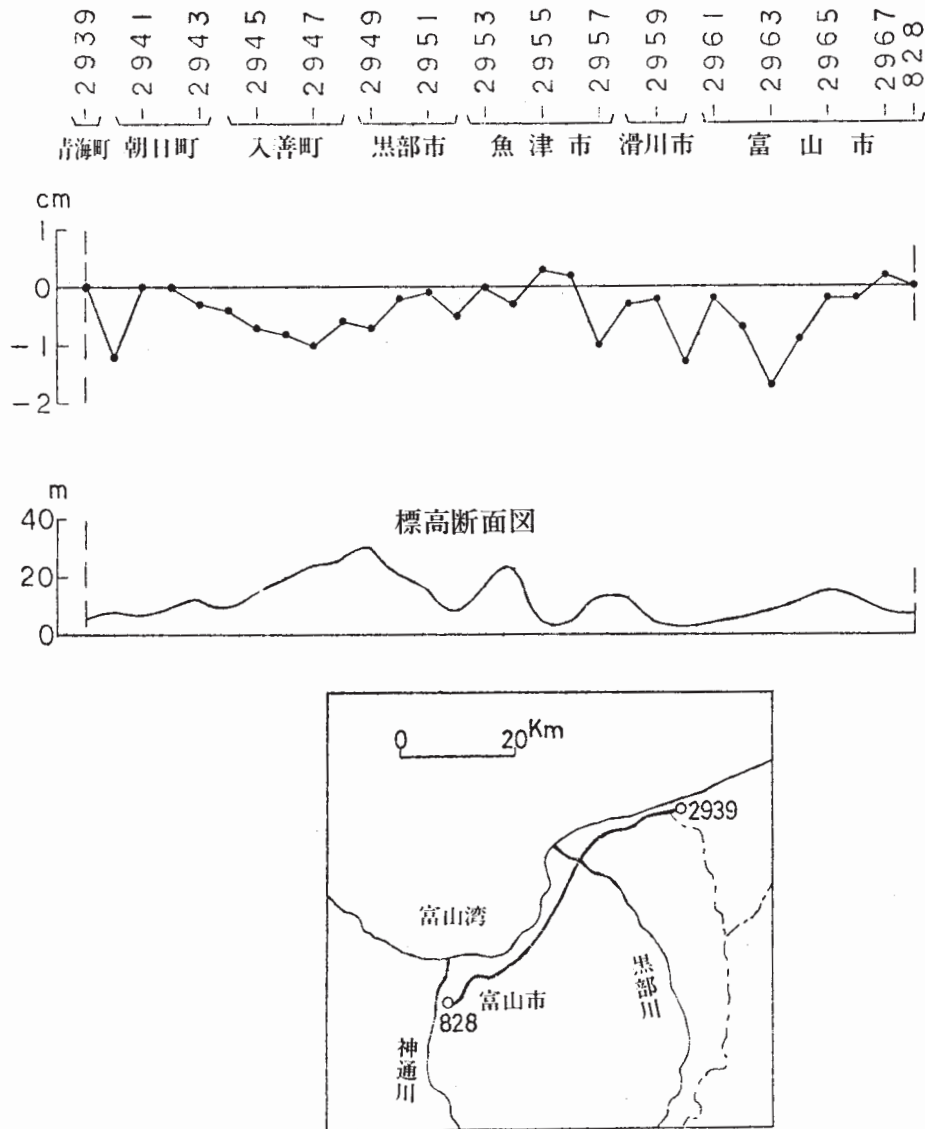
第1図 富山県北東部の上下変動
