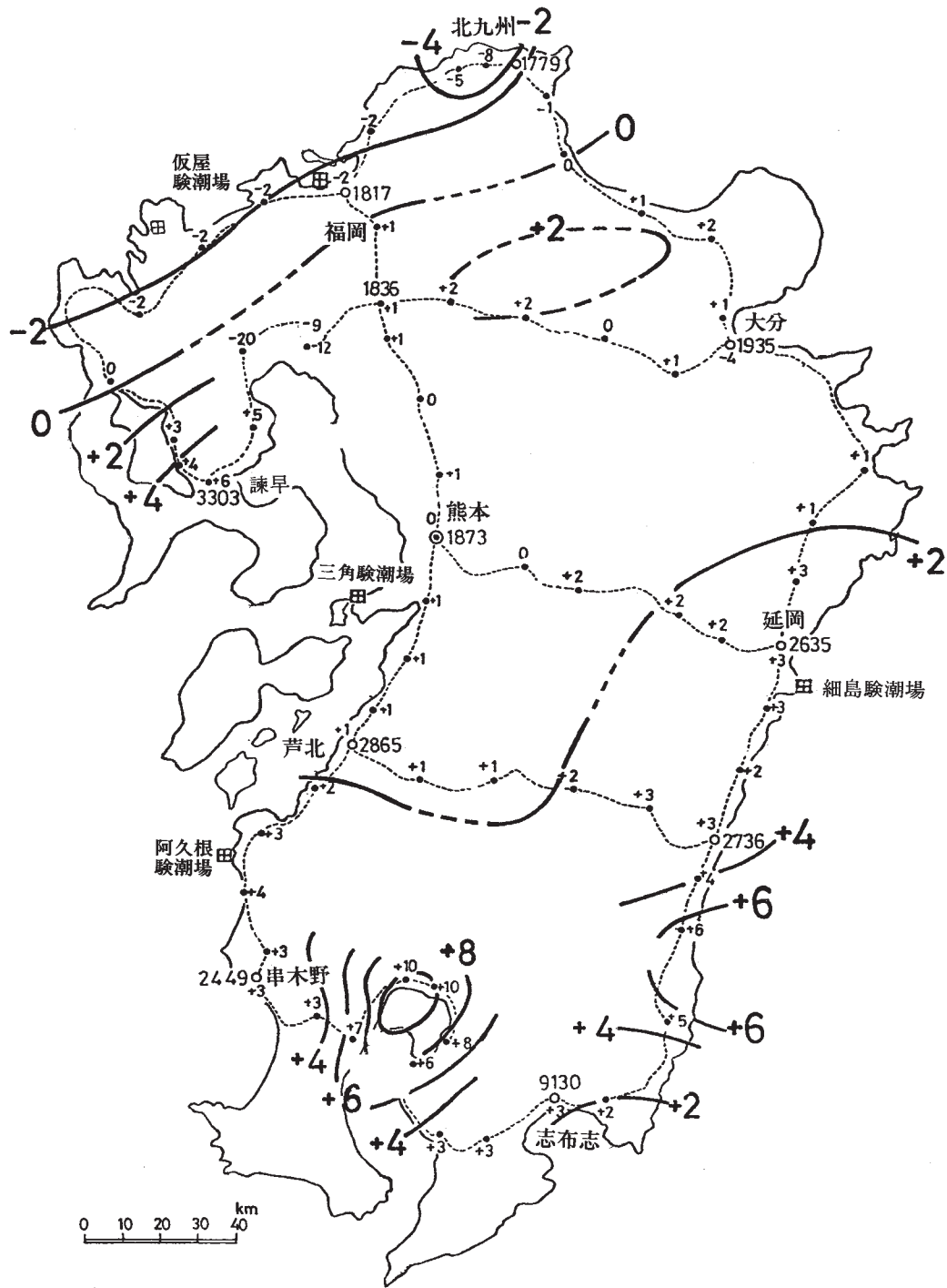
第1図 九州地方の上下変動コンター図
