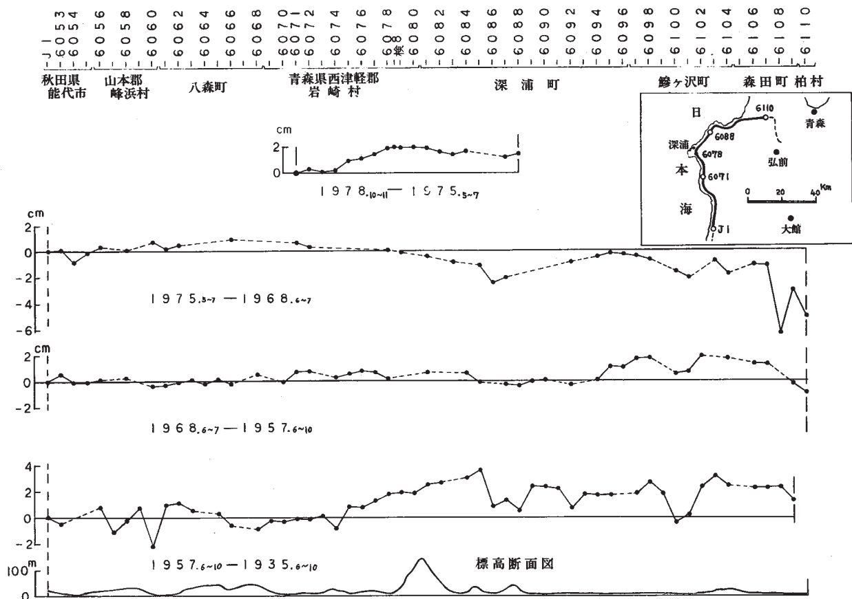
第1図 能代~五所川原間の上下変動
