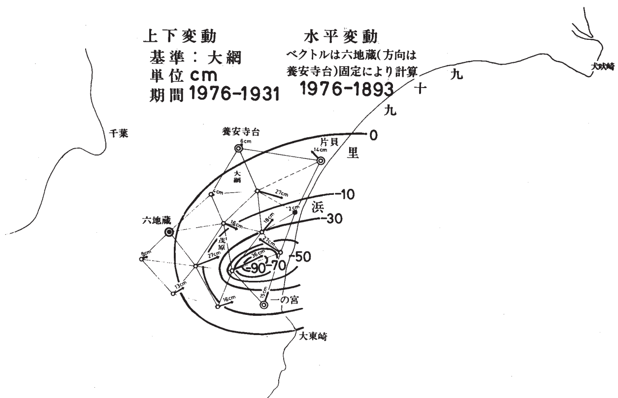
第 2 図 茂原付近の上下及び水平変動
