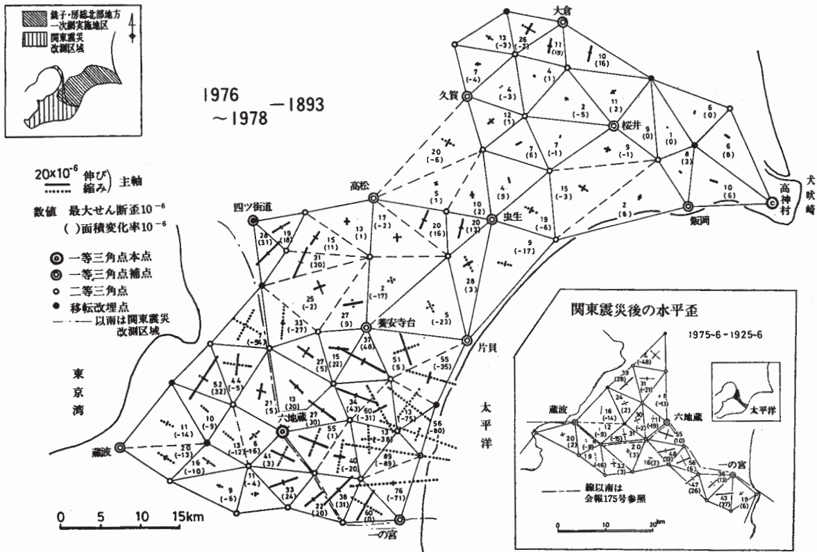
第1図 房総北部地方の水平歪
