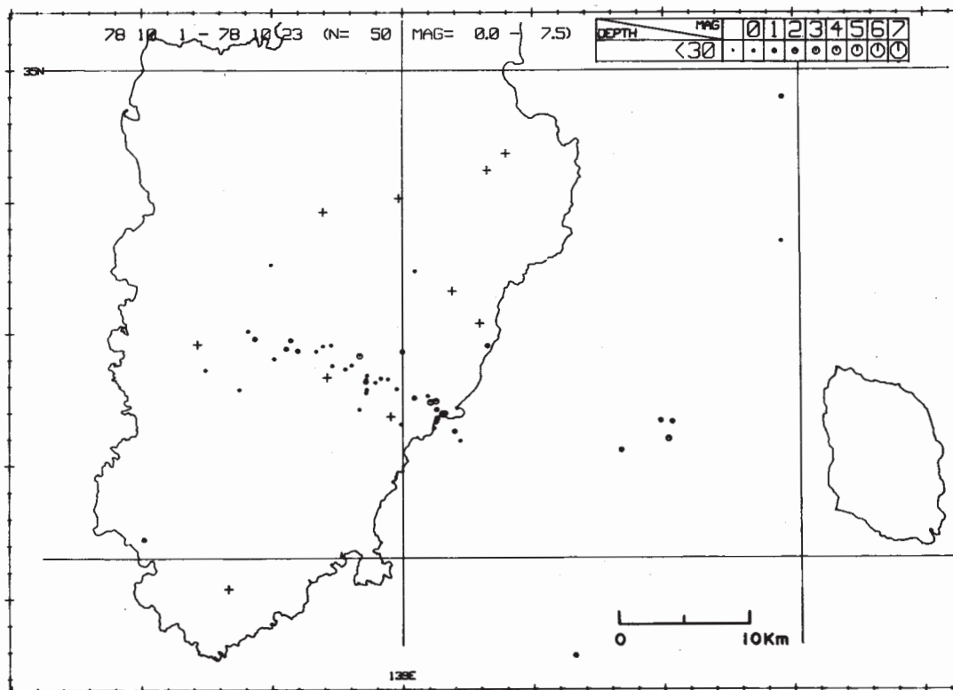
第 6 図 1978 年 10 月の震央分布図
