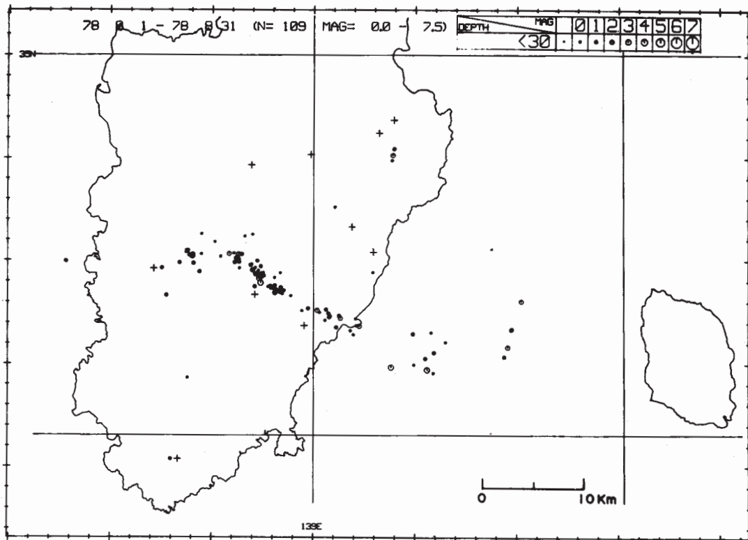
第4図 1978年8月の震央分布図
