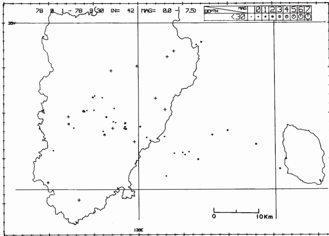
第 5 図 1978 年 9 月の震央分布図
