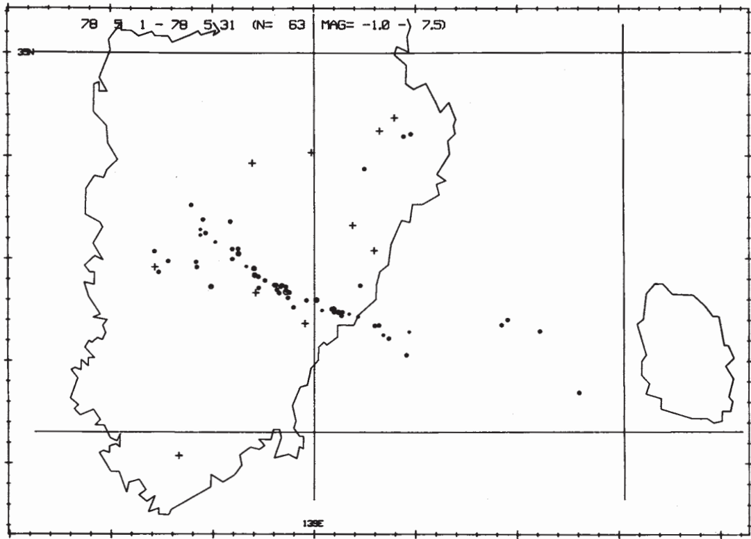
第1図 1978年5月の震央分布図
