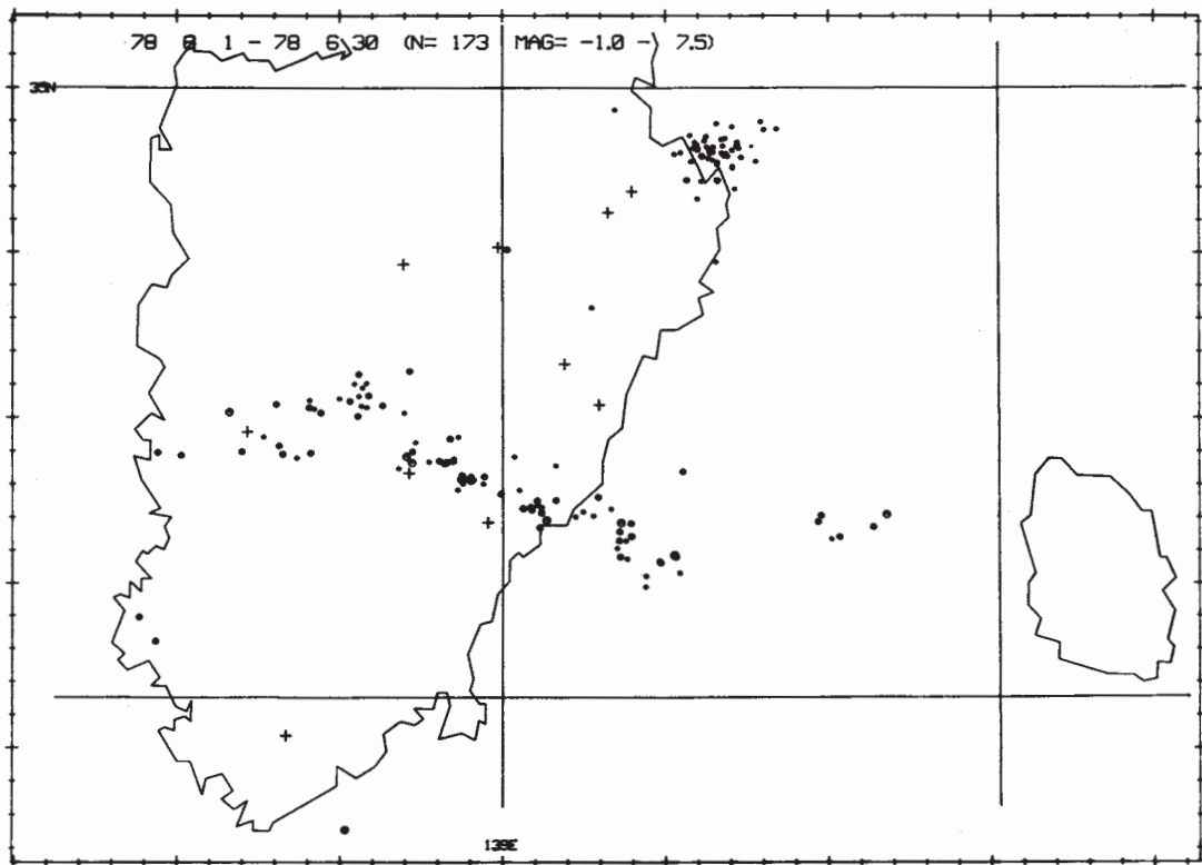
第2図 1978年6月の震央分布図
