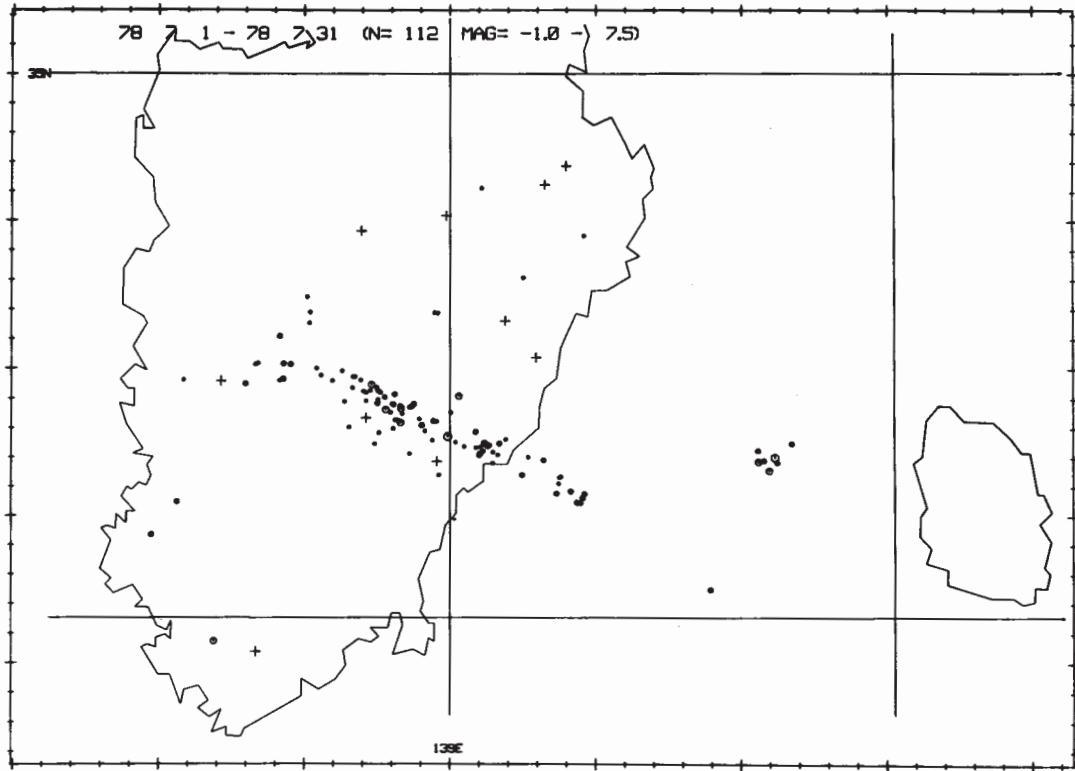
第3図 1978年7月の震央分布図
