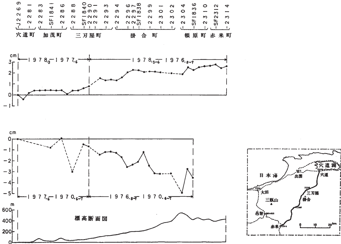
第2図 穴道-赤来間の上下変動
