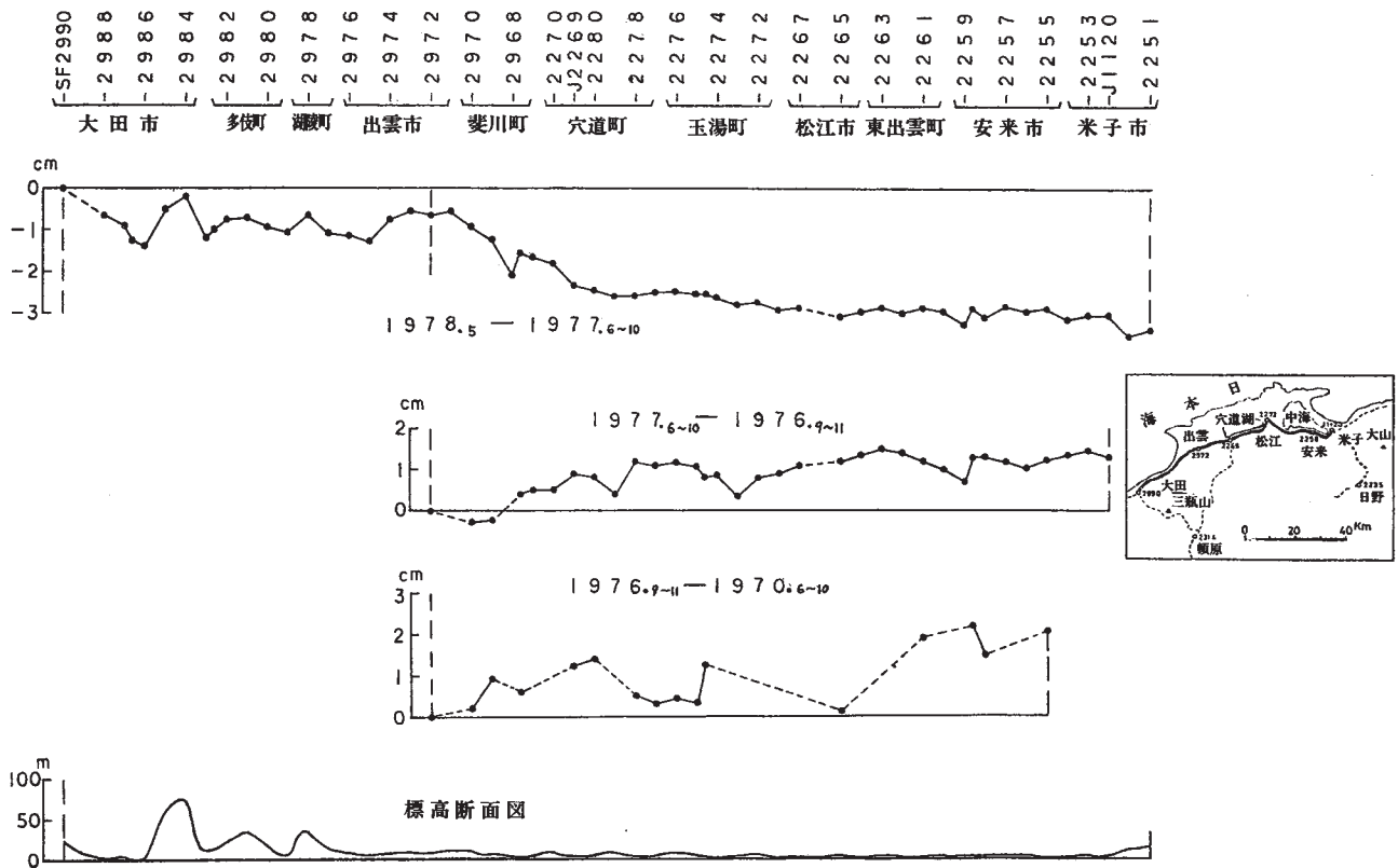
第1図 大田-米子間の上下変動
