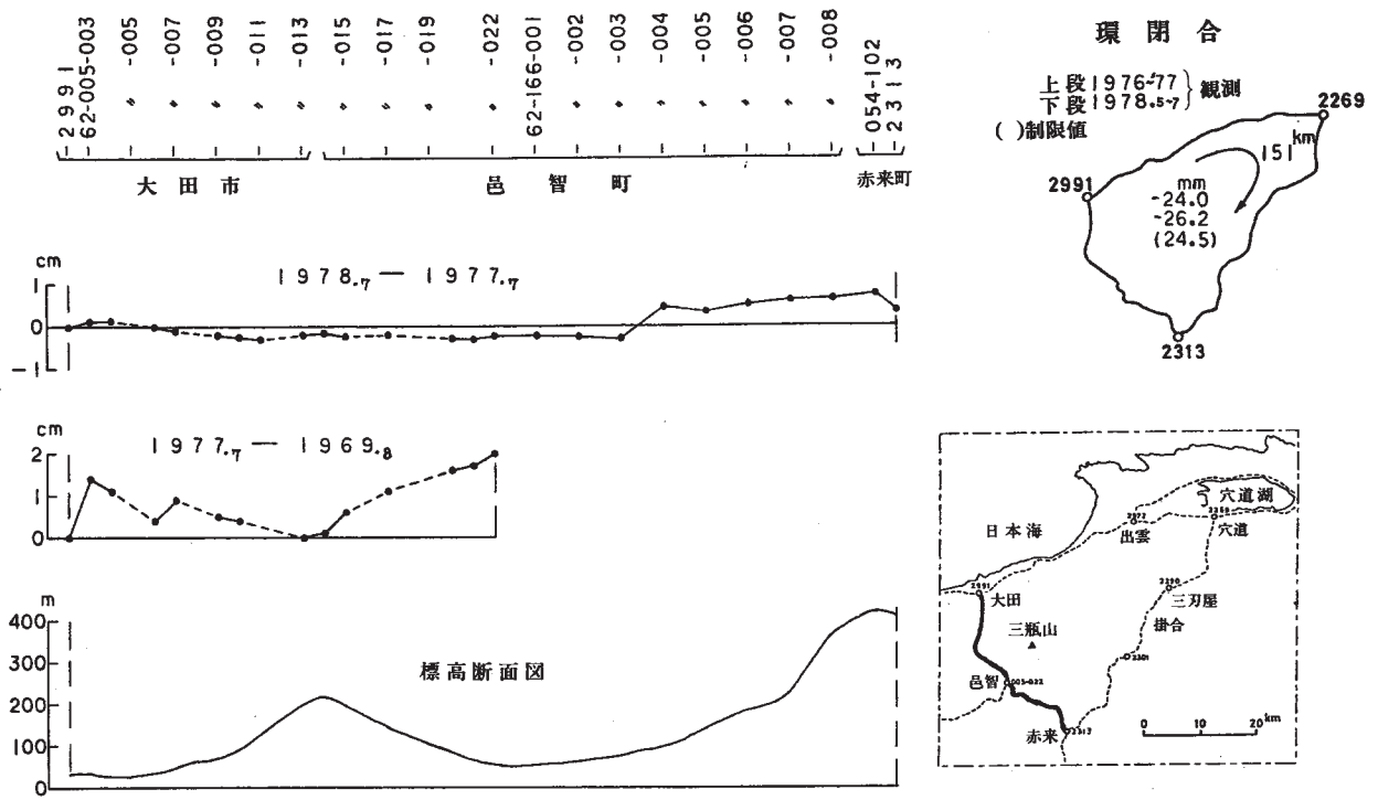
第3図 大田-赤来間の上下変動 Fig. 3 Vertical movements between Ooda and Akagi.
