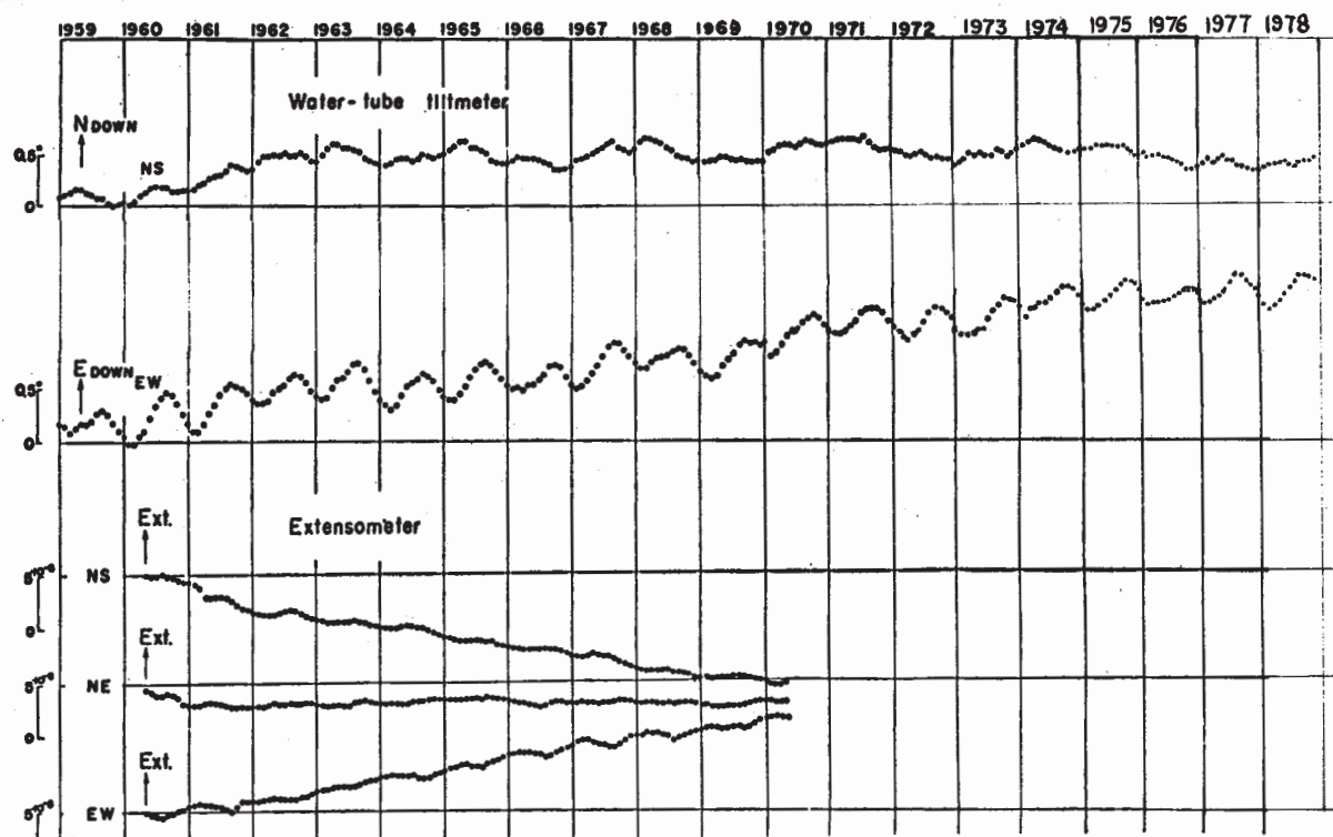
第2図 鋸山における土地傾斜（月平均値）
