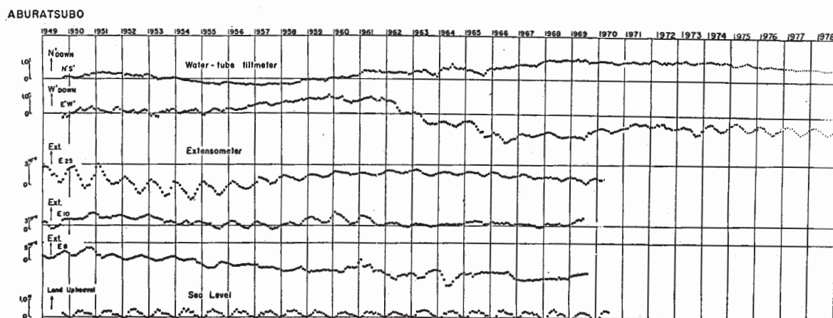
第1図 油壺における土地傾斜（月平均値）
