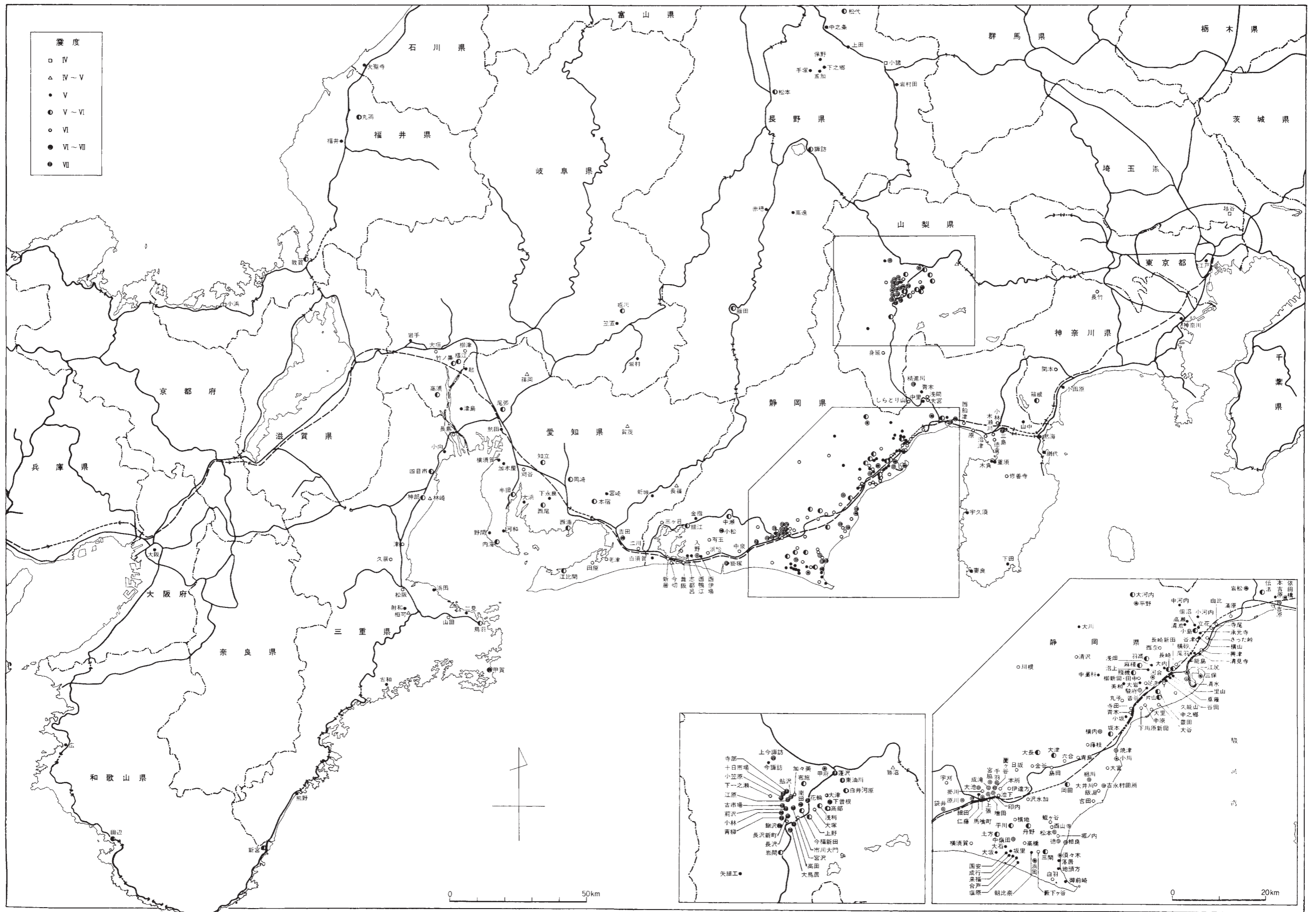
第1図 安政元年11月4日(1854年12月23日)の東海地震の震度分布図
