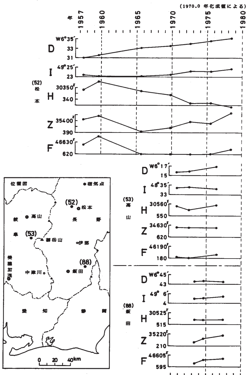
第1図 御岳山周辺の磁気点における経年変化
