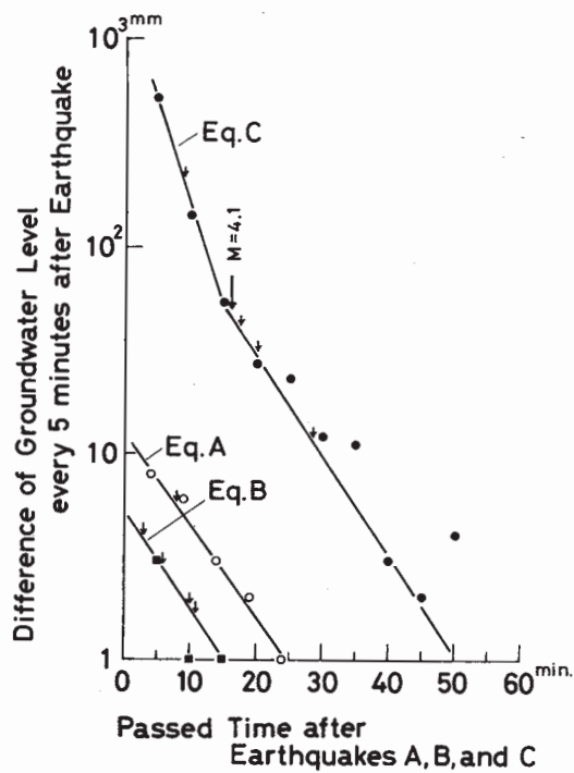
第4図 地震A, B, およびC後の経過時間と5分ごとの水位低下量との関係
