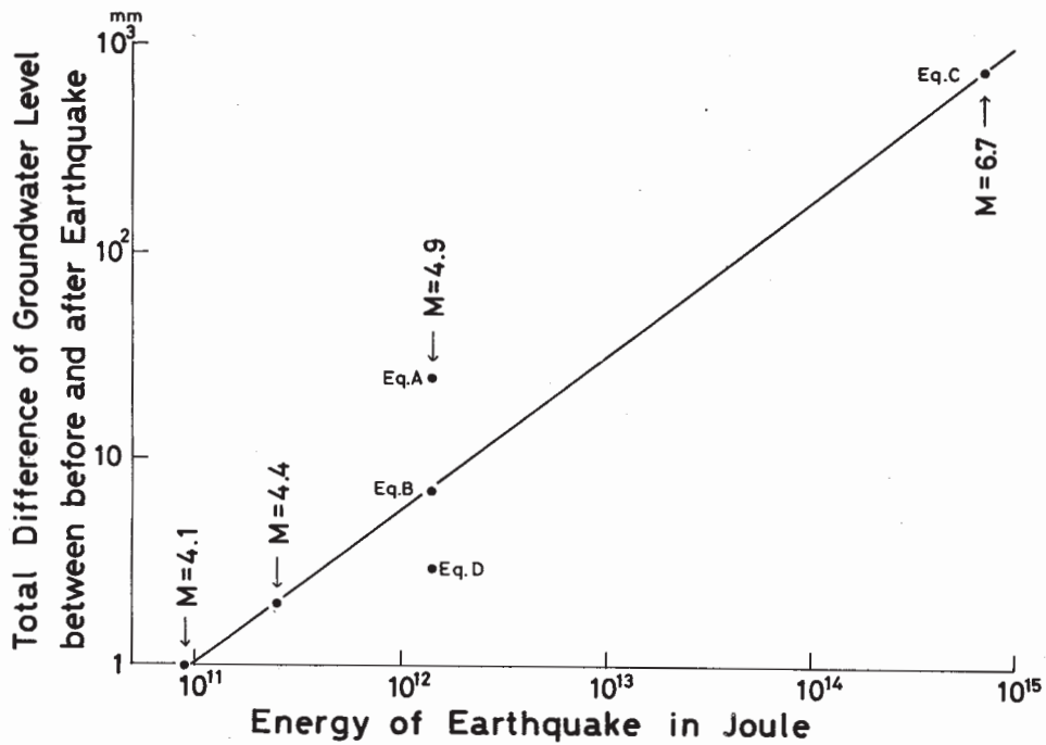
第3図 地震エネルギーと地下水位低下総変動量との関係
