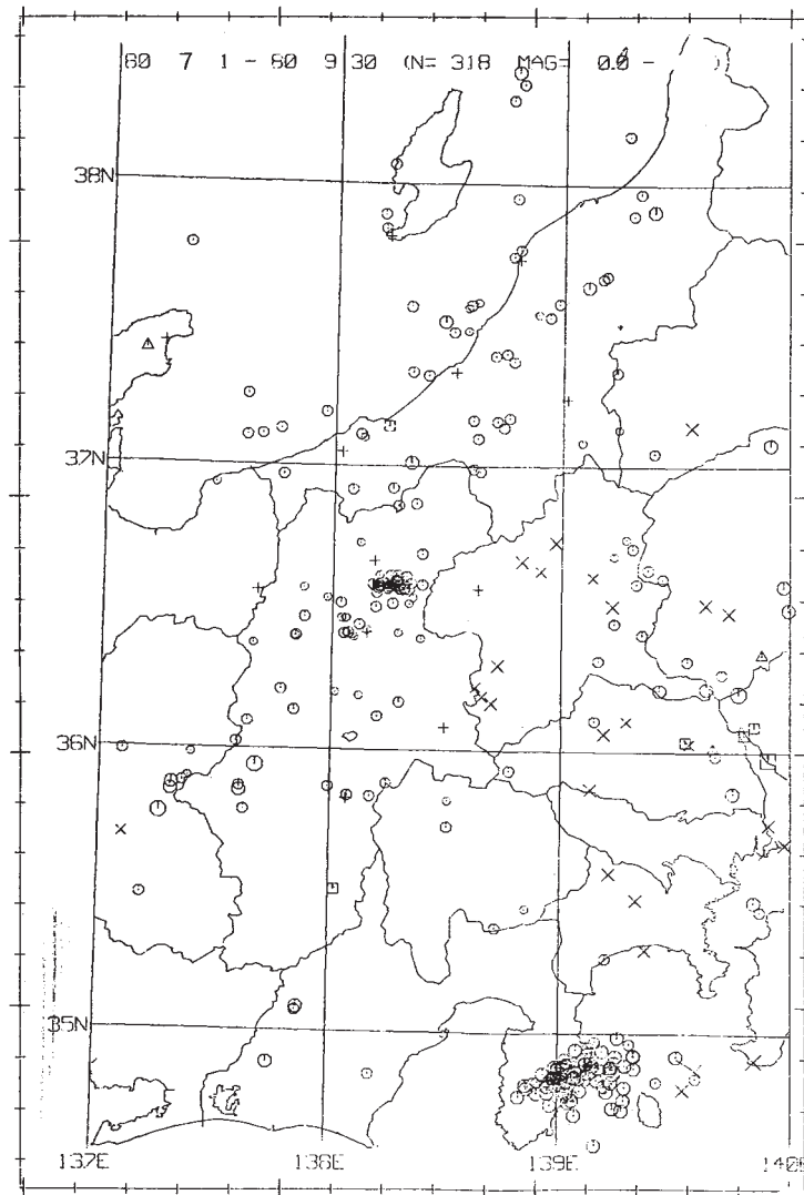
第2図 1980年7月-9月の震央分布図
