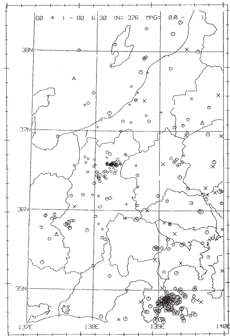
第1図 1980年4月 - 6月の震央分布図
