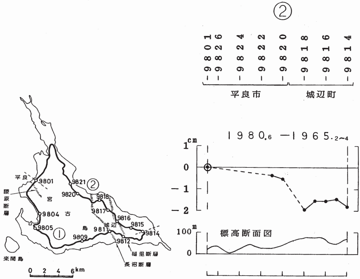
第 2 図 平良 - 城辺間の上下変動グラフ(2)
