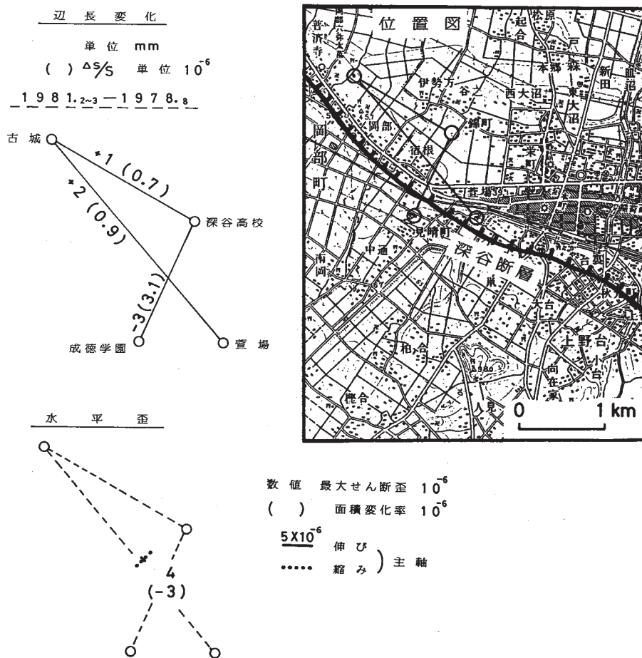
第1図 深谷地区精密変歪測量結果
