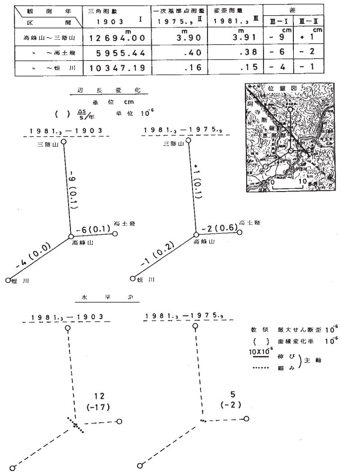
第1図 岐阜放射基線測量結果
