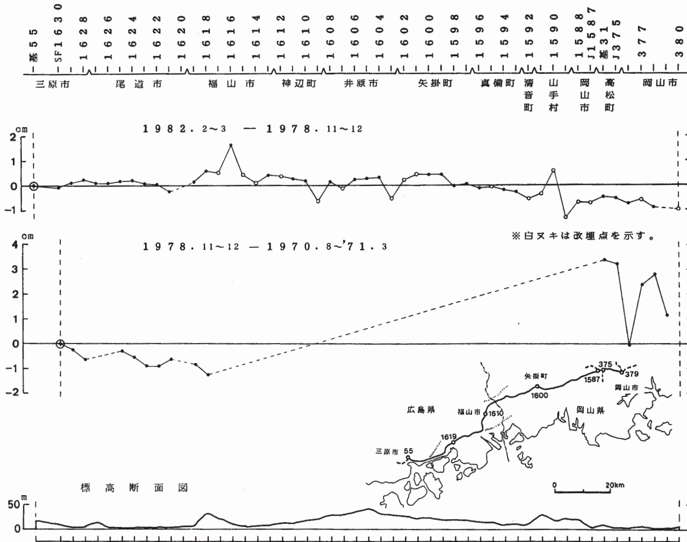
第1図 三原～岡山間の上下変動
