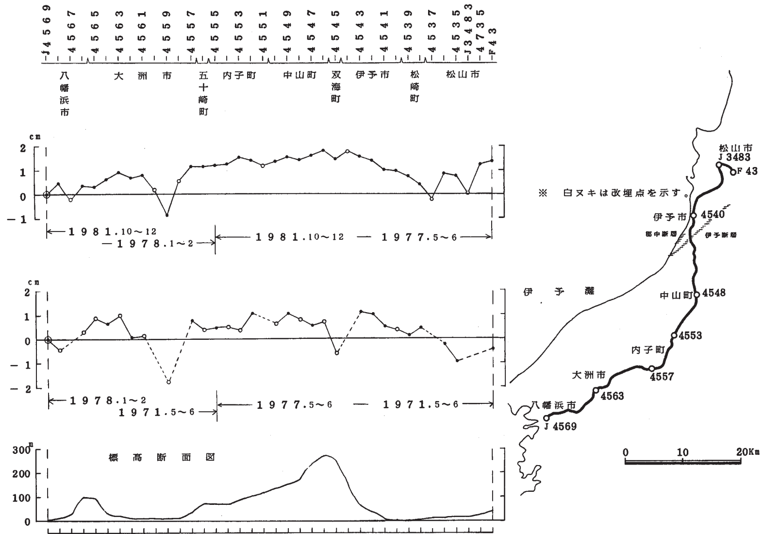
第2図 八幡浜～松山間の上下変動 Fig. 2 Vertical movement between Yahatahama and Matsuyama.
