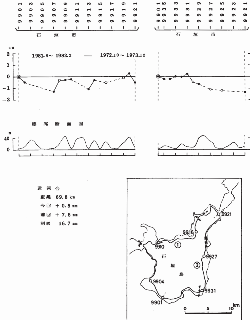
第1図 石垣島の上下変動
