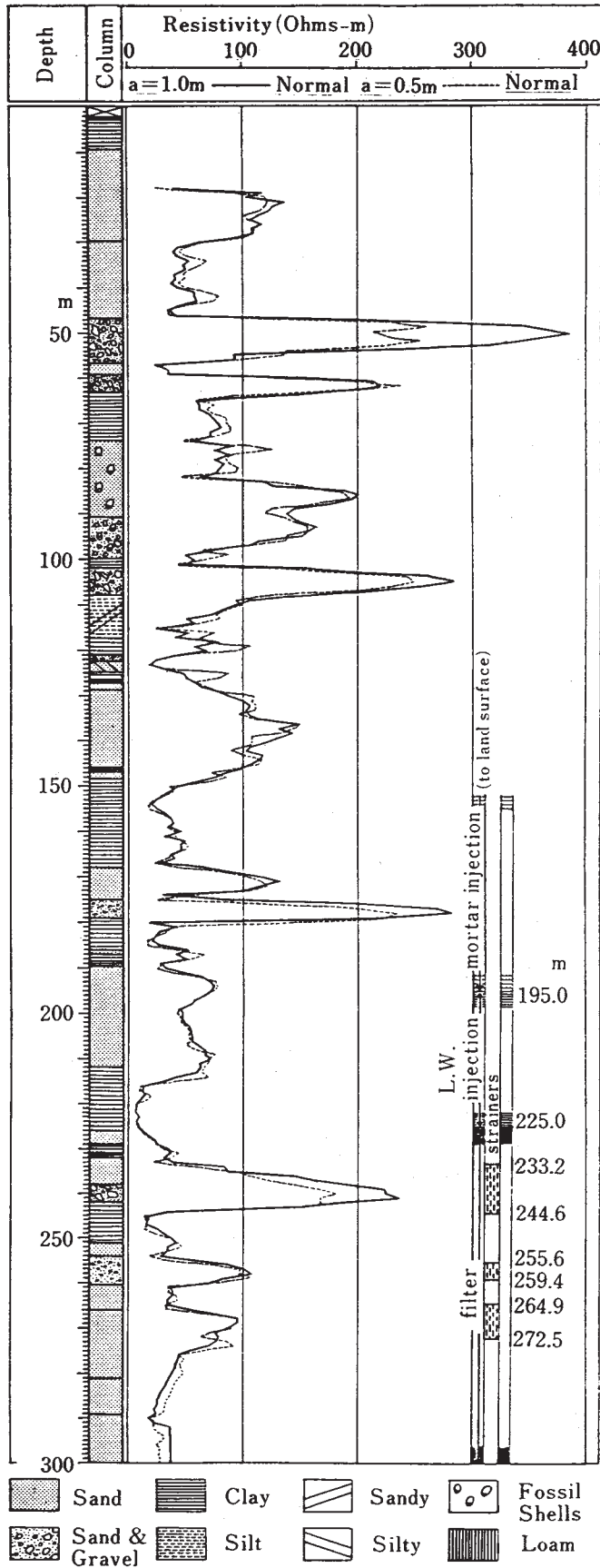
第1図 地質調査所 300m 井の地質柱状図 および電気検層図
