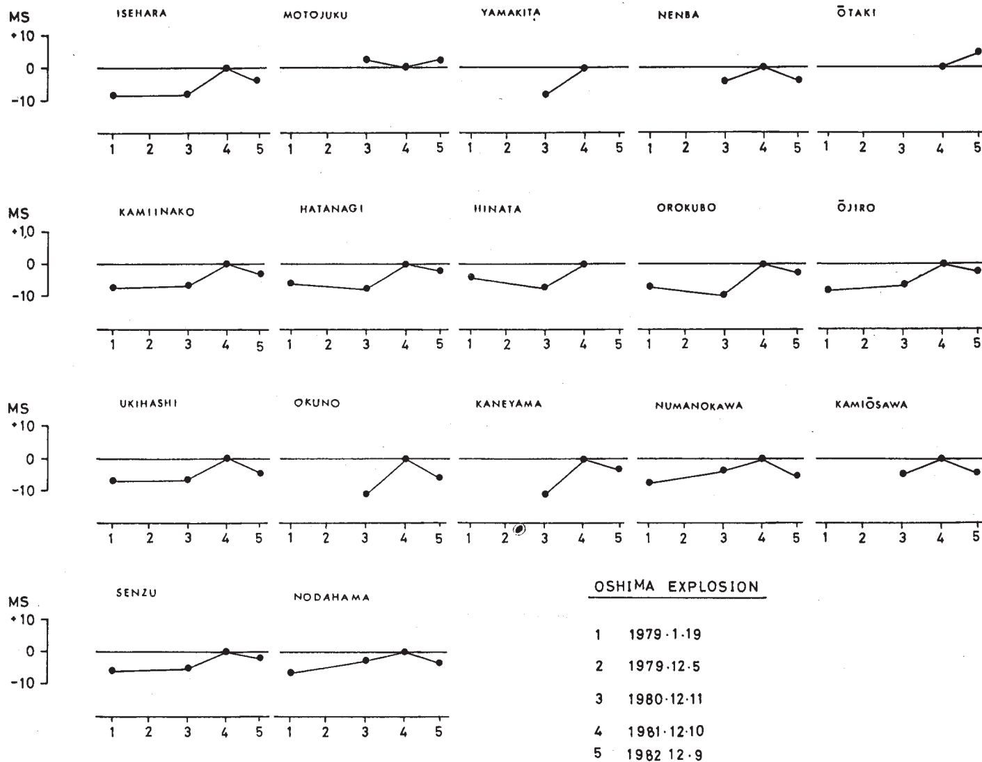
第2図 走時差の経年変化 (1979年1月~1982年12月) Fig. 2 Annual changes in travel time differences (January, 1979 - December, 1982).
