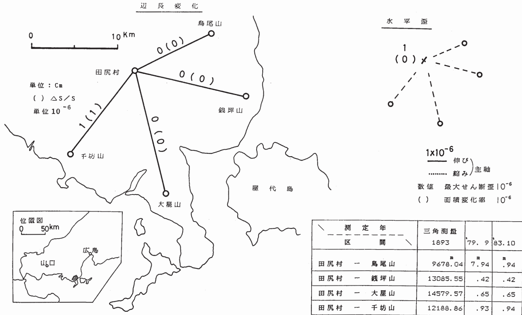
第1図 柳井地方精密変歪測量結果
