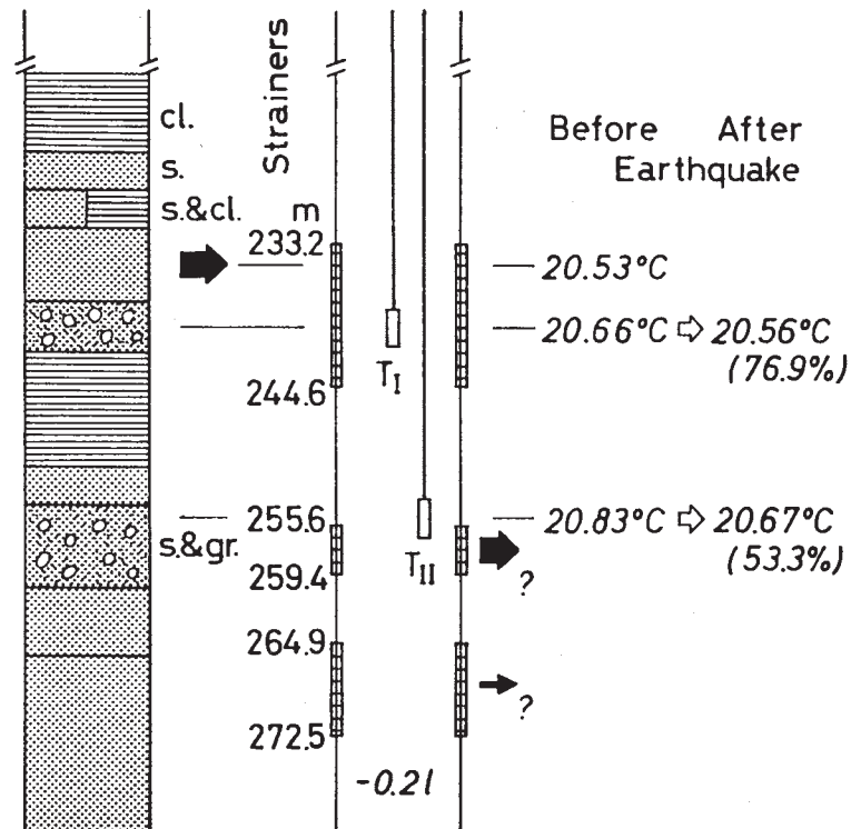
第3図 300 m井の地質柱状図，ストレーナの位置，および地震前後の水温変化と推定される地下水の流動経路（T I ：白金抵抗温度計，T II ：サーミスタ温度計）
