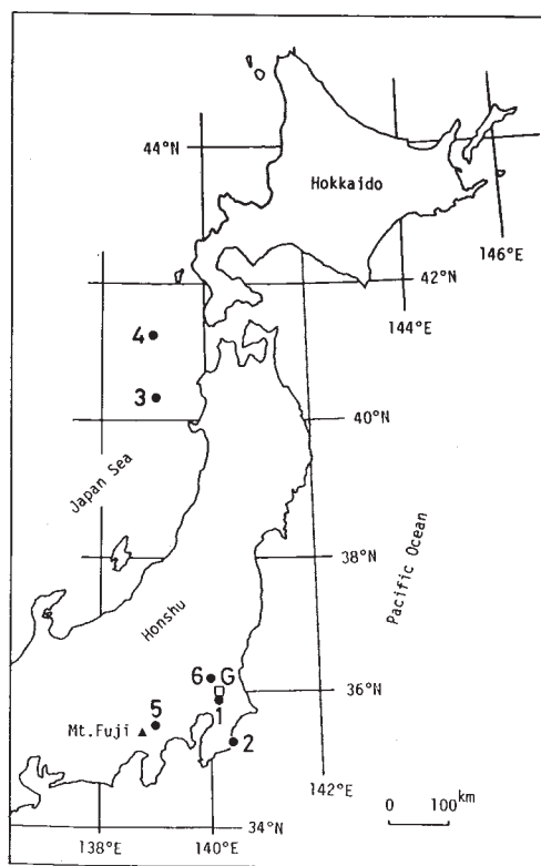
第 1 図 震央分布および観測井 ( G ) 位置図
