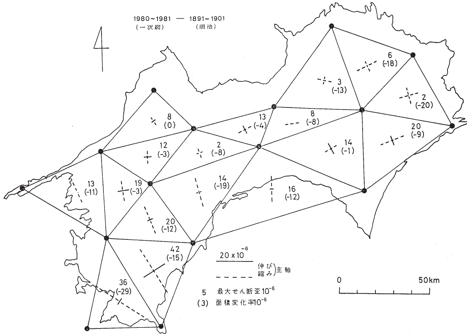
第2図 四国地方の水平歪 (2), 1980 ~ 1981 (一次網) - 1891 ~ 1901 (明治)
