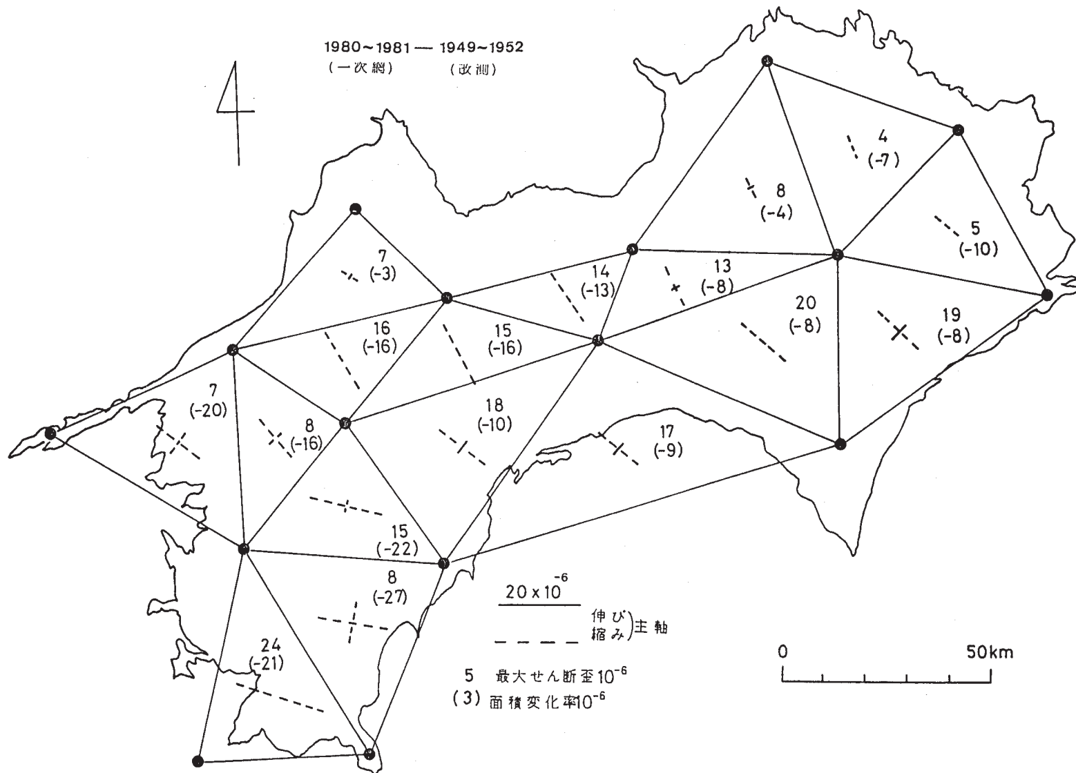
第1図 四国地方の水平歪(1), 1980~1981(一次網) - 1949~1952(改測)
