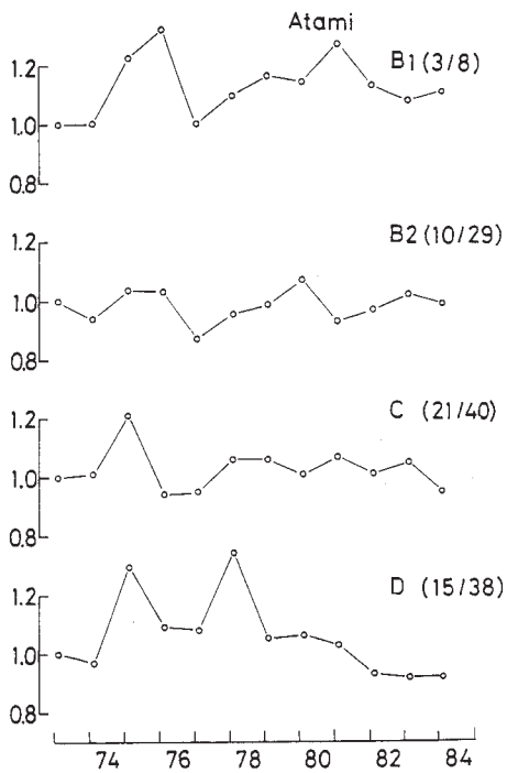
第6図 熱海温泉の各区域別における湧出熱量の変化 Fig. 6 Secular variation of heat output in each zone at Atami spa.
