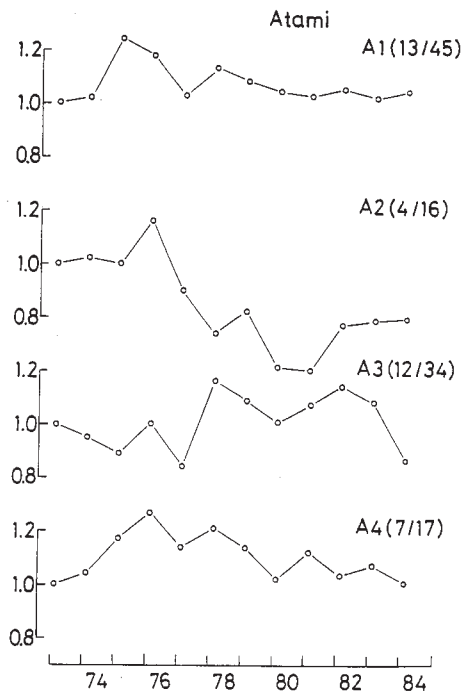
第5図 熱海温泉の各区域別における湧出熱量の変化 Fig. 5 Secular variation of heat output in each zone at Atami spa.
