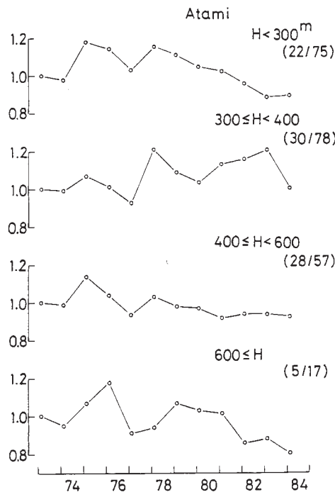
第2図 熱海温泉における深さ別源泉の湧出熱量変化。1973年から1974年の間安定していた源泉についての計算で、これらの源泉数と総源泉数との比を括弧内以示す。1973年の湧出熱量を基準
