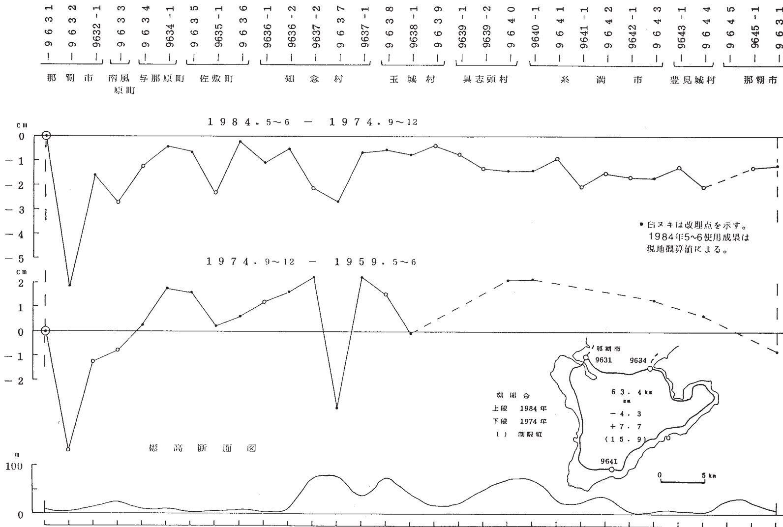
第1図 沖縄南部の上下変動
