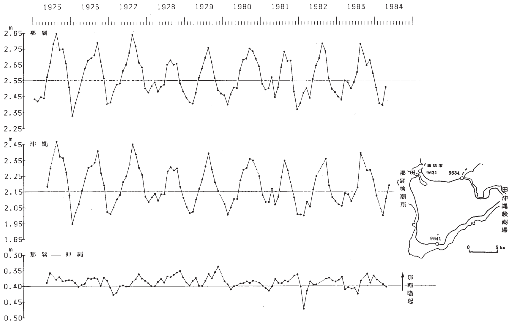
第2図 那覇・沖縄験潮場の月平均潮位及び潮位差。
