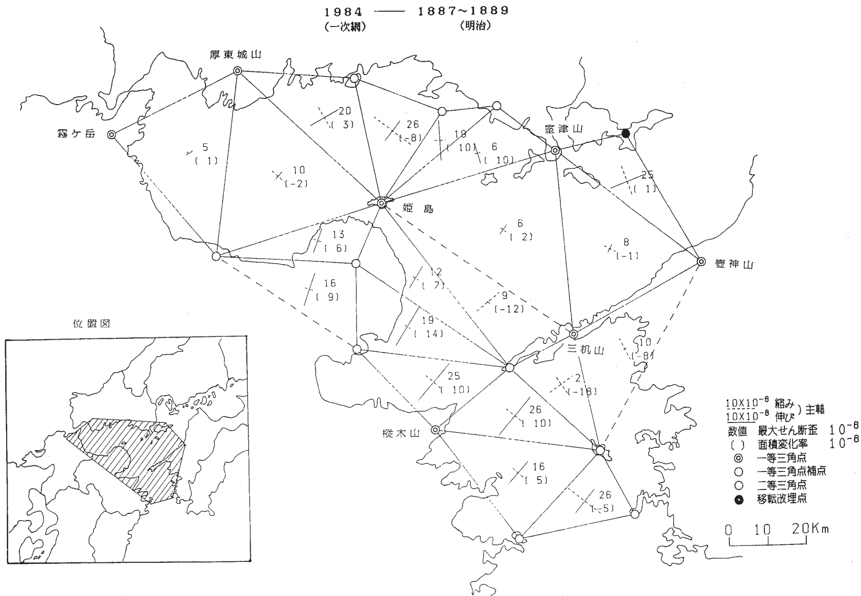
第1図 瀬戸内海西部地域の水平歪 Fig. 1 Horizontal strains in the western Seto Inland Sea region.
