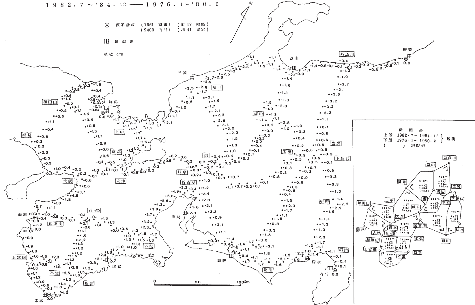
第1図 中部・近畿地方の上下変動
