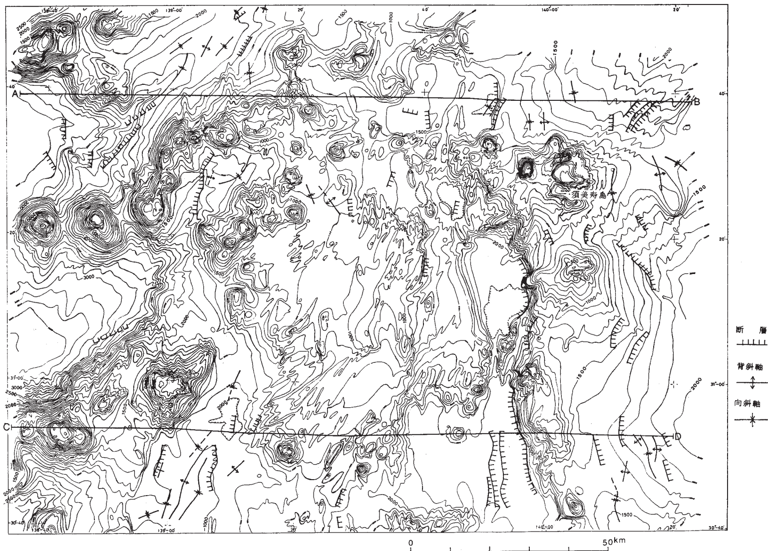
第2図 須美寿島付近の海底地形・地質構造 等深線は100m 間隔
