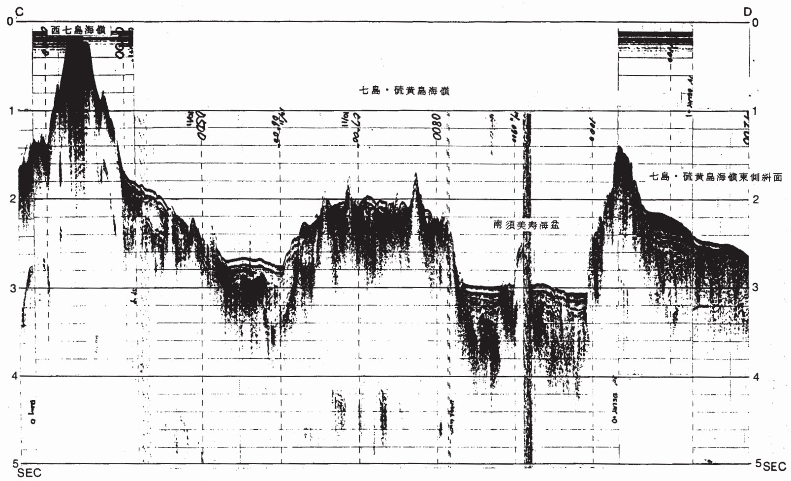
第4図 音波探査記録例 測線位置は第2図に示す Fig. 4 Single channel seismic section. Location is shown in Fig. 2.
