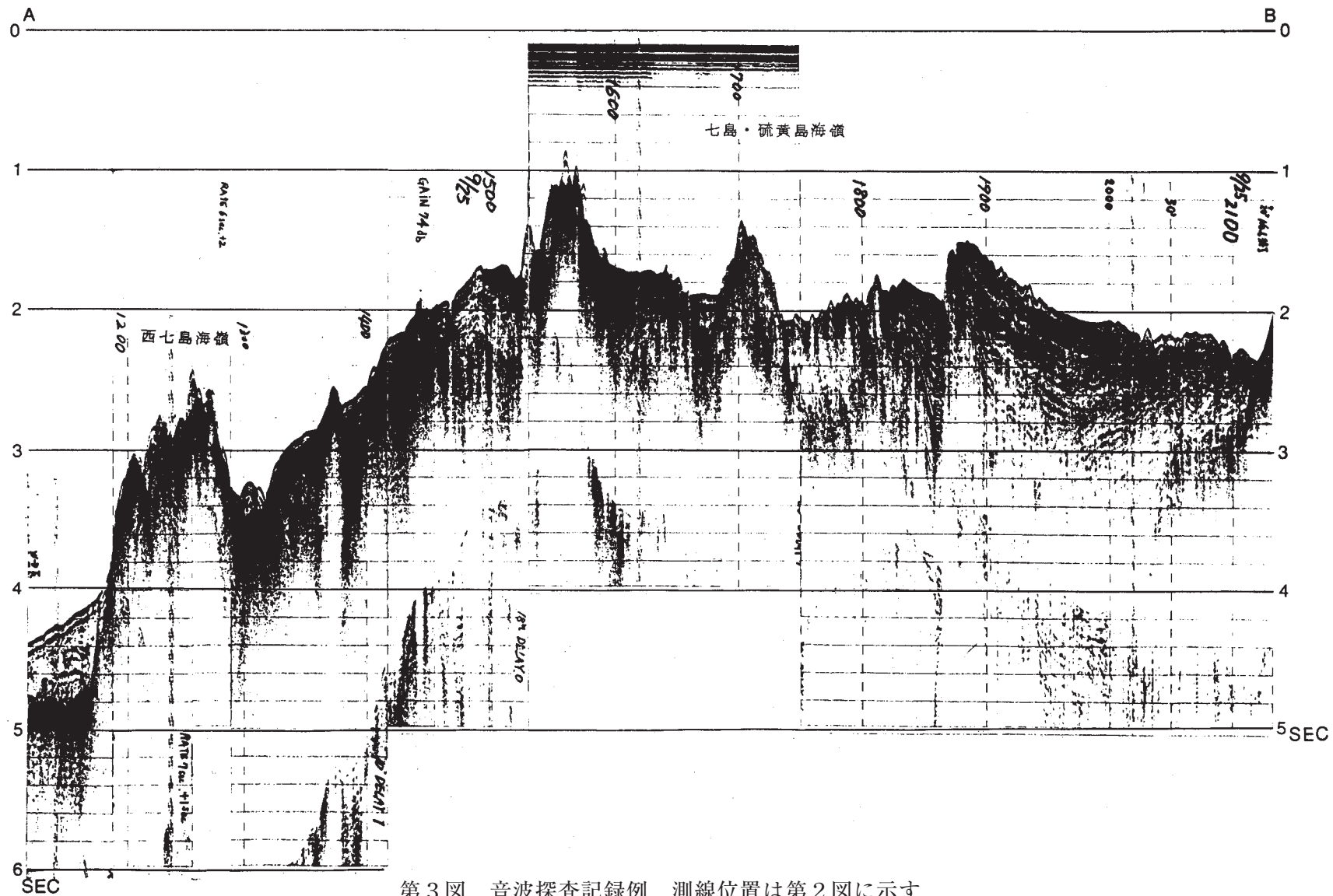
第3図 音波探査記録例 測線位置は第2図に示す Fig. 3 Single channel seismic section. Location is shown in Fig. 2.
