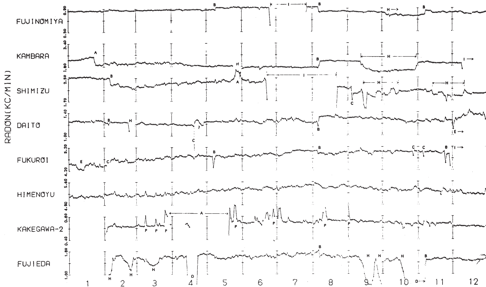
第2図 各観測地点地下水中のラドン計数率変化 (日平均, 1985年1月-12月)
