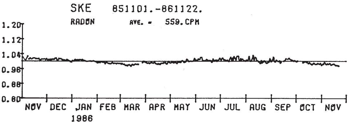
第2図 HTG (函南), RHB (中伊豆), SKE (中伊豆) における地下水中のラドン濃度の変化 (1985年11月~1986年11月)
