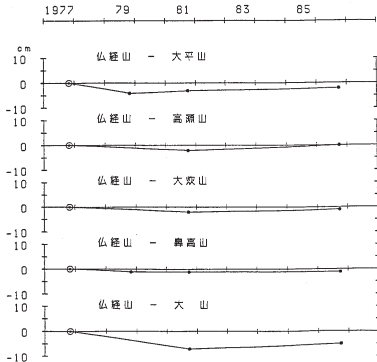
第1図 出雲地区精密変歪測量結果
