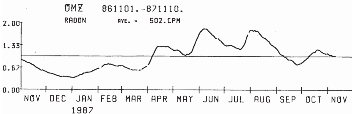
第2図 RYO (竜洋), YSD (吉田), OMZ (御前崎) における地下水中のラ ドン濃度の変化 (1986年11月 - 1987年11月)
