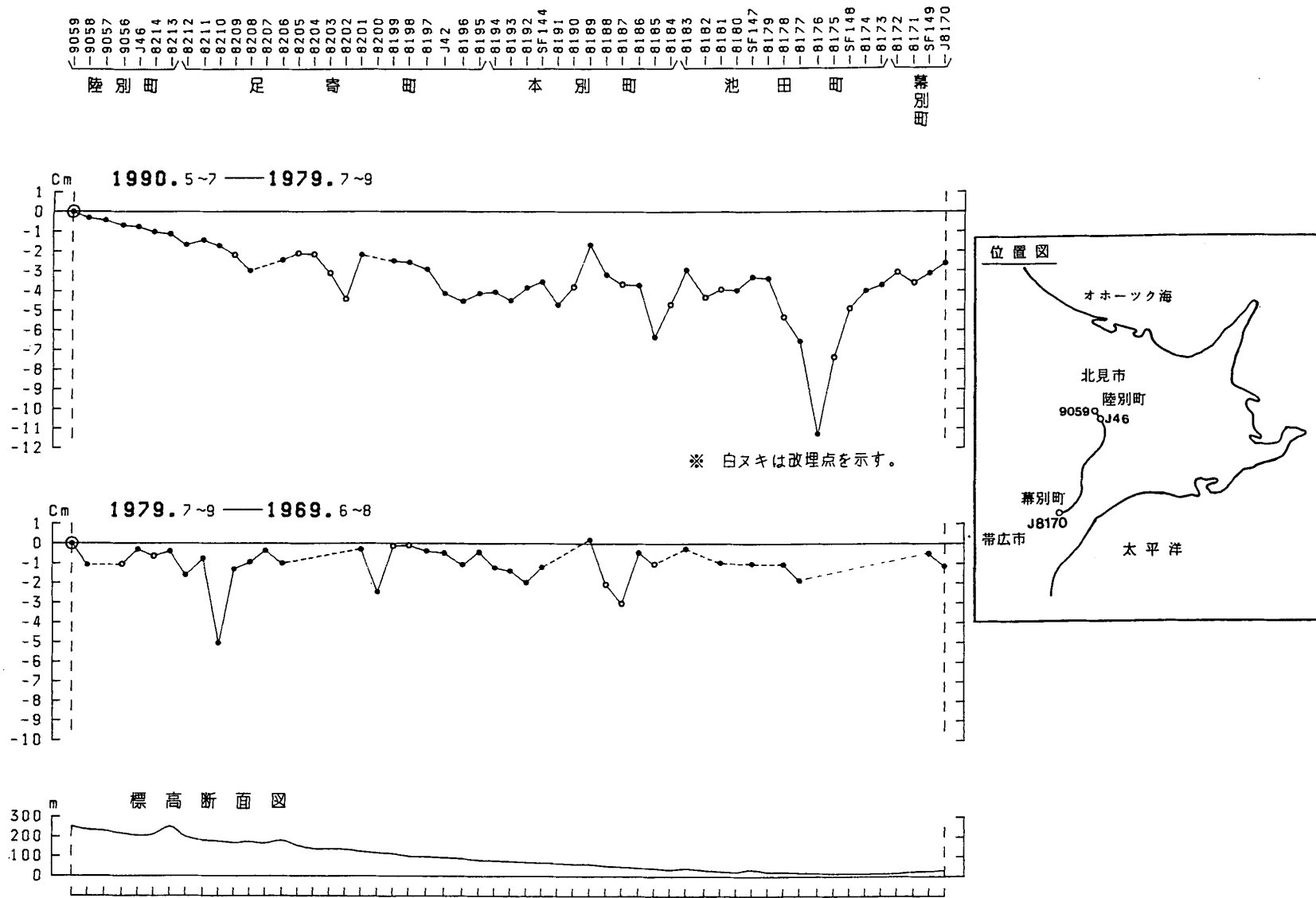
第1図 陸別—幕別間の上下変動
